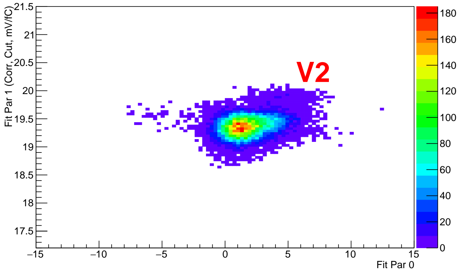
Fit Par 1 (Corr, Cut, mV/fC) vs Par 0
