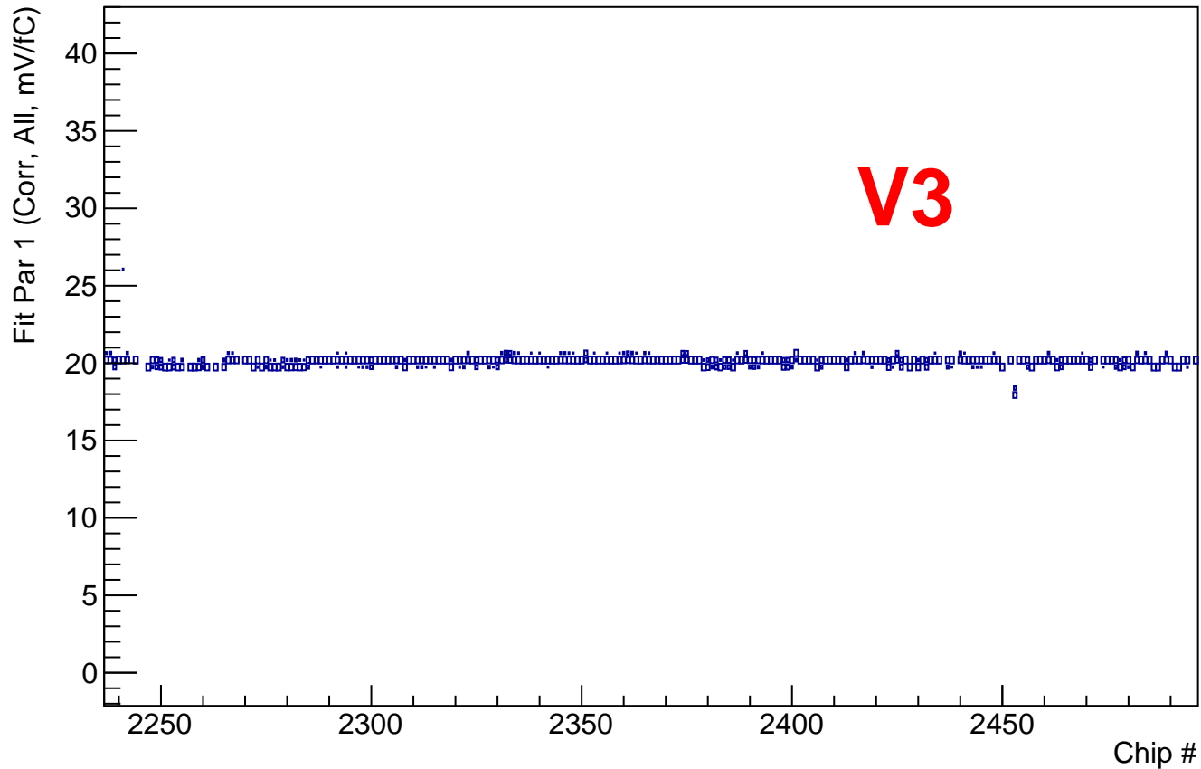
Fit Par 1 (Corr, All, mV/fC) vs Chip #
