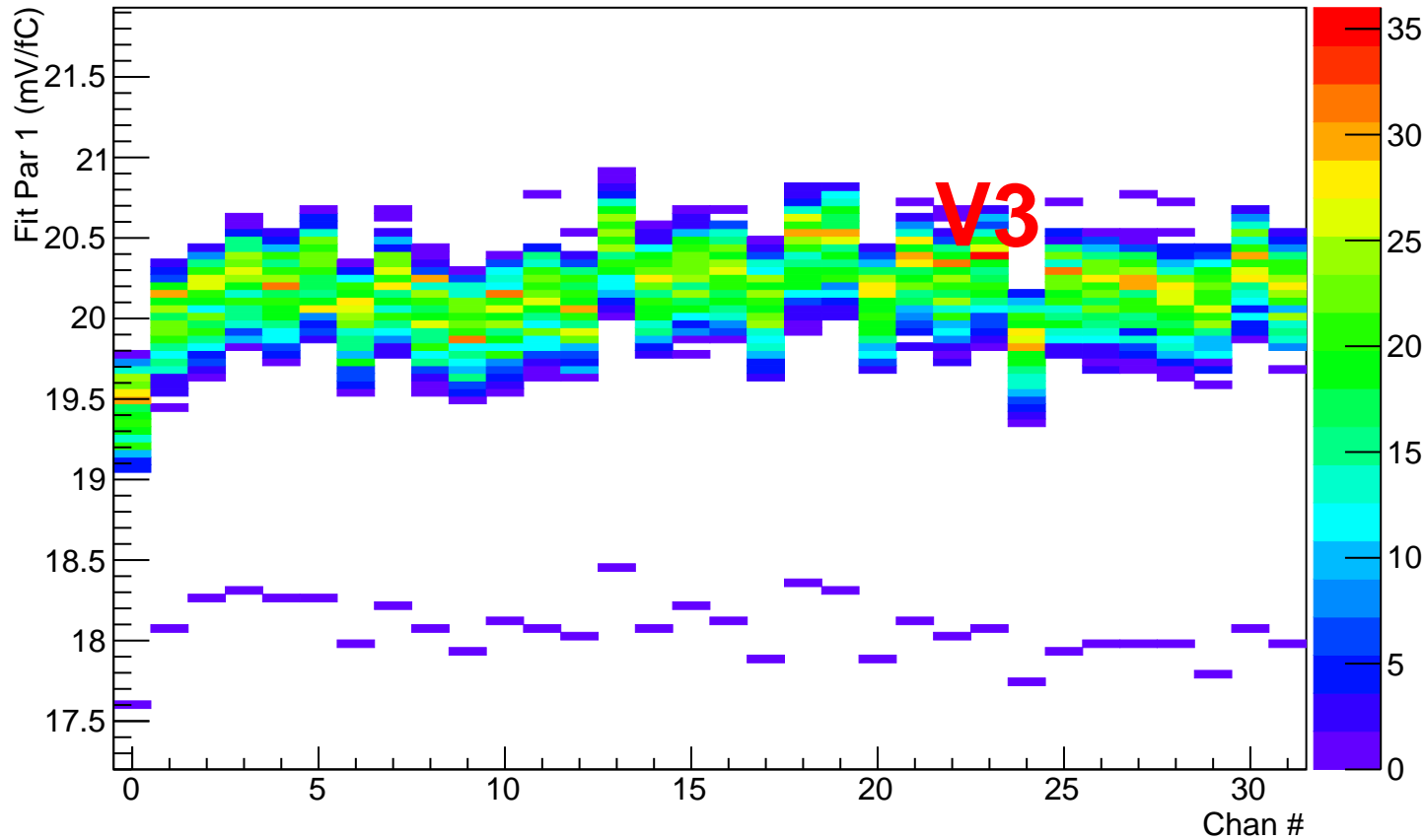
Fit Par 1 (mV/fC) vs Chan #
