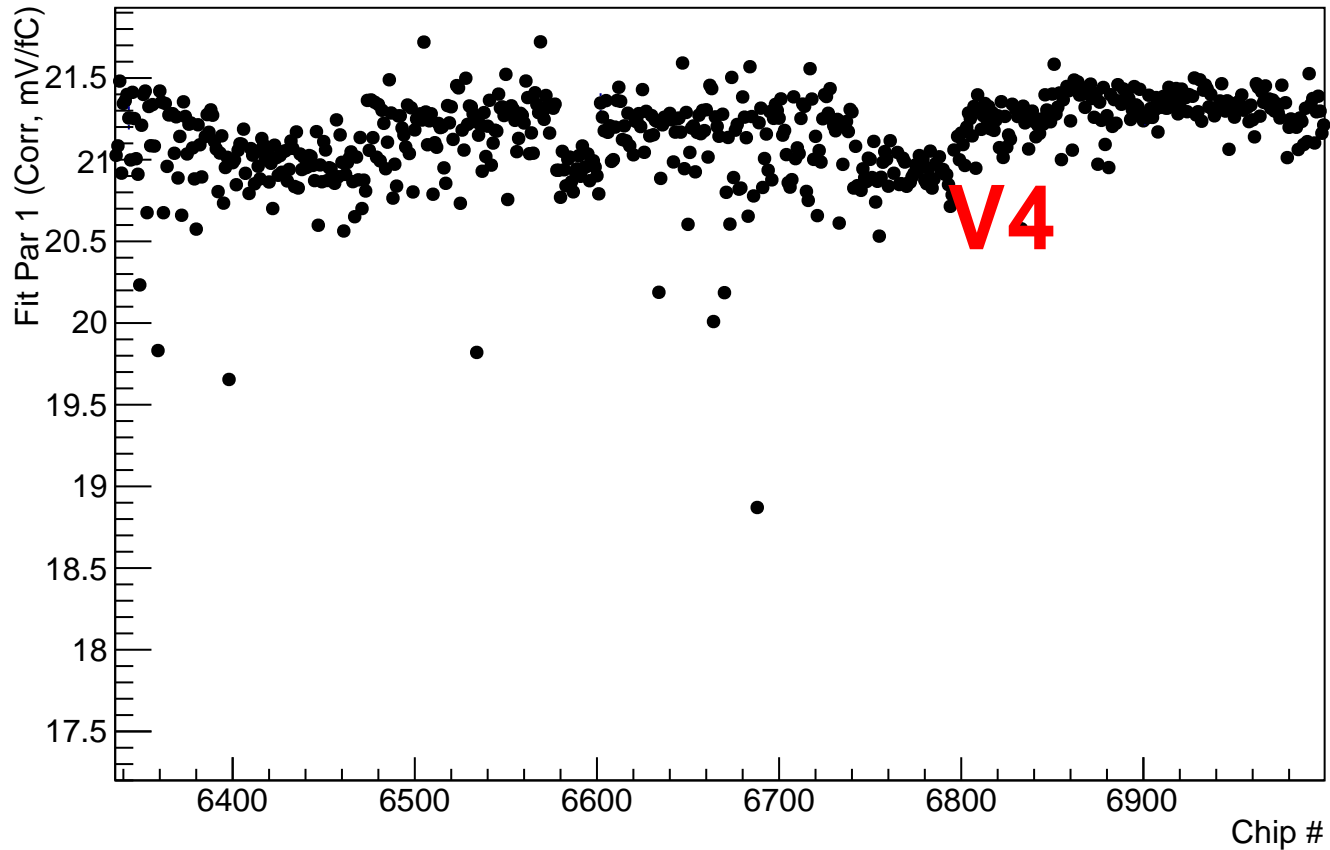
Fit Par 1 (Corr, mV/fC) vs Chip #
