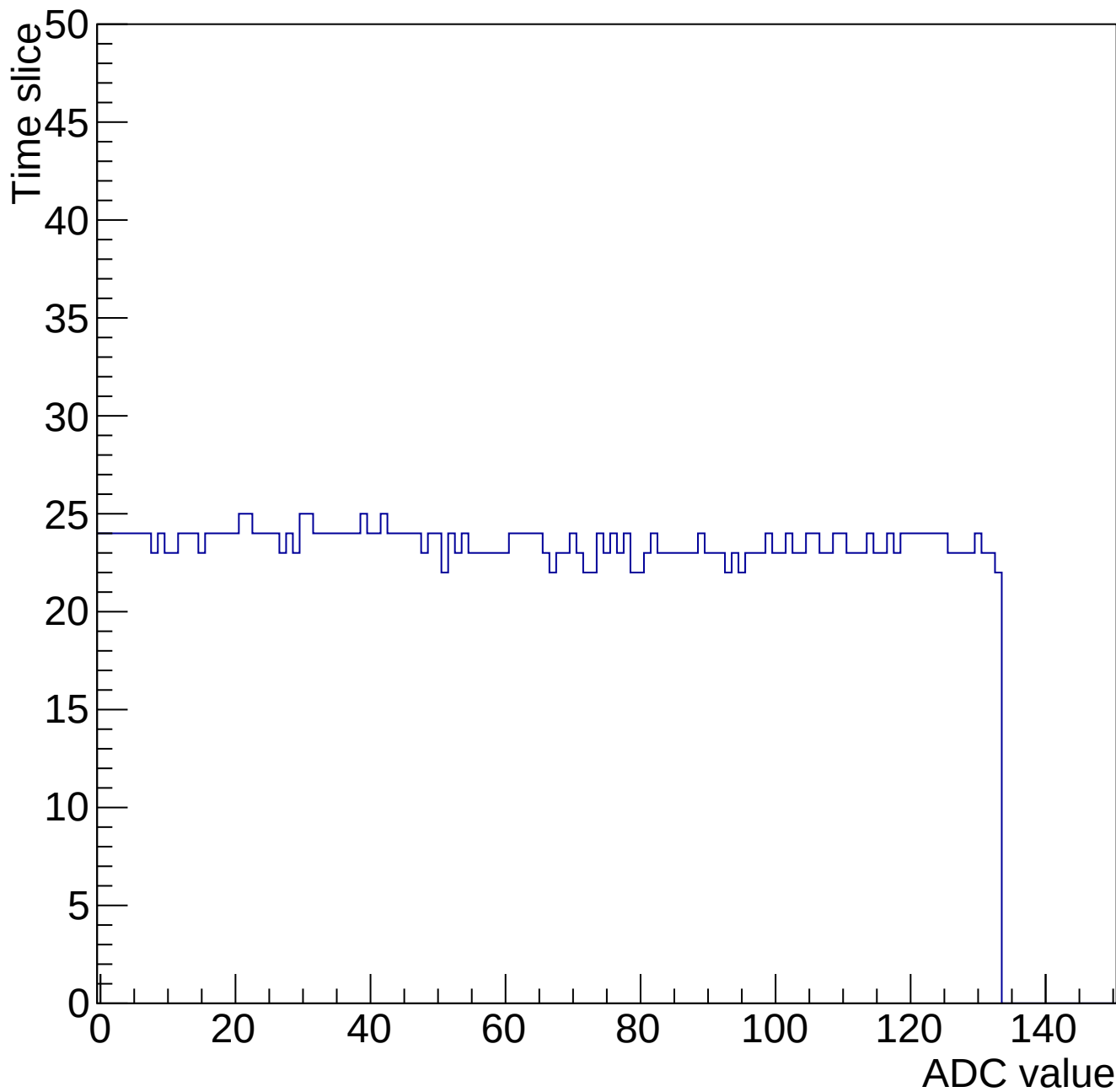
Evt 10 Time mcm 2006 chip 6 chan 13 chip6-nominal-34546
