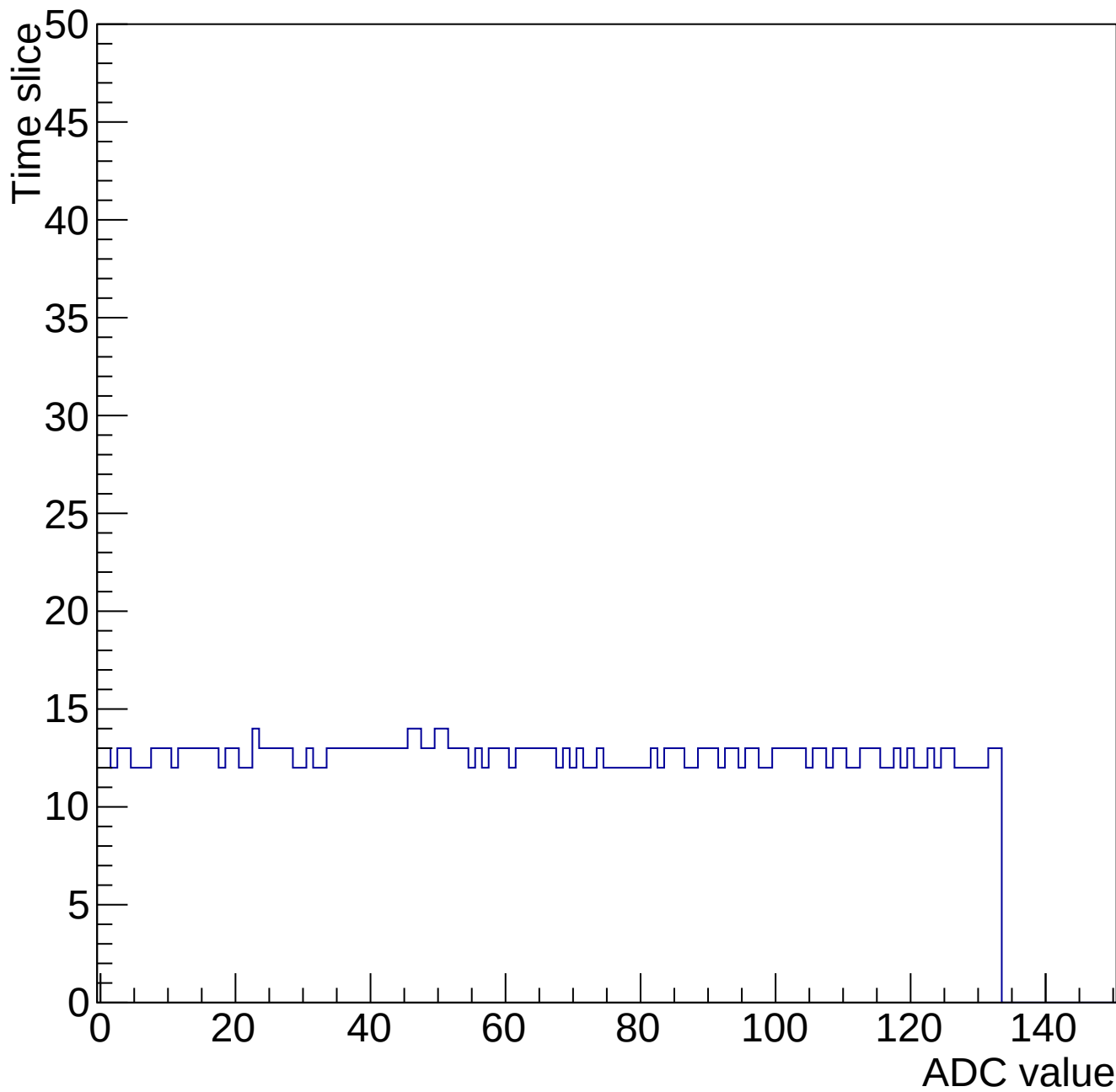
Evt 10 Time mcm 2006 chip 6 chan 9 chip6-nominal-34546
