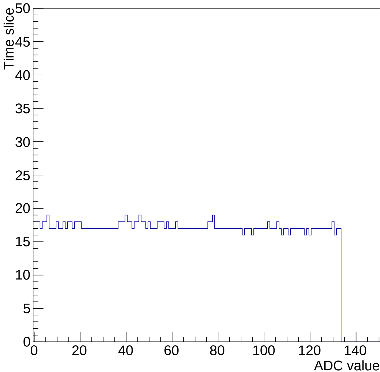
Evt 10 Time mcm 2006 chip 6 chan 12 chip6-nominal-34546
