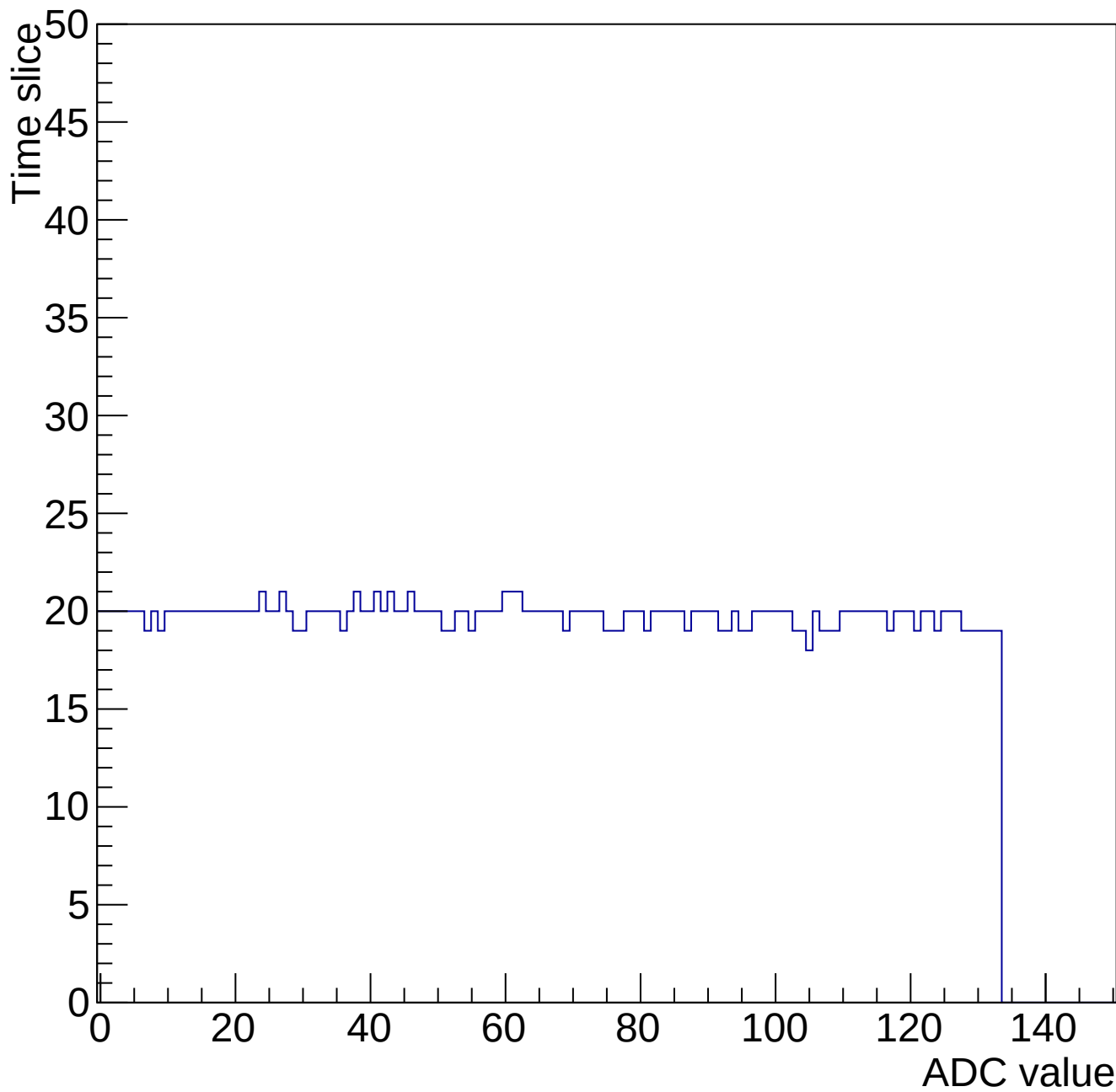
Evt 10 Time mcm 2006 chip 6 chan 2 chip6-nominal-34546
