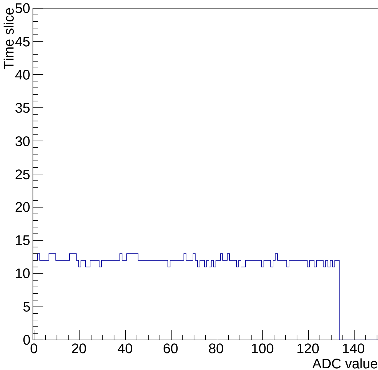
Evt 10 Time mcm 2006 chip 6 chan 15 chip6-nominal-34546
