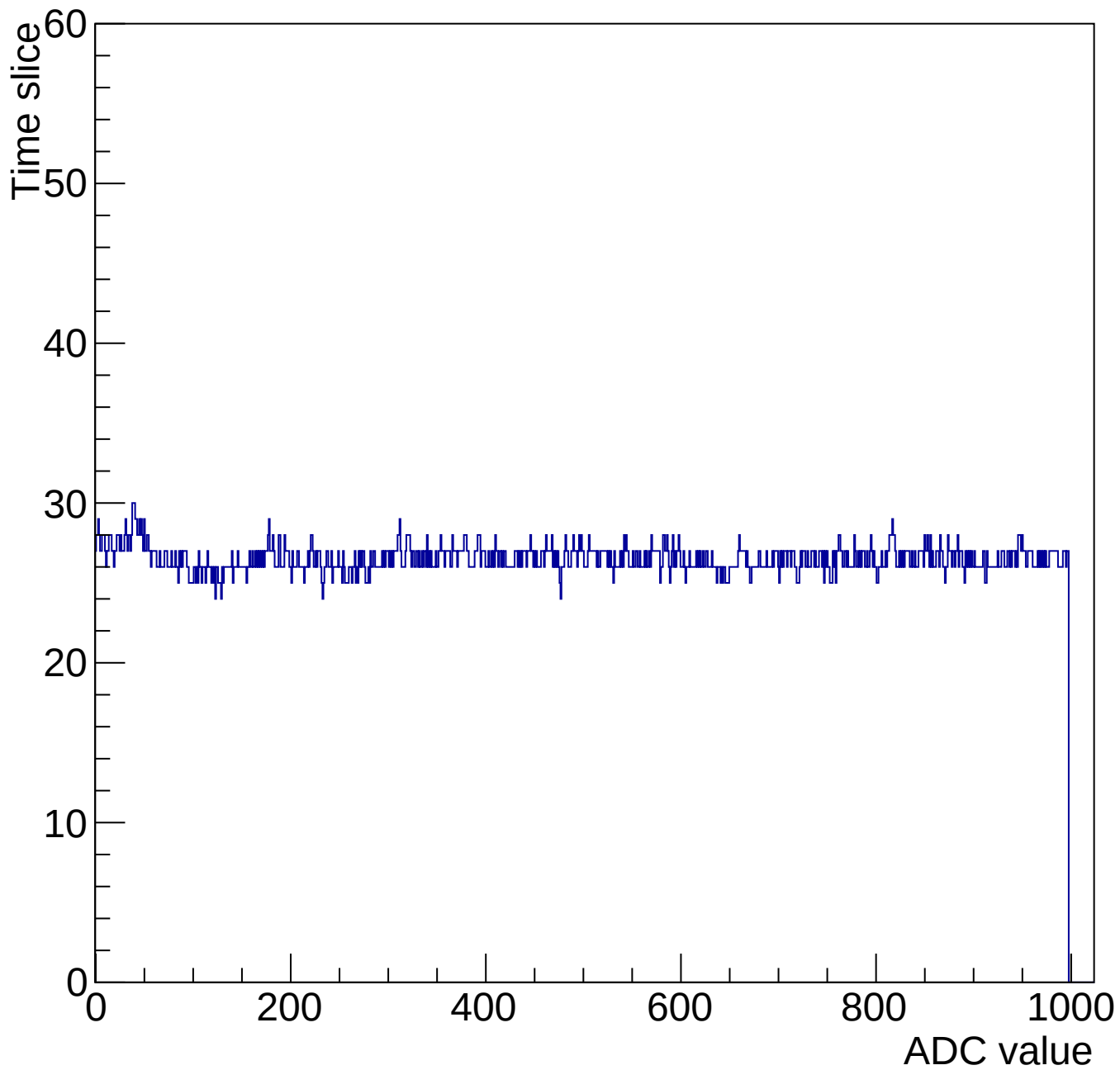
Evt 10 Time mcm 2005 chip 5 chan 6 1000-gain3-shaper0
