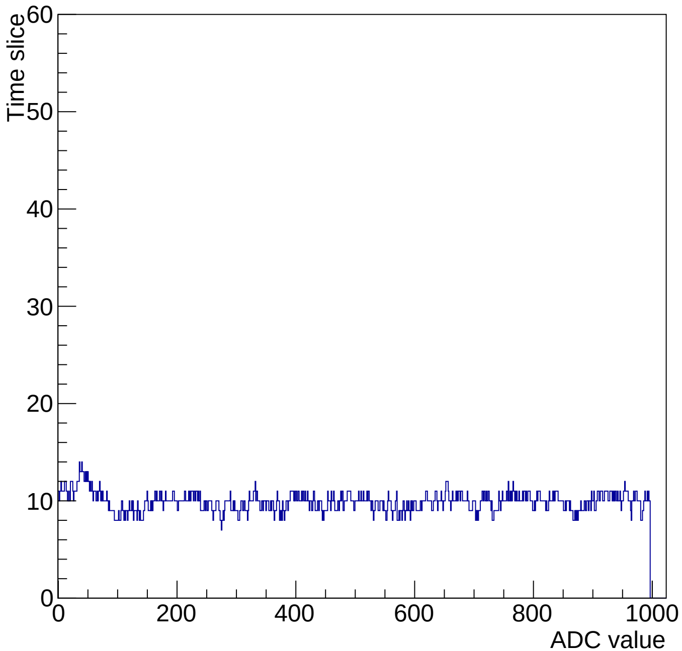
Evt 10 Time mcm 2006 chip 6 chan 3 1000-gain3-shaper0
