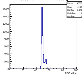
Pedestals mcm 0 ch 118 tlutrig
