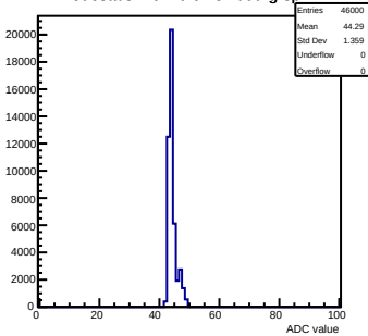
Pedestals mcm 0 ch 32 tlutrig-spill
