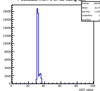
Pedestals mcm 0 ch 18 tlutrig-spill
