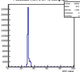
Pedestals mcm 0 ch 40 tlutrig-spill
