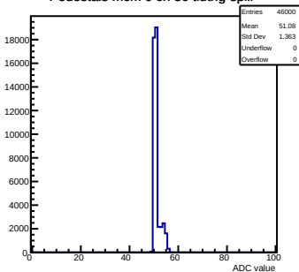
Pedestals mcm 0 ch 36 tlutrig-spill
