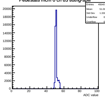
Pedestals mcm 0 ch 83 tlutrig-spill
