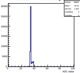
Pedestals mcm 0 ch 33 tlutrig-spill
