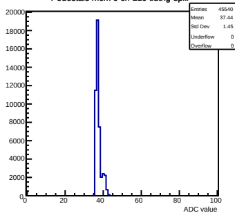
Pedestals mcm 0 ch 110 tlutrig-spill
