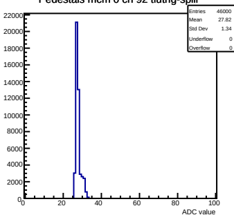
Pedestals mcm 0 ch 92 tlutrig-spill
