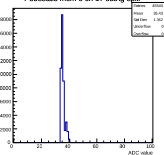
Pedestals mcm 0 ch 17 tlutrig-spill
