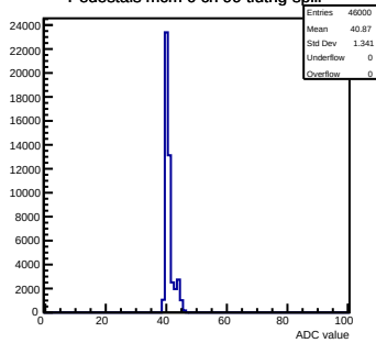
Pedestals mcm 0 ch 99 tlutrig-spill
