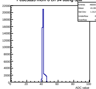
Pedestals mcm 0 ch 94 tlutrig-spill
