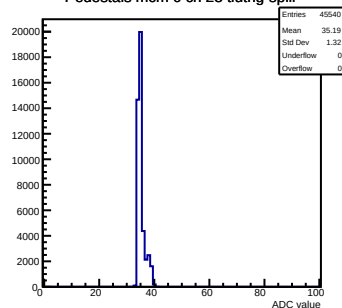
Pedestals mcm 0 ch 23 tlutrig-spill
