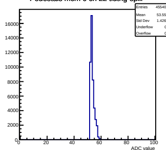
Pedestals mcm 0 ch 22 tlutrig-spill
