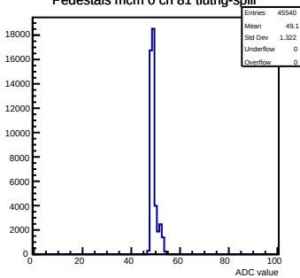
Pedestals mcm 0 ch 81 tlutrig-spill
