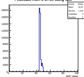
Pedestals mcm 0 ch 89 tlutrig-spill
