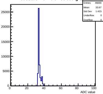
Pedestals mcm 0 ch 35 tlutrig-spill
