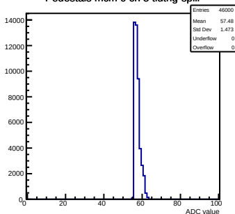
Pedestals mcm 0 ch 5 tlutrig-spill
