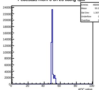
Pedestals mcm 0 ch 26 tlutrig-spill
