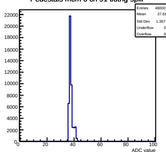
Pedestals mcm 0 ch 91 tlutrig-spill
