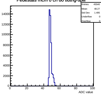
Pedestals mcm 0 ch 80 tlutrig-spill
