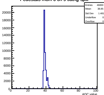
Pedestals mcm 0 ch 9 tlutrig-spill
