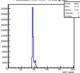
Pedestals mcm 0 ch 43 tlutrig-spill
