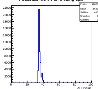
Pedestals mcm 0 ch 6 tlutrig-spill
