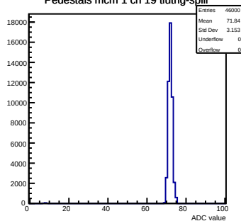
Pedestals mcm 1 ch 19 tlutrig-spill
