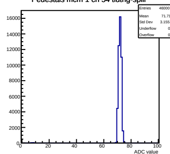
Pedestals mcm 1 ch 54 ttutrig-spill
