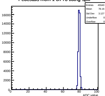
Pedestals mcm 1 ch 73 tlutrig-spill
