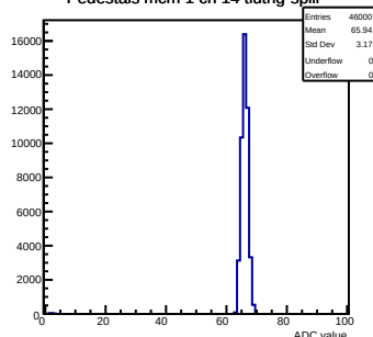
Pedestals mcm 1 ch 14 tlutrig-spill
