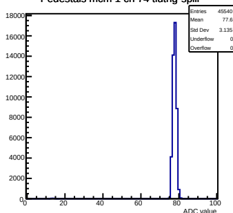
Pedestals mcm 1 ch 74 tlutrig-spill
