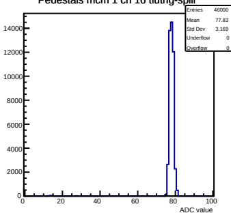
Pedestals mcm 1 ch 16 tlutrig-spill
