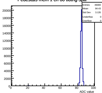
Pedestals mcm 1 ch 60 ttutrig-spill
