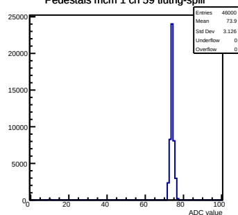
Pedestals mcm 1 ch 59 ttutrig-spill
