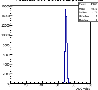
Pedestals mcm 1 ch 20 tlutrig-spill
