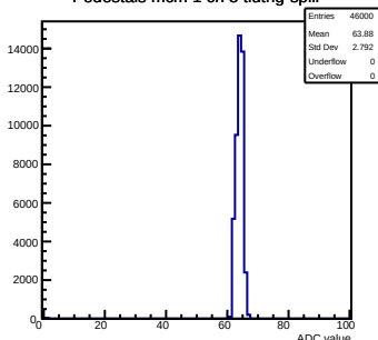
Pedestals mcm 1 ch 5 tlutrig-spill
