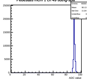
Pedestals mcm 1 ch 49 ttutrig-spill
