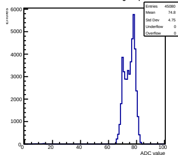
Pedestals mcm 1 ch 25 tlutrig-nospill
