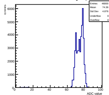
Pedestals mcm 1 ch 31 tlutrig-nospill
