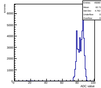
Pedestals mcm 1 ch 23 tlutrig-nospill
