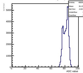
Pedestals mcm 1 ch 6 tlutrig-nospill
