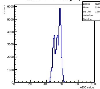
Pedestals mcm 1 ch 10 tlutrig-nospill
