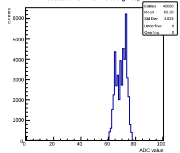
Pedestals mcm 1 ch 15 tlutrig-nospill
