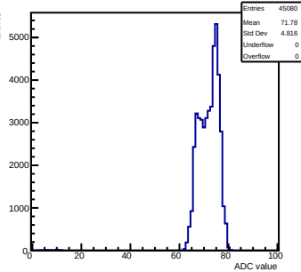
Pedestals mcm 1 ch 20 tlutrig-nospill
