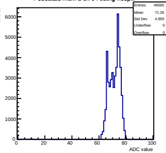
Pedestals mcm 1 ch 64 tlutrig-nospill
