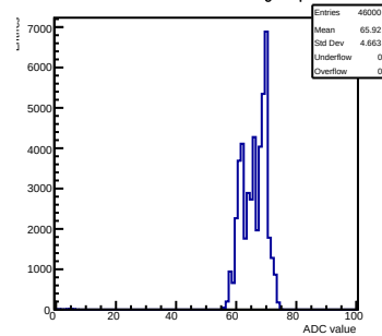
Pedestals mcm 1 ch 70 tlutrig-nospill
