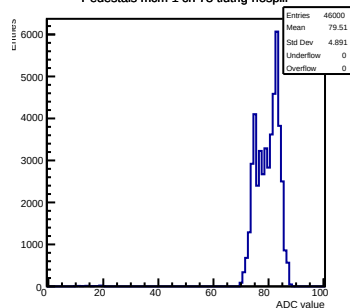
Pedestals mcm 1 ch 73 tlutrig-nospill
