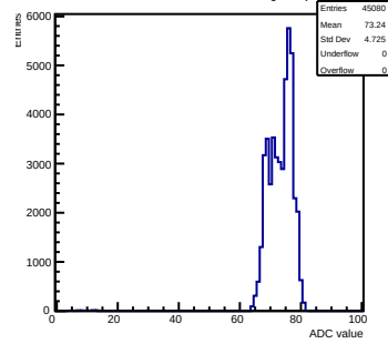
Pedestals mcm 1 ch 19 tlutrig-nospill
