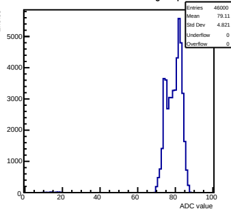
Pedestals mcm 1 ch 28 tlutrig-nospill
