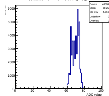
Pedestals mcm 1 ch 78 tlutrig-nospill
