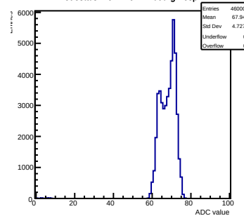
Pedestals mcm 1 ch 14 tlutrig-nospill
