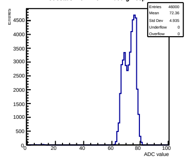
Pedestals mcm 1 ch 11 tlutrig-nospill
