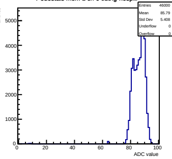
Pedestals mcm 1 ch 0 tlutrig-nospill
