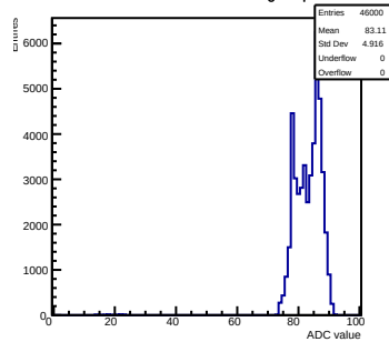
Pedestals mcm 1 ch 69 tlutrig-nospill
