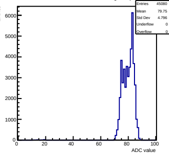
Pedestals mcm 1 ch 16 tlutrig-nospill
