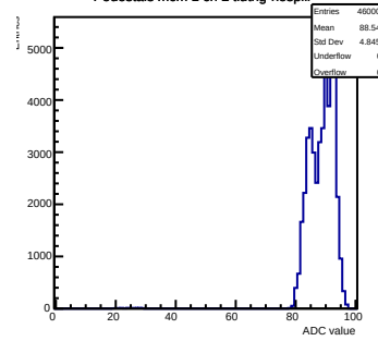
Pedestals mcm 1 ch 2 tlutrig-nospill
