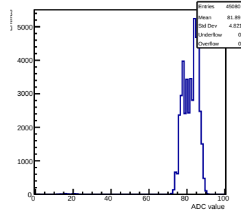
Pedestals mcm 1 ch 22 tlutrig-nospill
