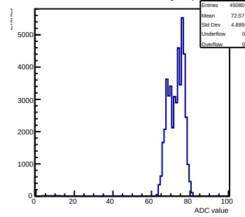
Pedestals mcm 1 ch 18 tlutrig-nospill
