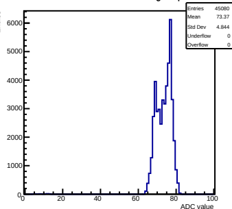
Pedestals mcm 1 ch 24 tlutrig-nospill
