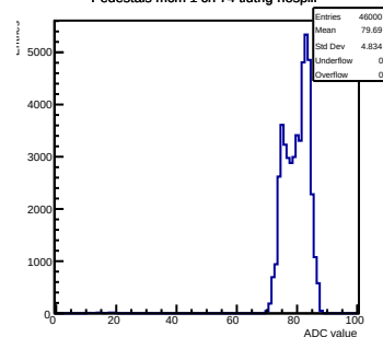
Pedestals mcm 1 ch 74 tlutrig-nospill
