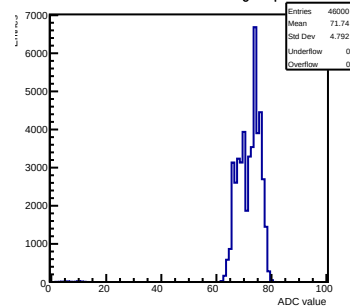
Pedestals mcm 1 ch 30 tlutrig-nospill
