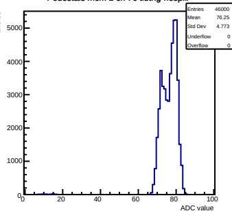
Pedestals mcm 1 ch 76 tlutrig-nospill
