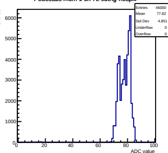
Pedestals mcm 1 ch 72 tlutrig-nospill
