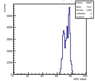
Pedestals mcm 1 ch 7 tlutrig-nospill
