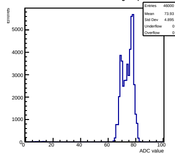
Pedestals mcm 1 ch 71 tlutrig-nospill
