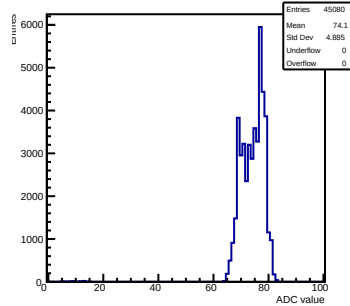
Pedestals mcm 1 ch 21 tlutrig-nospill
