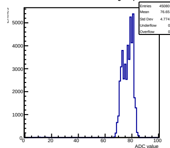
Pedestals mcm 1 ch 26 tlutrig-nospill
