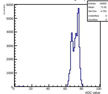
Pedestals mcm 1 ch 29 tlutrig-nospill
