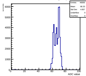
Pedestals mcm 1 ch 5 tlutrig-nospill
