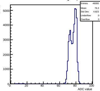
Pedestals mcm 1 ch 68 tlutrig-nospill
