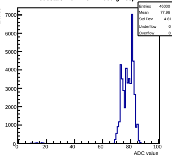
Pedestals mcm 1 ch 12 tlutrig-nospill
