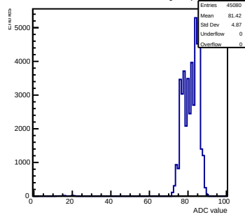
Pedestals mcm 1 ch 17 tlutrig-nospill
