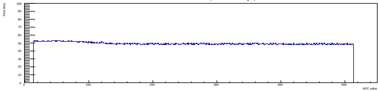
Run 8 Evt 19 Time mcm 0 chip 5 chan 7 tlutrig-spill
