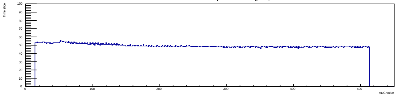
Run 9 Evt 19 Time mcm 0 chip 1 chan 0 tlutrig-nospill
