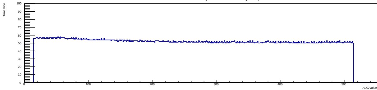
Run 9 Evt 19 Time mcm 0 chip 7 chan 13 tlutrig-nospill
