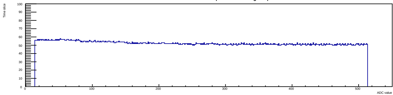
Run 9 Evt 19 Time mcm 0 chip 5 chan 7 tlutrig-nospill
