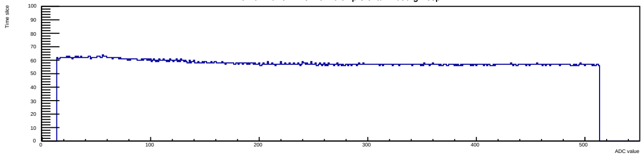
Run 9 Evt 19 Time mcm 0 chip 3 chan 4 tlutrig-nospill
