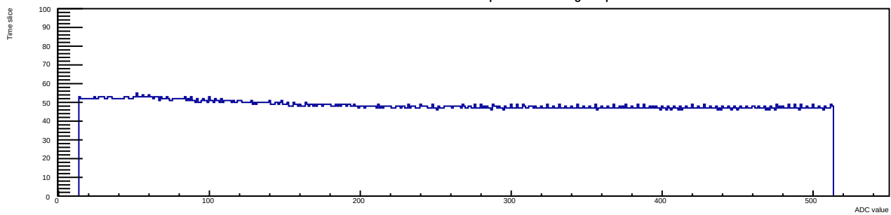
Run 9 Evt 19 Time mcm 0 chip 7 chan 3 tlutrig-nospill
