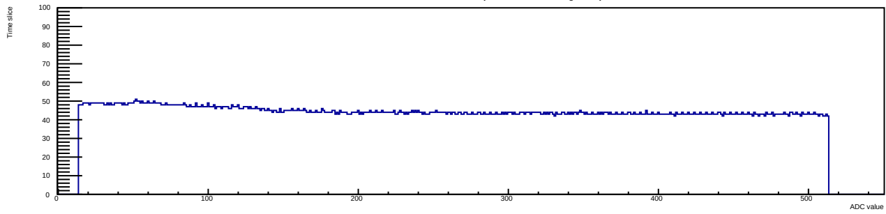
Run 9 Evt 2 Time mcm 0 chip 7 chan 9 tlutrig-nospill
