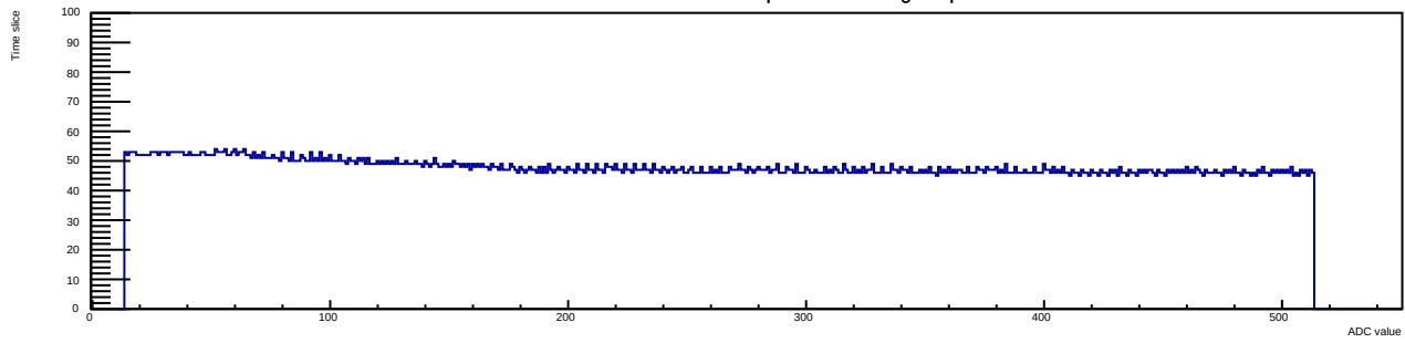
Run 9 Evt 2 Time mcm 0 chip 0 chan 4 tlutrig-nospill
