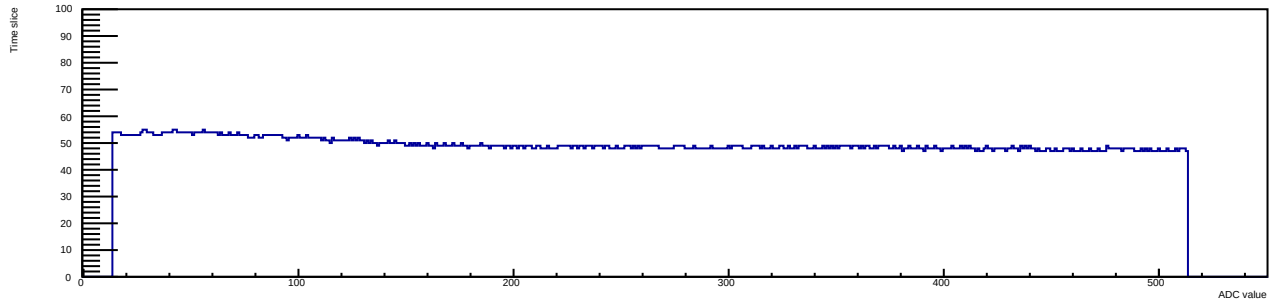
Run 9 Evt 2 Time mcm 0 chip 2 chan 5 tlutrig-nospill
