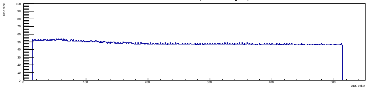
Run 9 Evt 2 Time mcm 0 chip 7 chan 3 tlutrig-nospill
