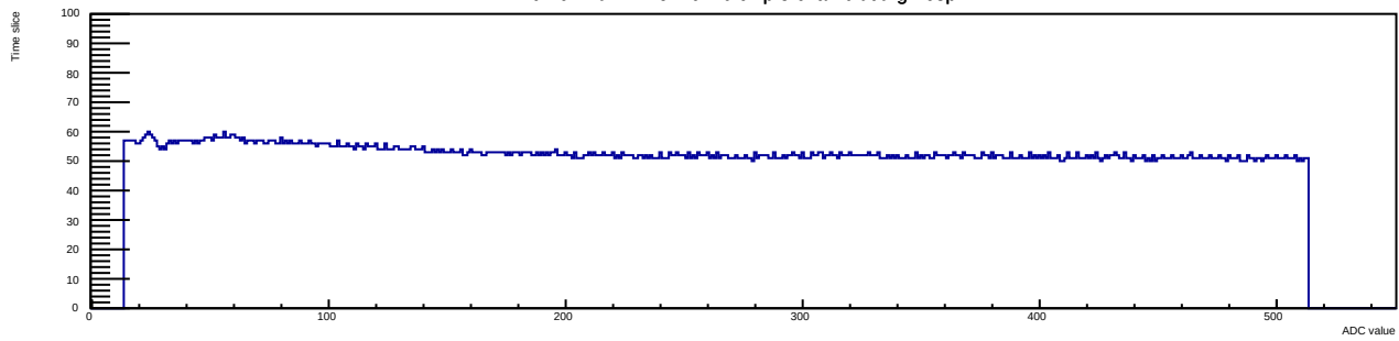
Run 9 Evt 2 Time mcm 0 chip 3 chan 0 tlutrig-nospill
