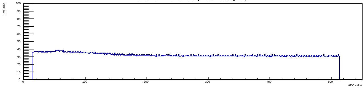
Run 9 Evt 2 Time mcm 0 chip 7 chan 0 tlutrig-nospill
