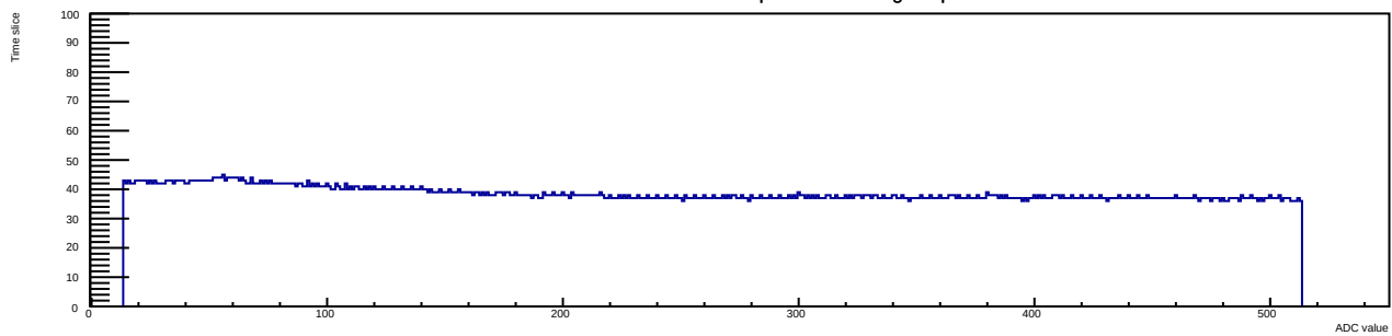
Run 9 Evt 2 Time mcm 0 chip 1 chan 7 tlutrig-nospill
