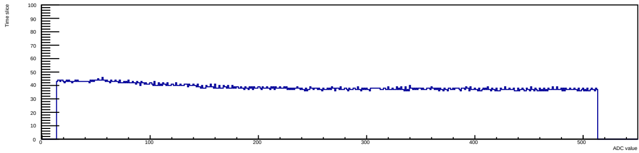
Run 9 Evt 2 Time mcm 0 chip 0 chan 6 tlutrig-nospill
