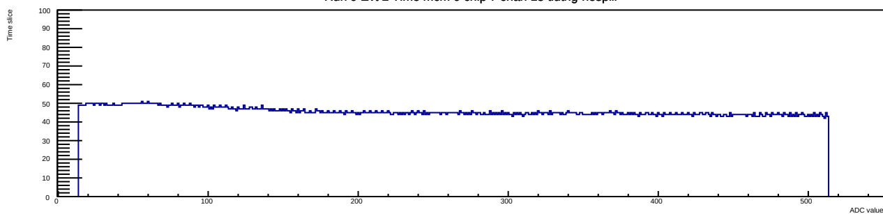
Run 9 Evt 2 Time mcm 0 chip 7 chan 15 tlutrig-nospill
