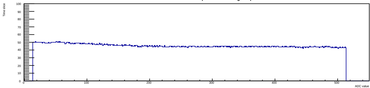
Run 9 Evt 2 Time mcm 0 chip 4 chan 2 tlutrig-nospill
