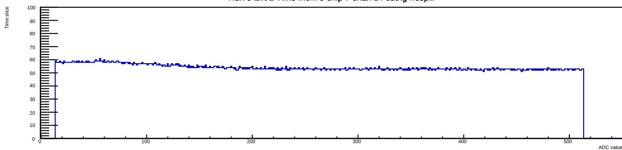
Run 9 Evt 2 Time mcm 0 chip 7 chan 14 tlutrig-nospill
