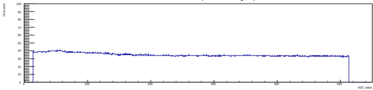
Run 9 Evt 2 Time mcm 0 chip 3 chan 14 tlutrig-nospill
