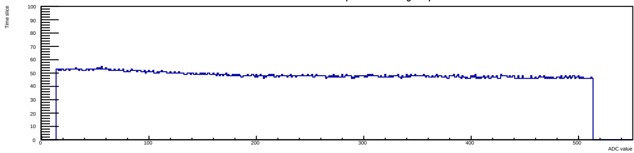
Run 9 Evt 2 Time mcm 0 chip 3 chan 2 tlutrig-nospill
