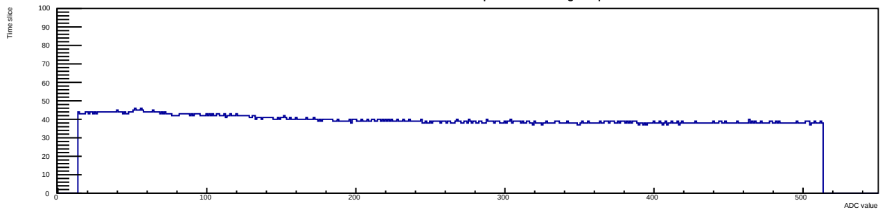
Run 9 Evt 99 Time mcm 0 chip 4 chan 5 tlutrig-nospill
