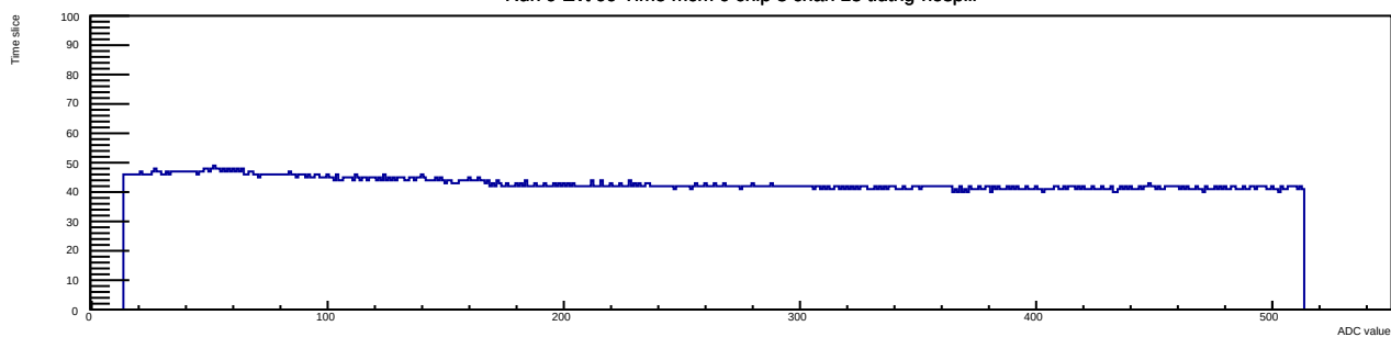
Run 9 Evt 99 Time mcm 0 chip 3 chan 15 tlutrig-nospill
