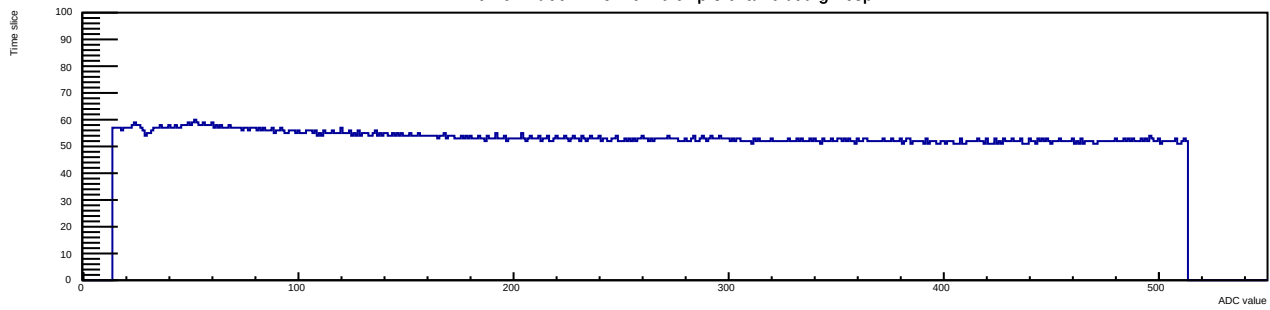
Run 9 Evt 99 Time mcm 0 chip 3 chan 0 tlutrig-nospill
