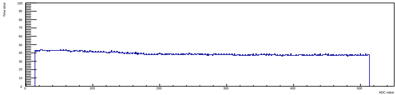
Run 9 Evt 99 Time mcm 0 chip 1 chan 7 tlutrig-nospill
