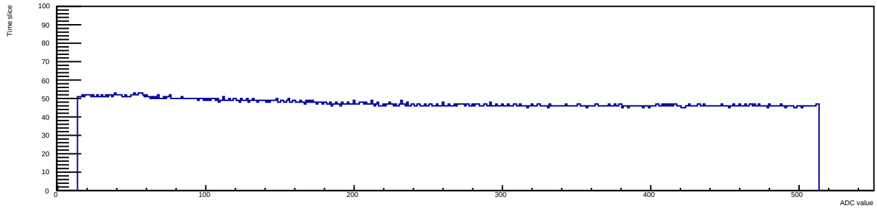
Run 9 Evt 99 Time mcm 0 chip 5 chan 9 tlutrig-nospill
