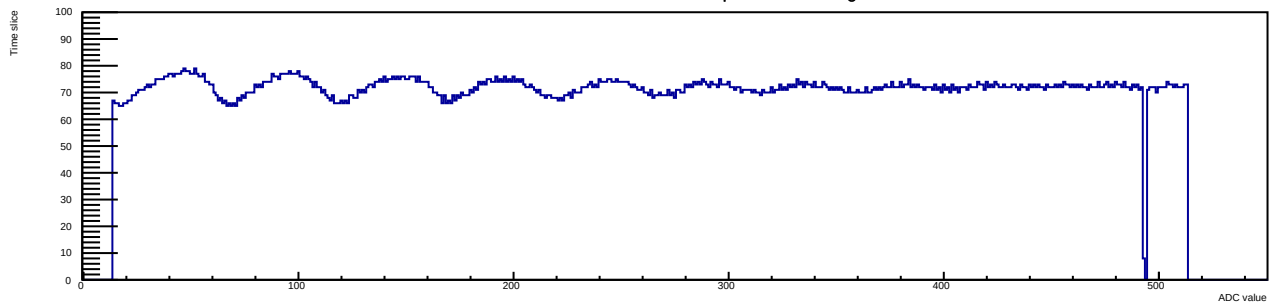
Run 7 Evt 19 Time mcm 1 chip 0 chan 9 swtrig
