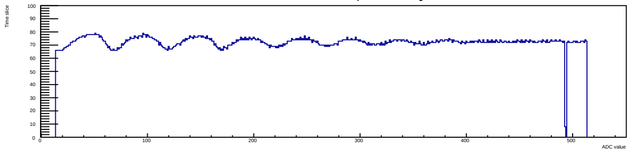
Run 7 Evt 19 Time mcm 1 chip 0 chan 7 swtrig
