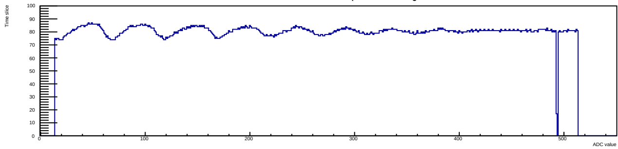
Run 7 Evt 19 Time mcm 1 chip 7 chan 1 swtrig
