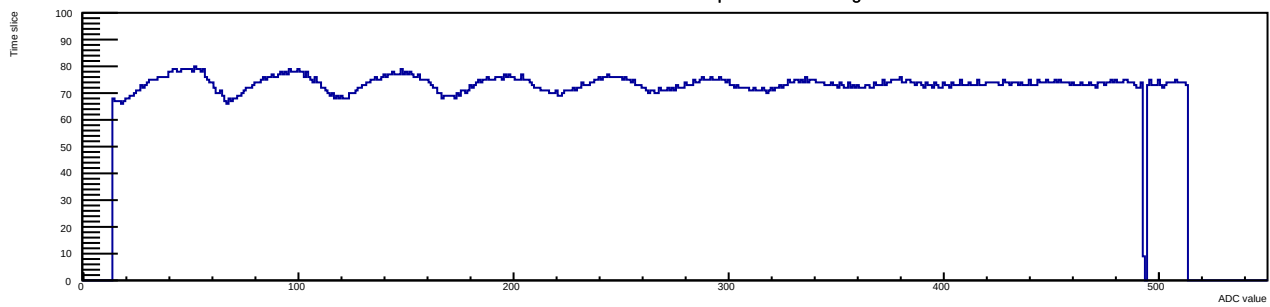
Run 7 Evt 19 Time mcm 1 chip 3 chan 10 swtrig
