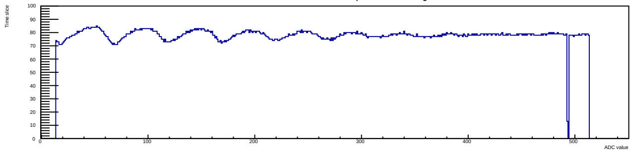
Run 7 Evt 19 Time mcm 1 chip 5 chan 13 swtrig
