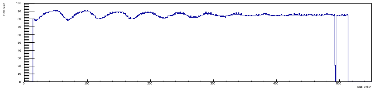
Run 7 Evt 19 Time mcm 1 chip 5 chan 1 swtrig
