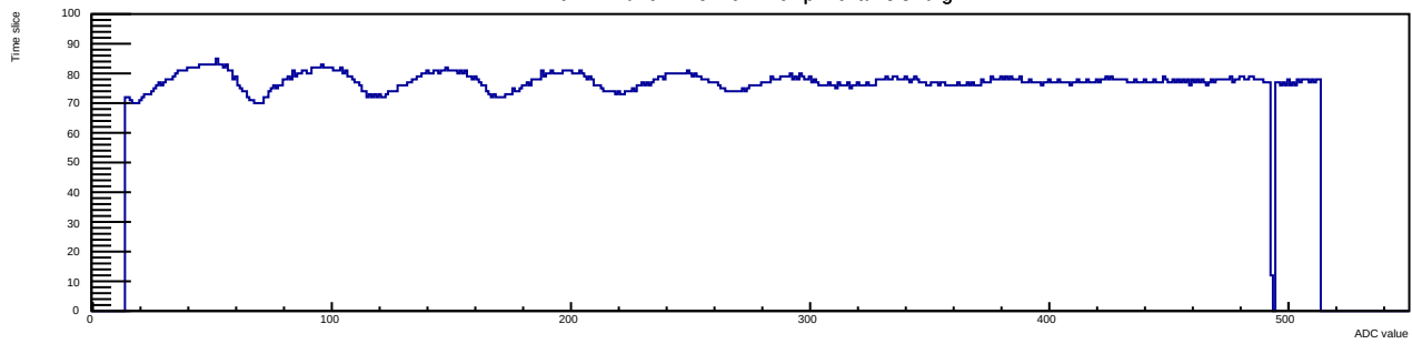
Run 7 Evt 19 Time mcm 1 chip 4 chan 8 swtrig
