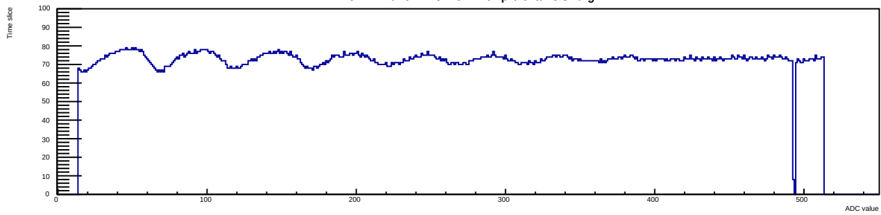
Run 7 Evt 19 Time mcm 1 chip 6 chan 8 swtrig
