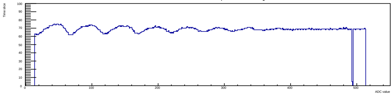
Run 7 Evt 19 Time mcm 1 chip 4 chan 15 swtrig
