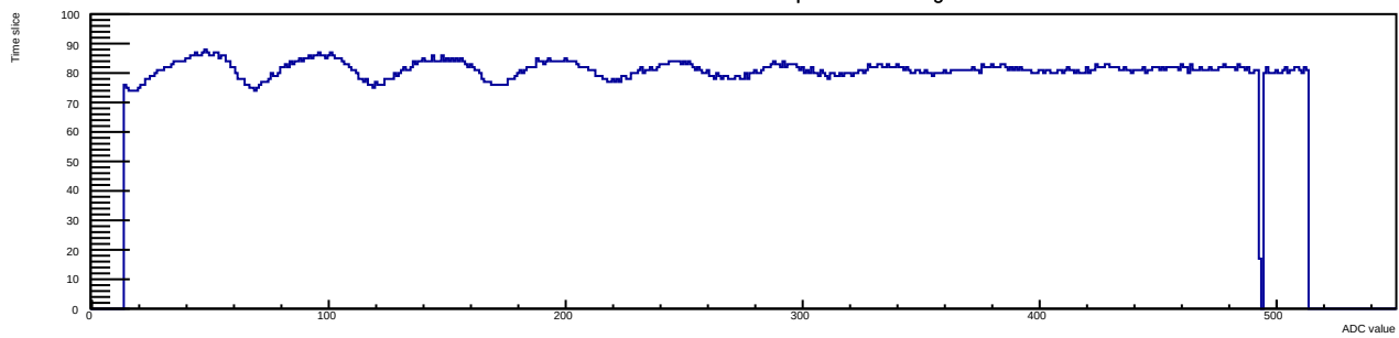
Run 7 Evt 19 Time mcm 1 chip 1 chan 6 swtrig
