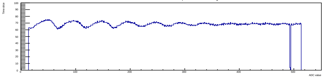
Run 7 Evt 19 Time mcm 1 chip 0 chan 15 swtrig
