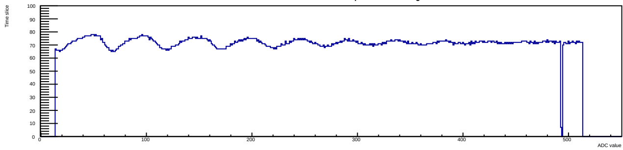
Run 7 Evt 19 Time mcm 1 chip 6 chan 6 swtrig
