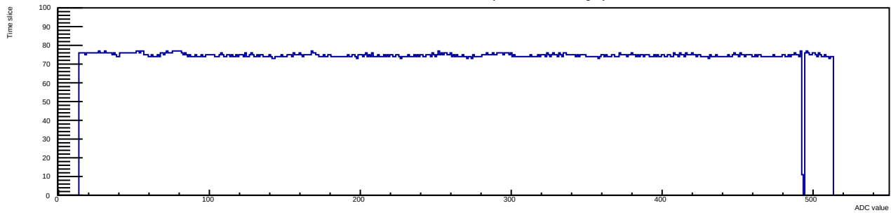
Run 8 Evt 19 Time mcm 1 chip 3 chan 13 tlutrig-spill
