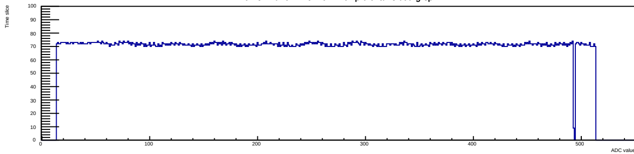
Run 8 Evt 19 Time mcm 1 chip 0 chan 8 tlutrig-spill
