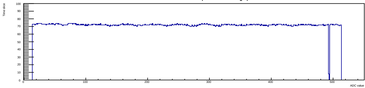
Run 8 Evt 19 Time mcm 1 chip 7 chan 11 tlutrig-spill
