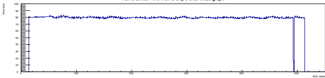
Run 8 Evt 19 Time mcm 1 chip 0 chan 6 tlutrig-spill
