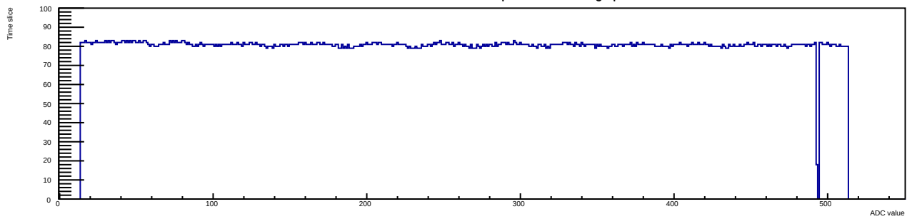
Run 8 Evt 19 Time mcm 1 chip 5 chan 11 tlutrig-spill
