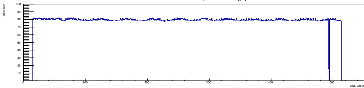
Run 8 Evt 19 Time mcm 1 chip 7 chan 1 tlutrig-spill
