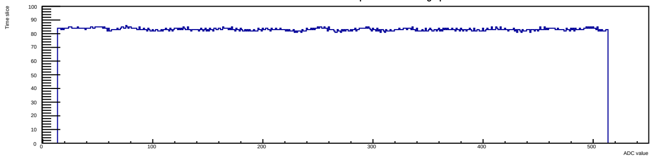
Run 8 Evt 19 Time mcm 1 chip 7 chan 15 tlutrig-spill
