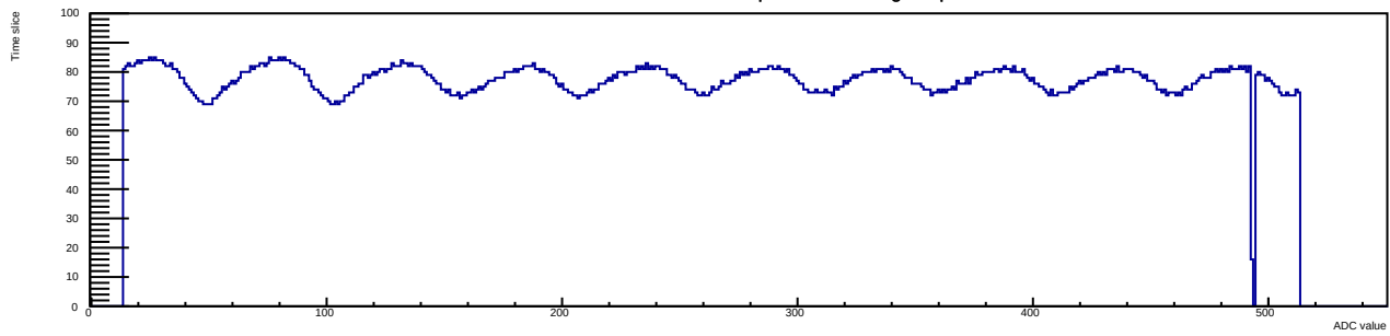
Run 9 Evt 2 Time mcm 1 chip 6 chan 9 tlutrig-nospill
