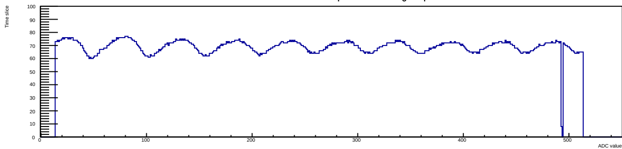
Run 9 Evt 2 Time mcm 1 chip 4 chan 14 tlutrig-nospill
