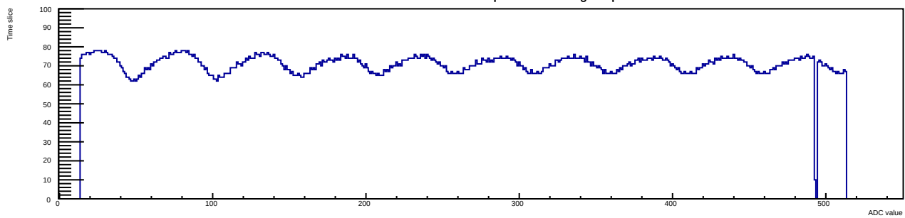
Run 9 Evt 2 Time mcm 1 chip 0 chan 3 tlutrig-nospill
