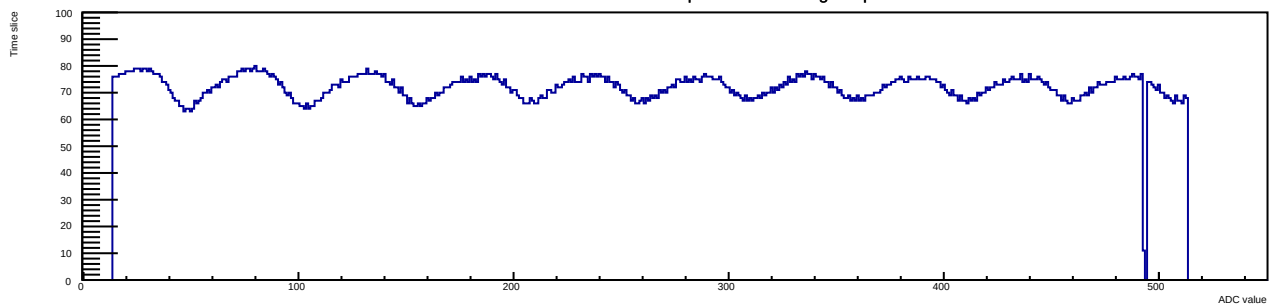
Run 9 Evt 2 Time mcm 1 chip 0 chan 11 tlutrig-nospill
