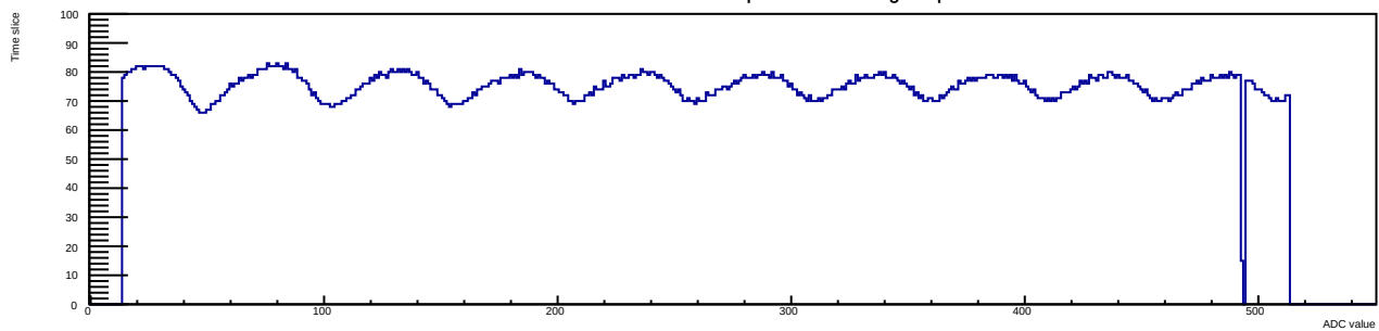
Run 9 Evt 2 Time mcm 1 chip 7 chan 14 tlutrig-nospill
