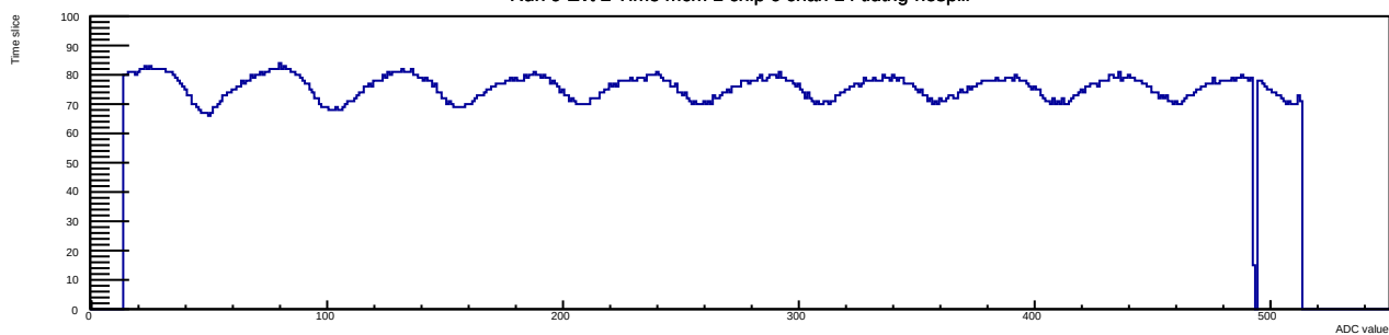
Run 9 Evt 2 Time mcm 1 chip 6 chan 14 tlutrig-nospill
