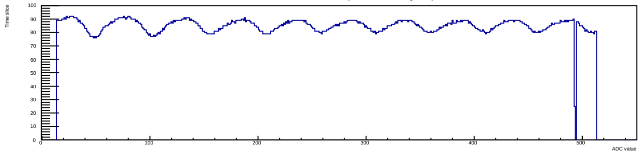
Run 9 Evt 2 Time mcm 1 chip 6 chan 1 tlutrig-nospill
