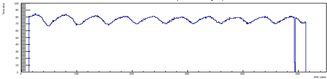
Run 9 Evt 2 Time mcm 1 chip 2 chan 11 tlutrig-nospill
