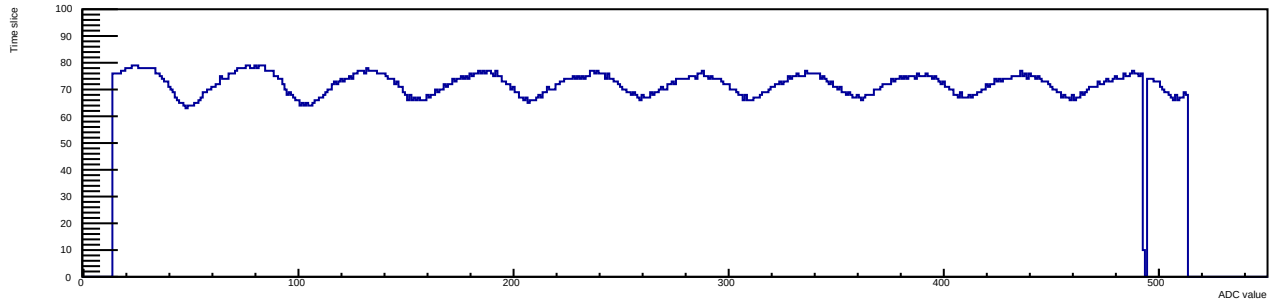
Run 9 Evt 2 Time mcm 1 chip 6 chan 5 tlutrig-nospill
