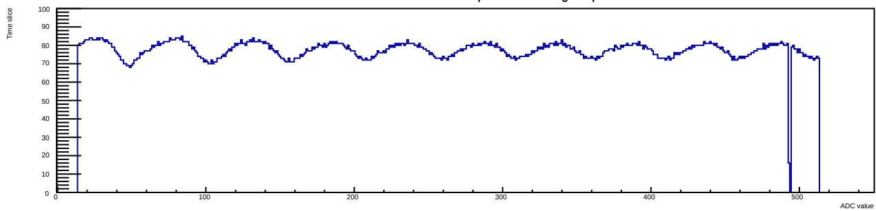
Run 9 Evt 2 Time mcm 1 chip 3 chan 3 tlutrig-nospill
