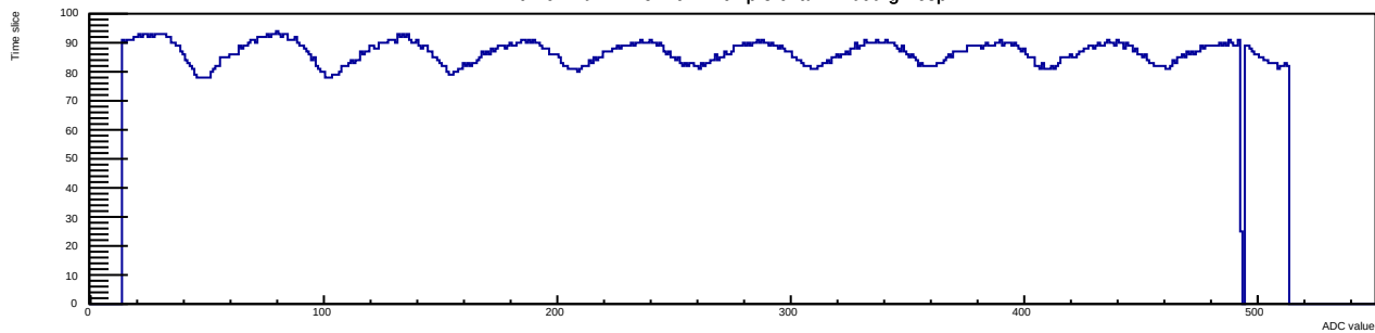
Run 9 Evt 2 Time mcm 1 chip 3 chan 12 tlutrig-nospill
