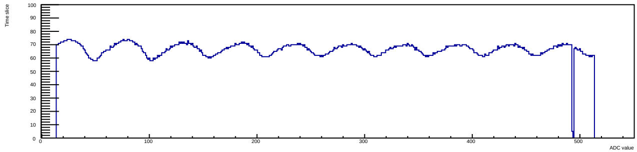
Run 9 Evt 2 Time mcm 1 chip 1 chan 11 tlutrig-nospill
