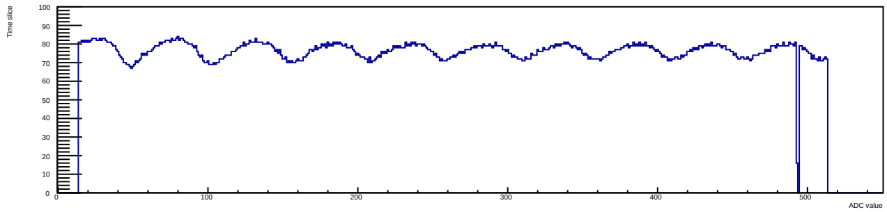
Run 9 Evt 2 Time mcm 1 chip 1 chan 10 tlutrig-nospill
