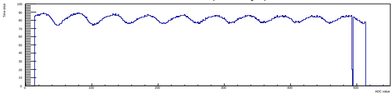
Run 9 Evt 2 Time mcm 1 chip 1 chan 6 tlutrig-nospill
