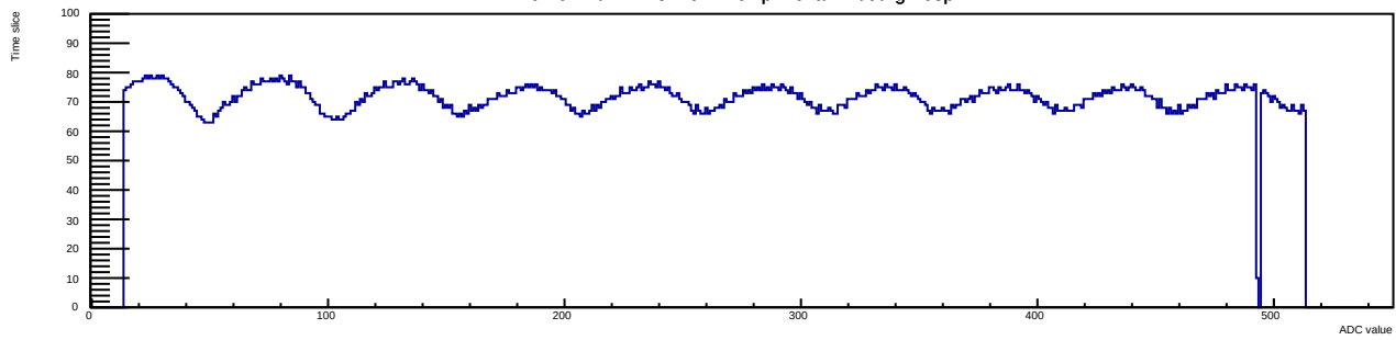
Run 9 Evt 2 Time mcm 1 chip 1 chan 4 tlutrig-nospill
