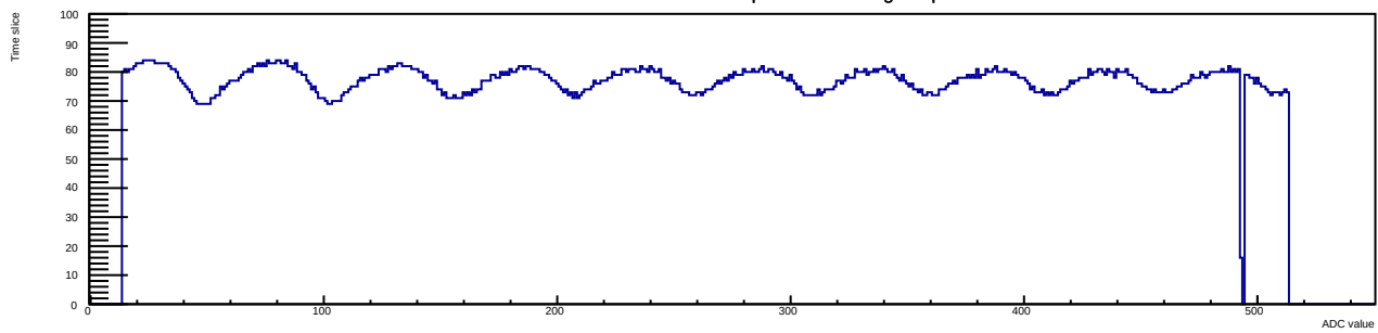
Run 9 Evt 2 Time mcm 1 chip 3 chan 2 tlutrig-nospill
