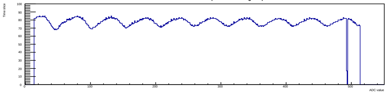
Run 9 Evt 99 Time mcm 1 chip 3 chan 2 tlutrig-nospill
