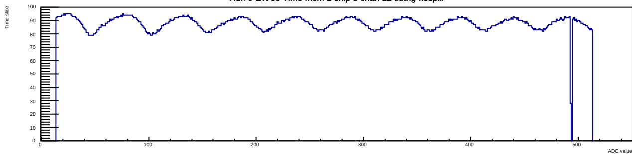
Run 9 Evt 99 Time mcm 1 chip 5 chan 12 tlutrig-nospill
