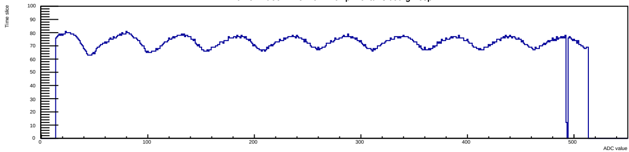
Run 9 Evt 99 Time mcm 1 chip 7 chan 8 tlutrig-nospill
