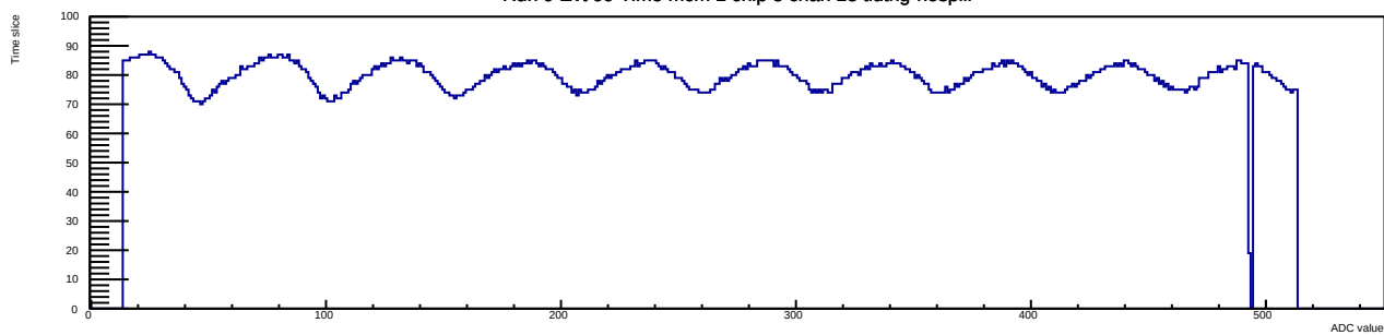
Run 9 Evt 99 Time mcm 1 chip 5 chan 13 tlutrig-nospill
