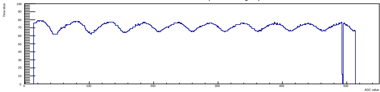
Run 9 Evt 99 Time mcm 1 chip 5 chan 7 tlutrig-nospill
