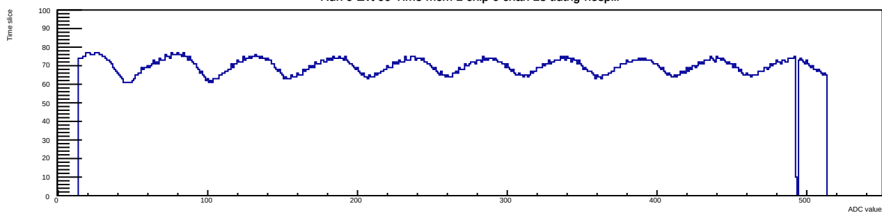
Run 9 Evt 99 Time mcm 1 chip 0 chan 15 tlutrig-nospill
