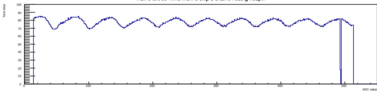
Run 9 Evt 99 Time mcm 1 chip 3 chan 14 tlutrig-nospill
