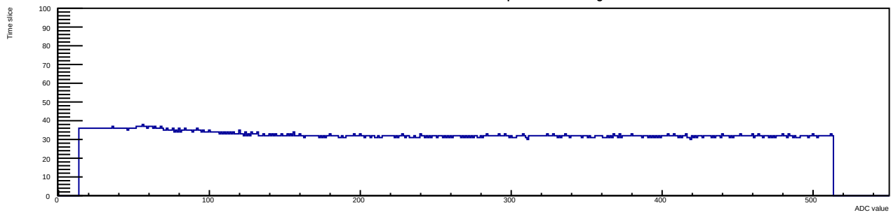
Run 12 Evt 4 Time mcm 0 chip 1 chan 2 30deg
