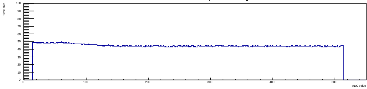
Run 12 Evt 4 Time mcm 0 chip 2 chan 0 30deg
