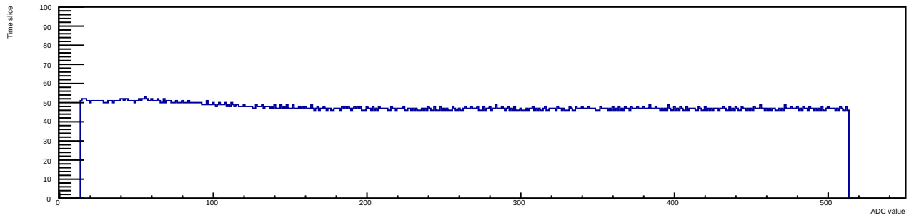
Run 12 Evt 4 Time mcm 0 chip 5 chan 2 30deg
