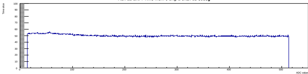
Run 12 Evt 4 Time mcm 0 chip 1 chan 15 30deg
