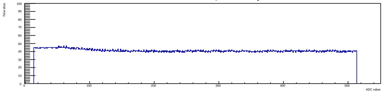
Run 12 Evt 4 Time mcm 0 chip 0 chan 11 30deg
