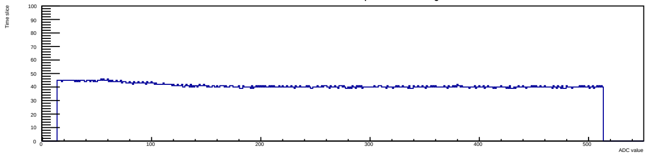
Run 12 Evt 4 Time mcm 0 chip 6 chan 10 30deg
