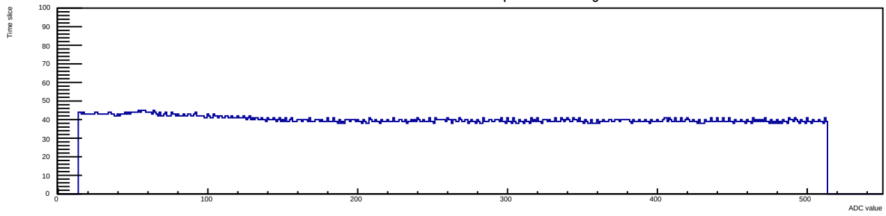
Run 12 Evt 4 Time mcm 0 chip 7 chan 8 30deg
