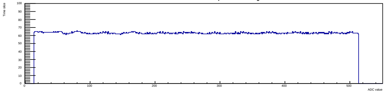
Run 12 Evt 1 Time mcm 1 chip 2 chan 8 30deg
