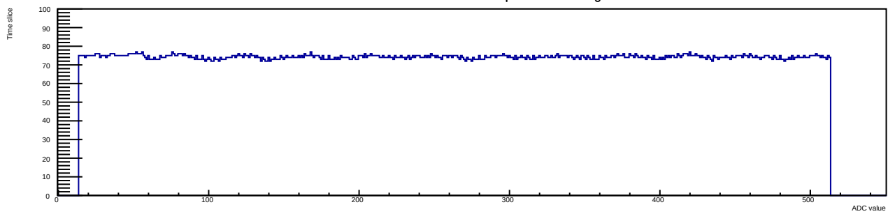
Run 12 Evt 1 Time mcm 1 chip 7 chan 2 30deg
