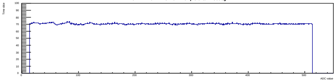
Run 12 Evt 1 Time mcm 1 chip 5 chan 4 30deg
