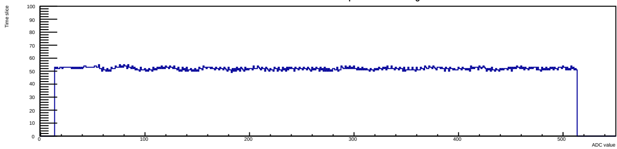
Run 12 Evt 1 Time mcm 1 chip 0 chan 10 30deg
