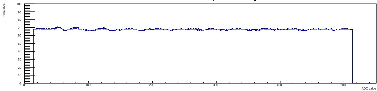
Run 12 Evt 1 Time mcm 1 chip 4 chan 14 30deg
