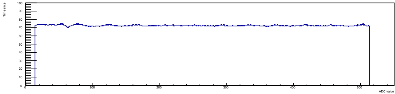
Run 12 Evt 1 Time mcm 1 chip 4 chan 7 30deg
