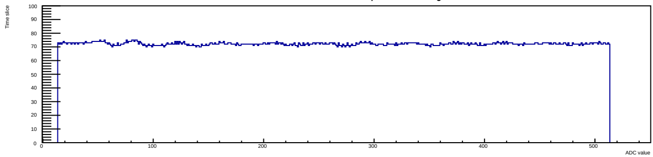
Run 12 Evt 1 Time mcm 1 chip 7 chan 7 30deg
