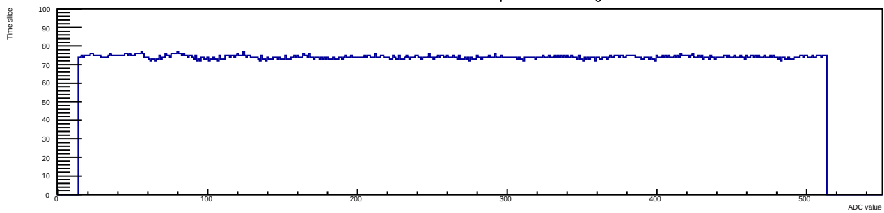
Run 12 Evt 1 Time mcm 1 chip 7 chan 14 30deg
