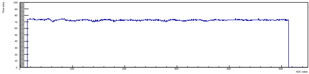
Run 12 Evt 1 Time mcm 1 chip 3 chan 6 30deg
