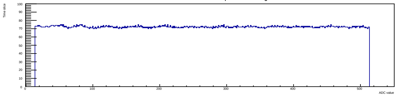
Run 12 Evt 1 Time mcm 1 chip 1 chan 3 30deg
