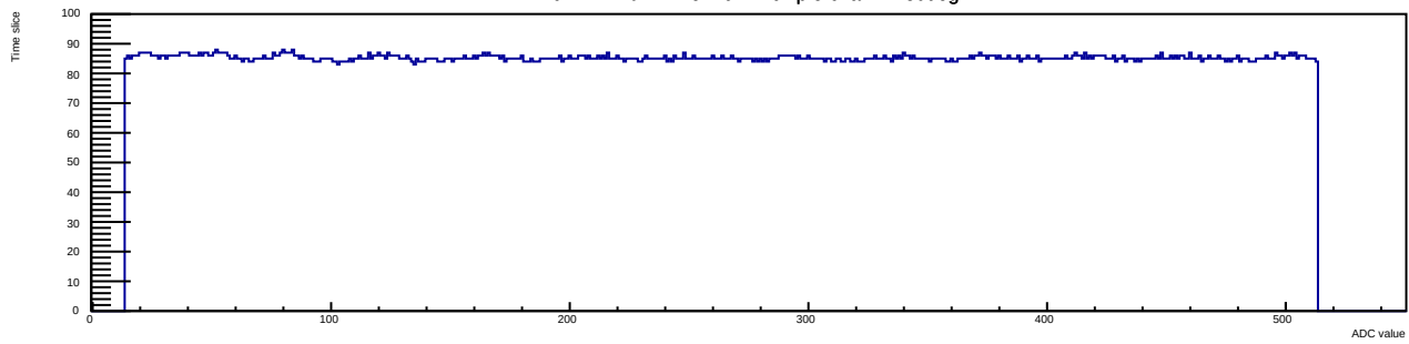
Run 12 Evt 1 Time mcm 1 chip 5 chan 12 30deg
