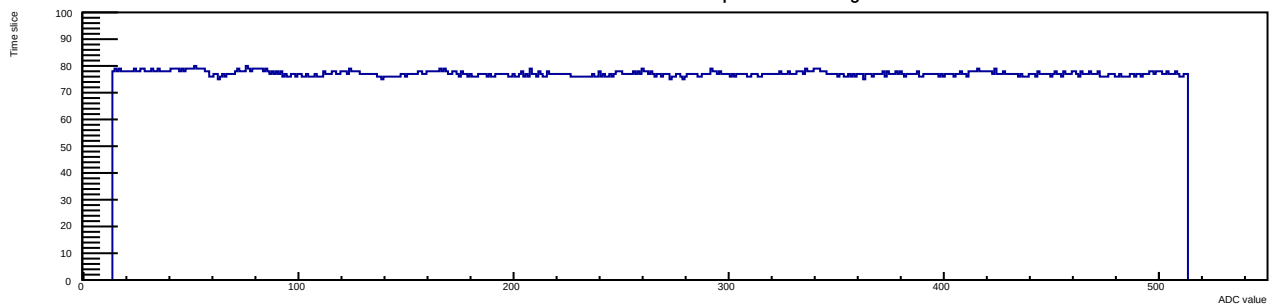
Run 12 Evt 1 Time mcm 1 chip 2 chan 3 30deg
