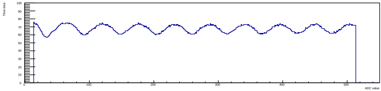
Run 14 Evt 1 Time mcm 1 chip 4 chan 2 50deg
