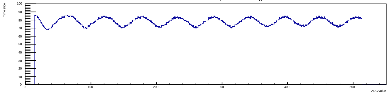
Run 14 Evt 1 Time mcm 1 chip 5 chan 8 50deg
