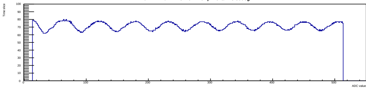
Run 14 Evt 1 Time mcm 1 chip 2 chan 13 50deg
