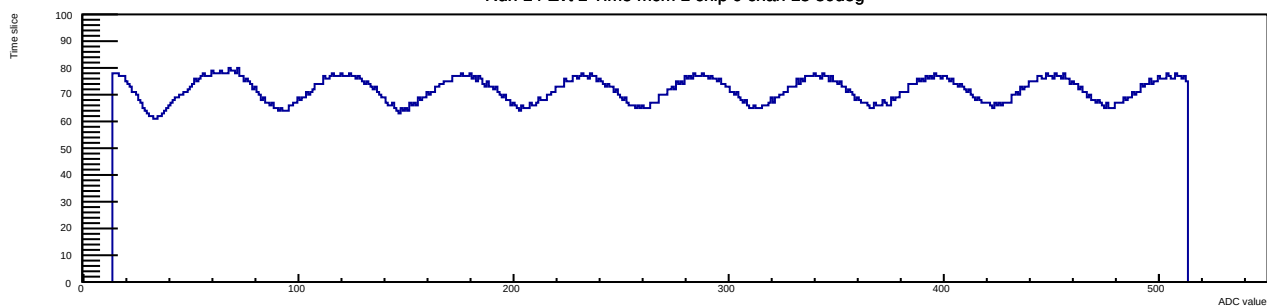
Run 14 Evt 1 Time mcm 1 chip 0 chan 15 50deg
