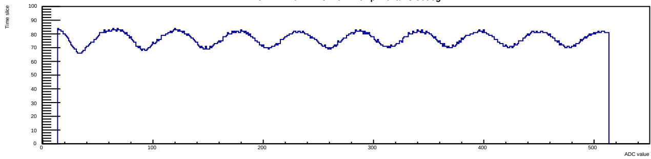
Run 14 Evt 1 Time mcm 1 chip 7 chan 8 50deg
