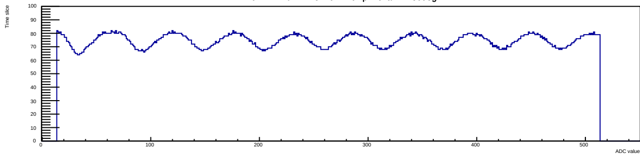
Run 14 Evt 1 Time mcm 1 chip 2 chan 12 50deg
