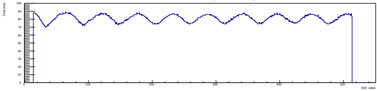
Run 14 Evt 1 Time mcm 1 chip 6 chan 9 50deg
