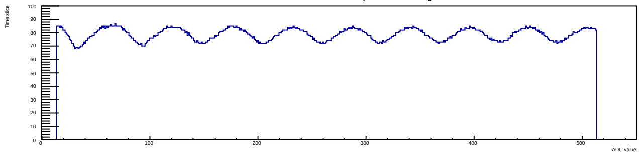
Run 14 Evt 1 Time mcm 1 chip 2 chan 7 50deg
