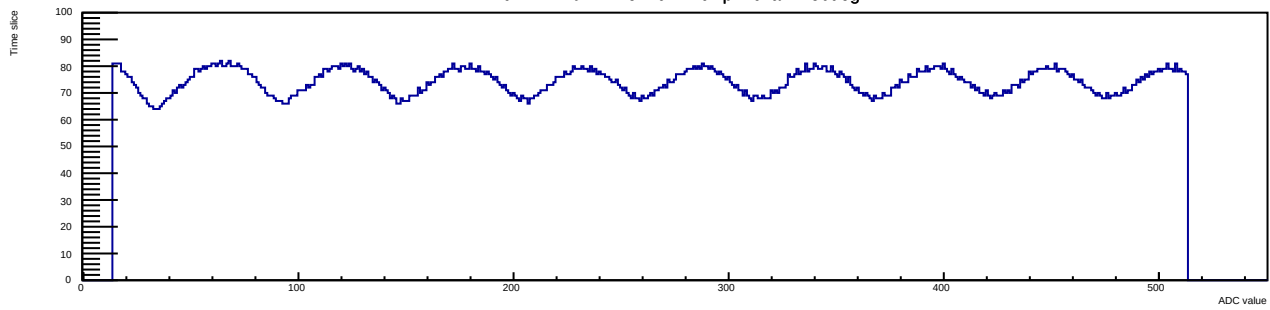
Run 14 Evt 1 Time mcm 1 chip 1 chan 4 50deg
