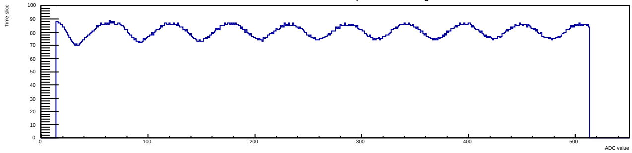
Run 14 Evt 1 Time mcm 1 chip 1 chan 12 50deg
