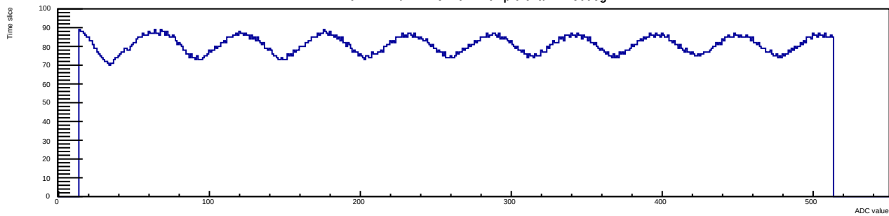
Run 14 Evt 1 Time mcm 1 chip 0 chan 12 50deg
