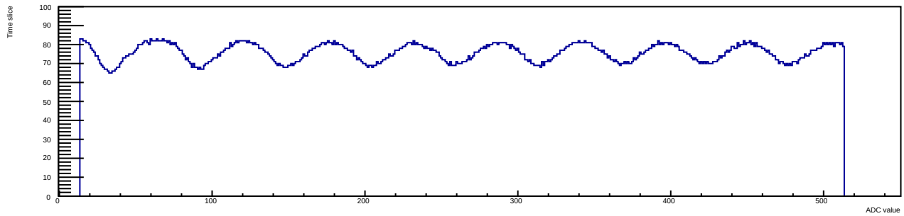
Run 14 Evt 1 Time mcm 1 chip 6 chan 3 50deg
