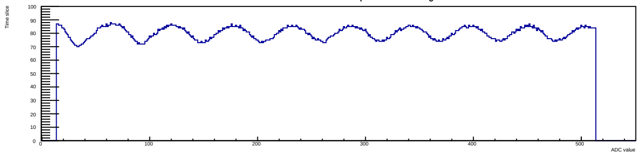
Run 14 Evt 1 Time mcm 1 chip 3 chan 14 50deg
