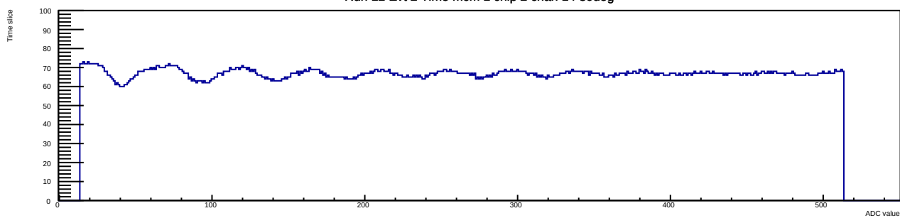
Run 12 Evt 2 Time mcm 1 chip 2 chan 14 30deg
