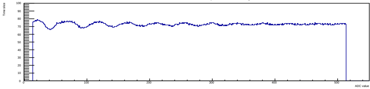
Run 12 Evt 2 Time mcm 1 chip 1 chan 9 30deg
