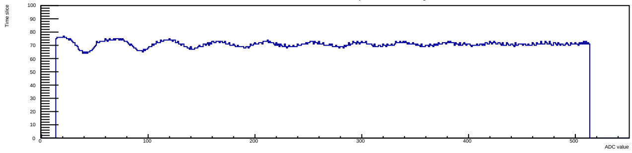
Run 12 Evt 2 Time mcm 1 chip 7 chan 9 30deg
