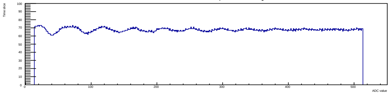
Run 12 Evt 2 Time mcm 1 chip 0 chan 15 30deg
