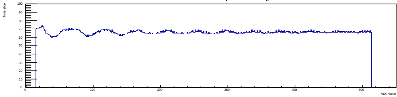
Run 12 Evt 2 Time mcm 1 chip 3 chan 0 30deg
