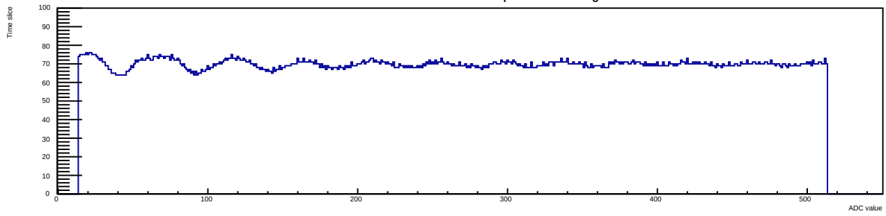
Run 12 Evt 2 Time mcm 1 chip 1 chan 4 30deg
