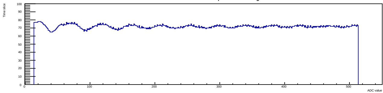
Run 12 Evt 2 Time mcm 1 chip 0 chan 7 30deg
