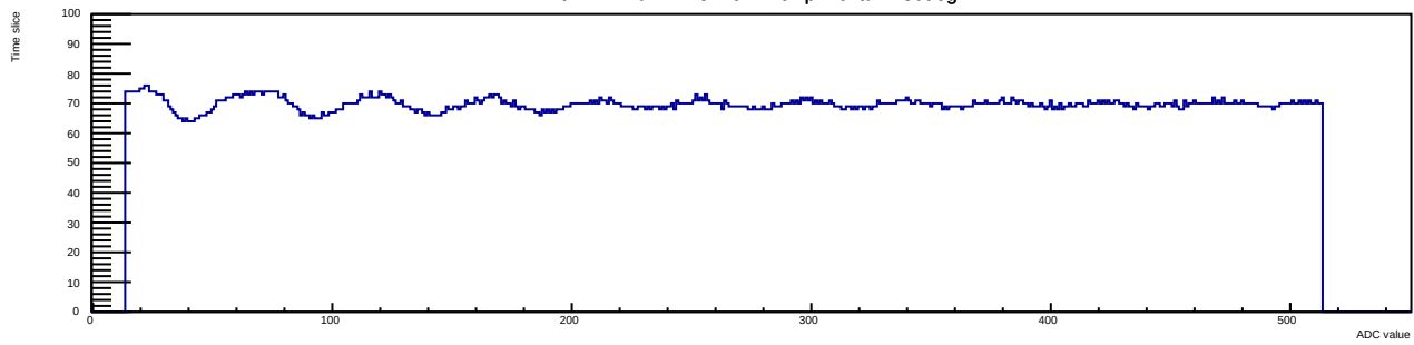
Run 12 Evt 2 Time mcm 1 chip 2 chan 4 30deg
