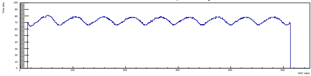
Run 13 Evt 2 Time mcm 1 chip 2 chan 4 40deg
