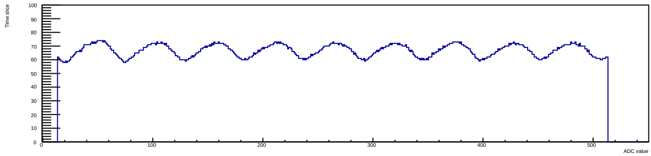
Run 13 Evt 2 Time mcm 1 chip 4 chan 2 40deg
