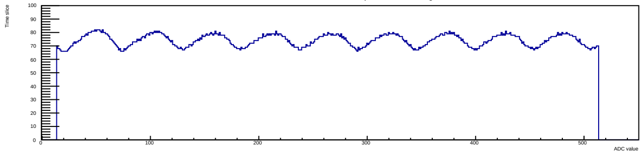
Run 13 Evt 2 Time mcm 1 chip 7 chan 9 40deg
