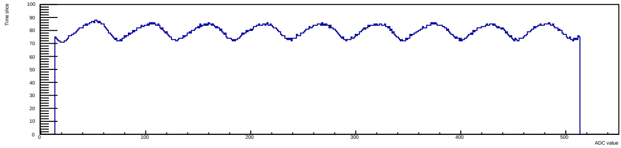
Run 13 Evt 2 Time mcm 1 chip 6 chan 9 40deg
