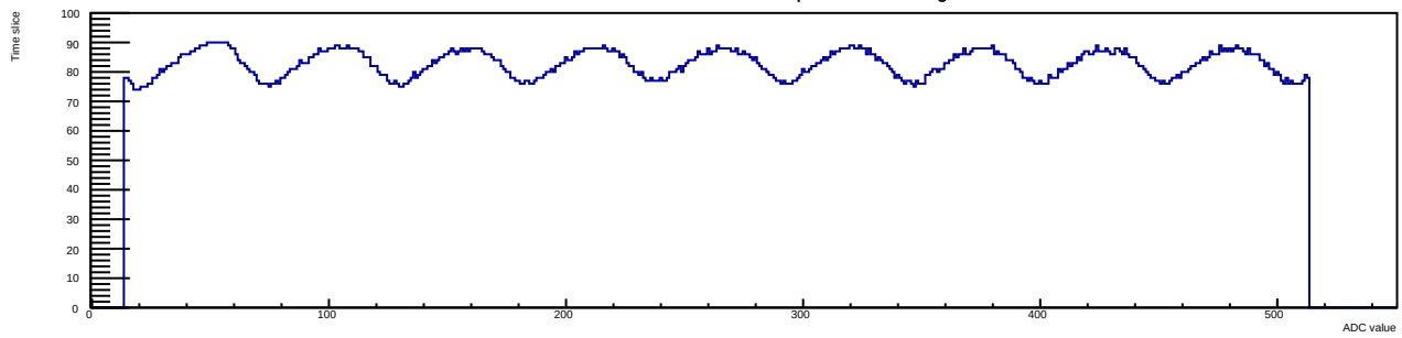
Run 13 Evt 2 Time mcm 1 chip 1 chan 6 40deg
