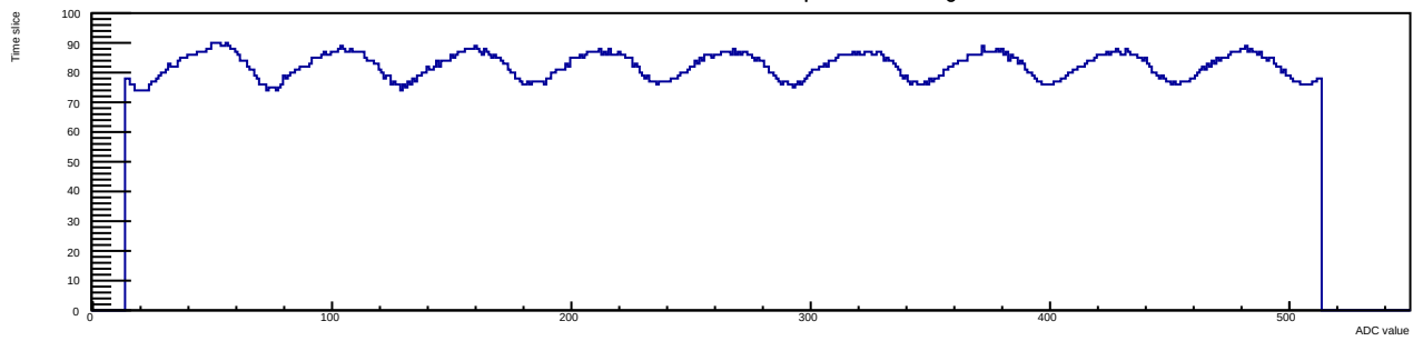
Run 13 Evt 2 Time mcm 1 chip 2 chan 2 40deg
