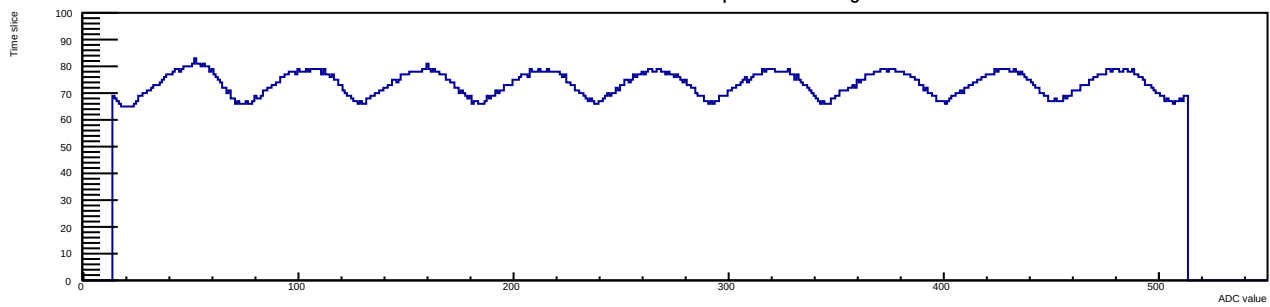
Run 13 Evt 2 Time mcm 1 chip 6 chan 6 40deg
