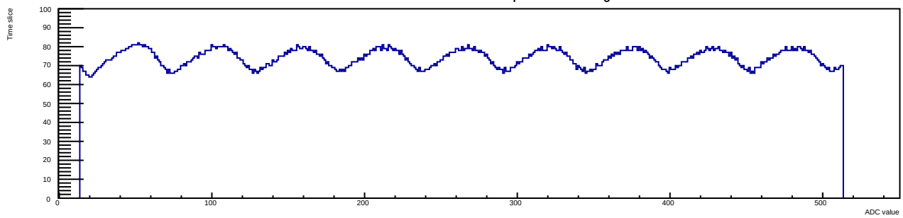
Run 13 Evt 2 Time mcm 1 chip 0 chan 7 40deg
