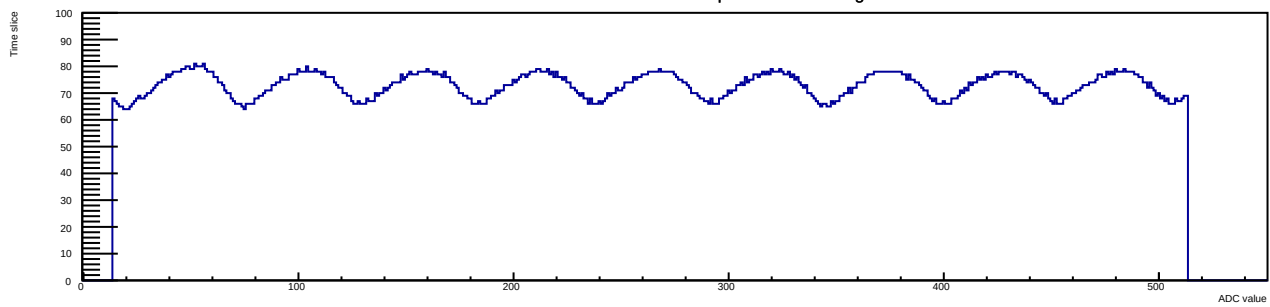
Run 13 Evt 2 Time mcm 1 chip 1 chan 14 40deg
