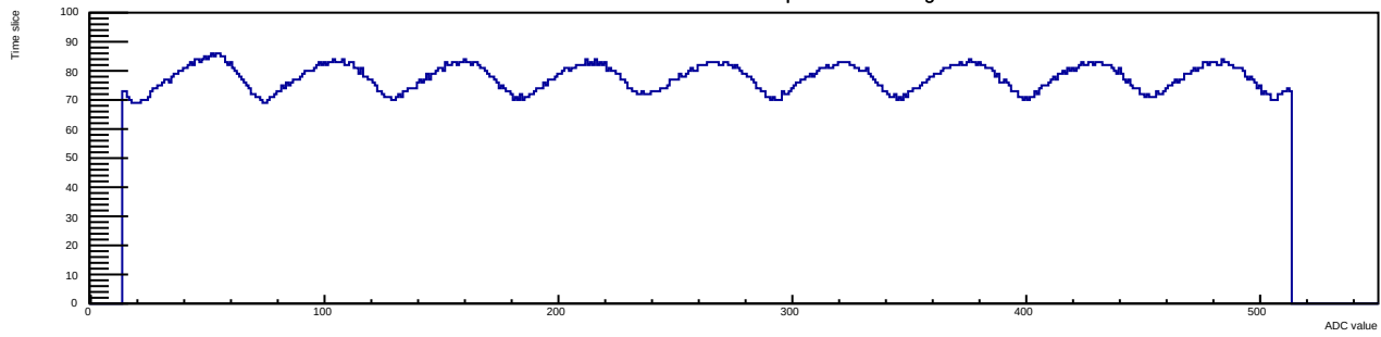
Run 13 Evt 2 Time mcm 1 chip 4 chan 4 40deg
