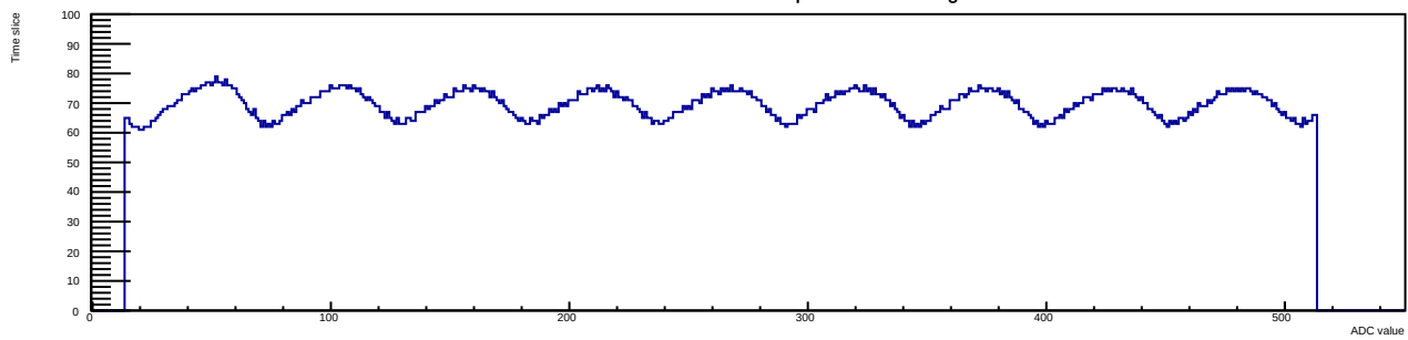
Run 13 Evt 2 Time mcm 1 chip 0 chan 14 40deg
