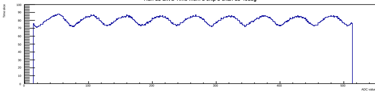
Run 13 Evt 2 Time mcm 1 chip 5 chan 15 40deg
