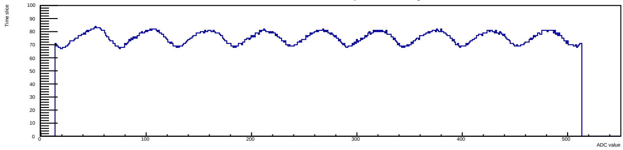
Run 13 Evt 2 Time mcm 1 chip 1 chan 5 40deg
