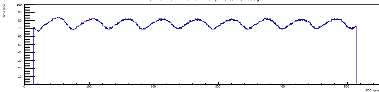
Run 13 Evt 2 Time mcm 1 chip 2 chan 15 40deg
