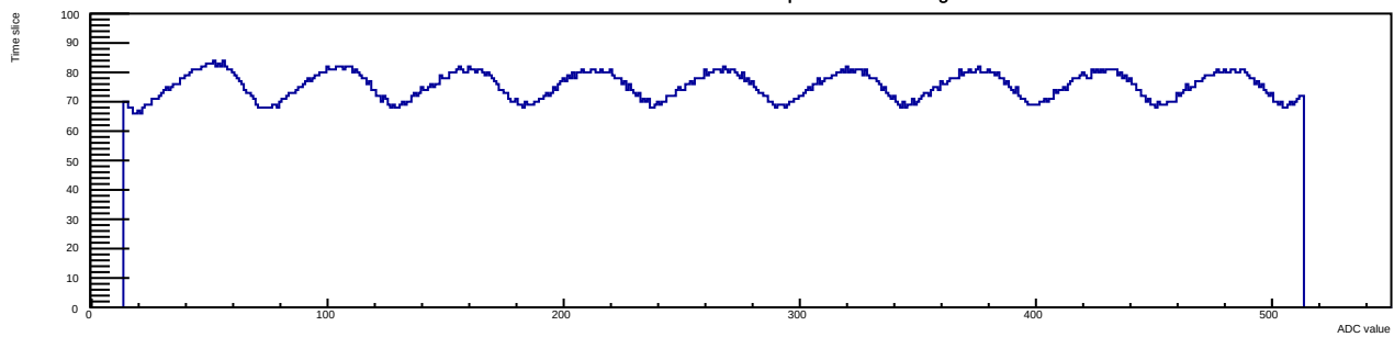
Run 13 Evt 2 Time mcm 1 chip 1 chan 15 40deg
