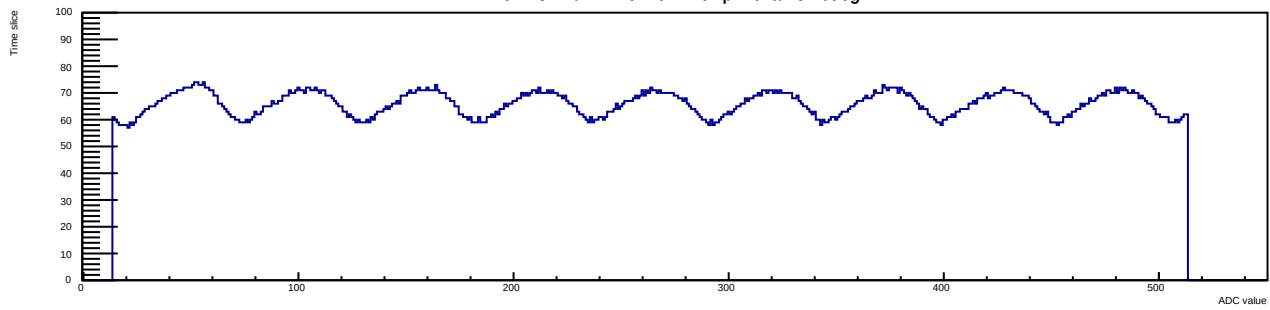
Run 13 Evt 2 Time mcm 1 chip 2 chan 8 40deg
