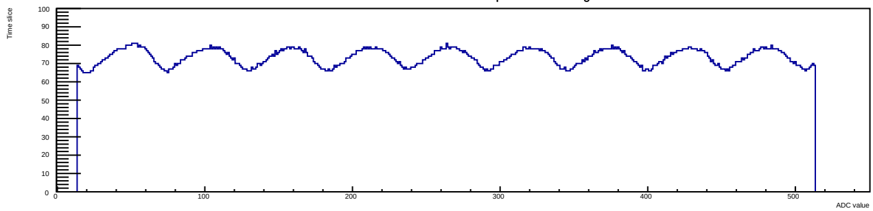
Run 13 Evt 2 Time mcm 1 chip 3 chan 7 40deg
