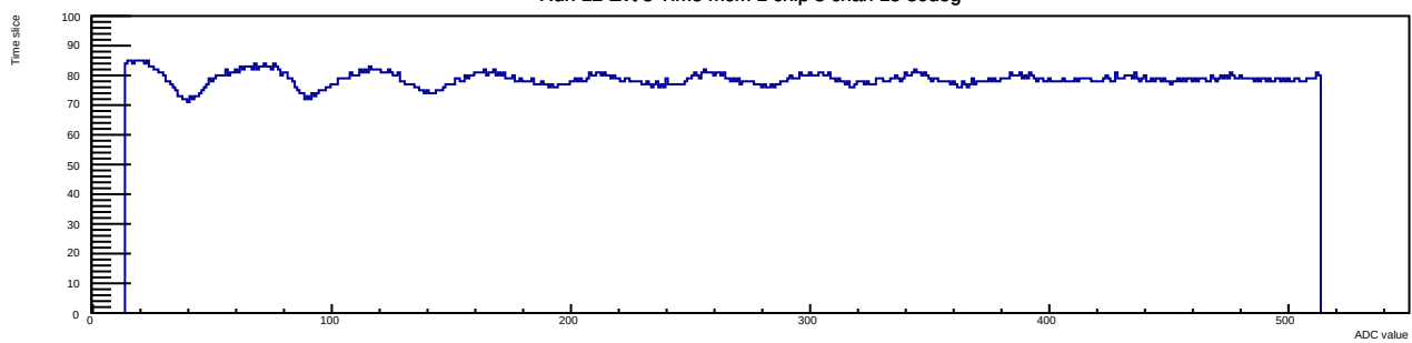
Run 12 Evt 3 Time mcm 1 chip 3 chan 15 30deg
