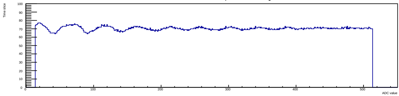
Run 12 Evt 3 Time mcm 1 chip 2 chan 10 30deg
