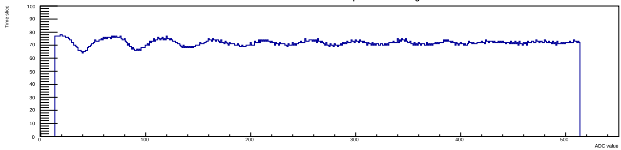
Run 12 Evt 3 Time mcm 1 chip 0 chan 7 30deg
