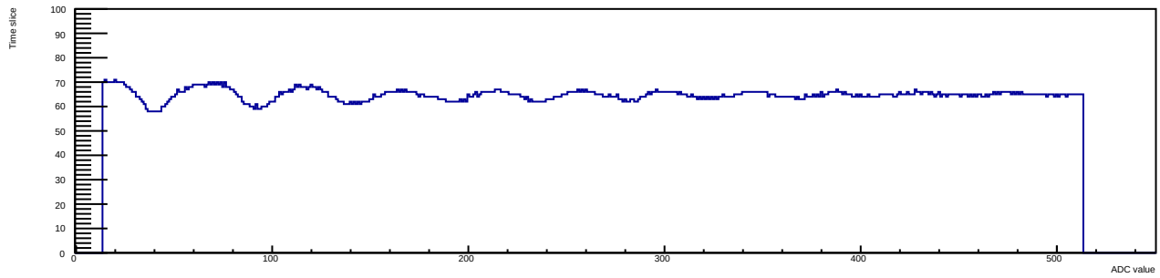
Run 12 Evt 3 Time mcm 1 chip 4 chan 6 30deg
