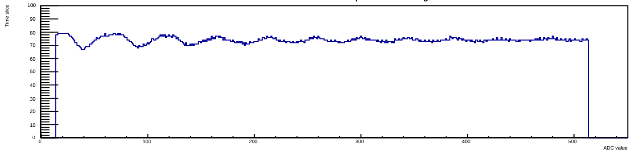
Run 12 Evt 3 Time mcm 1 chip 7 chan 12 30deg
