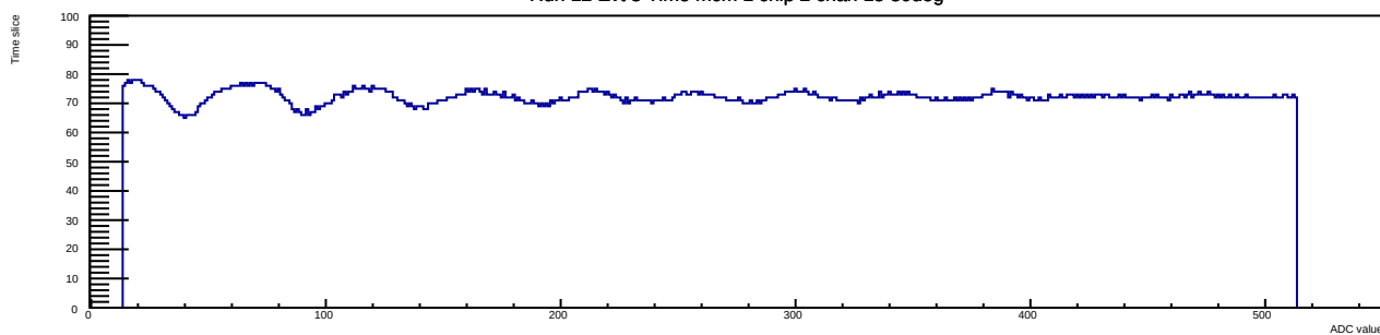
Run 12 Evt 3 Time mcm 1 chip 2 chan 15 30deg
