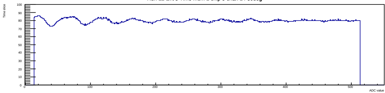
Run 12 Evt 3 Time mcm 1 chip 5 chan 14 30deg
