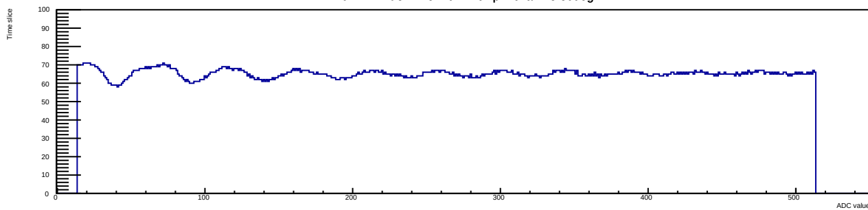
Run 12 Evt 3 Time mcm 1 chip 2 chan 13 30deg
