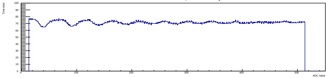
Run 12 Evt 3 Time mcm 1 chip 0 chan 9 30deg
