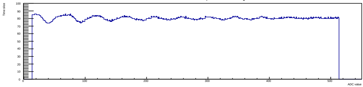
Run 12 Evt 3 Time mcm 1 chip 1 chan 6 30deg
