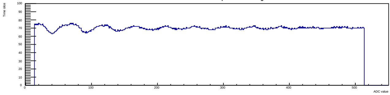
Run 12 Evt 3 Time mcm 1 chip 5 chan 8 30deg
