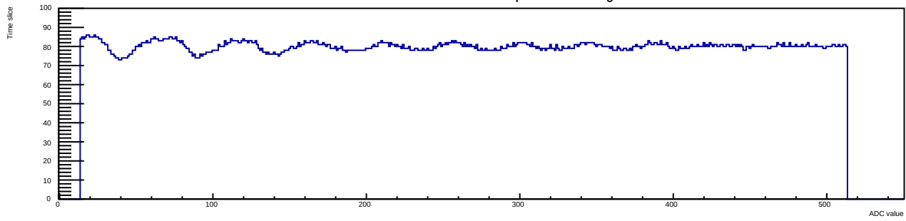
Run 12 Evt 3 Time mcm 1 chip 3 chan 4 30deg
