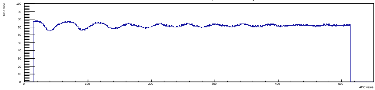
Run 12 Evt 3 Time mcm 1 chip 6 chan 10 30deg
