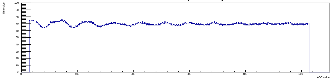
Run 12 Evt 3 Time mcm 1 chip 1 chan 4 30deg
