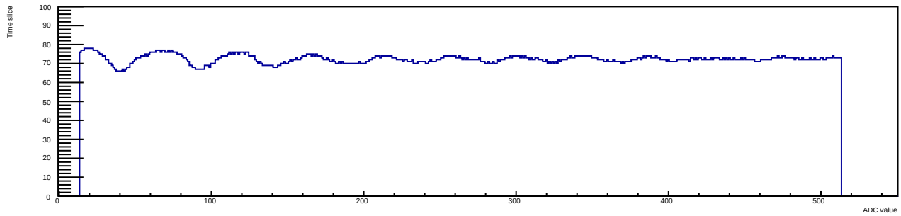
Run 12 Evt 3 Time mcm 1 chip 4 chan 7 30deg
