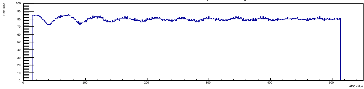
Run 12 Evt 3 Time mcm 1 chip 5 chan 0 30deg
