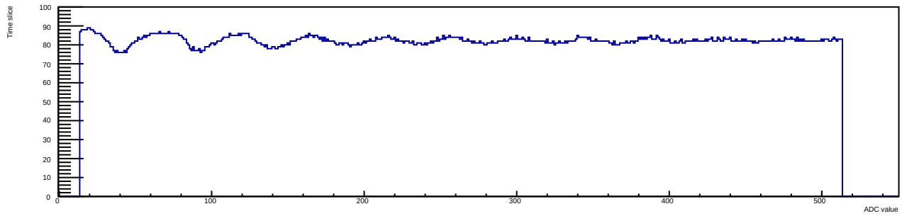
Run 12 Evt 3 Time mcm 1 chip 5 chan 10 30deg
