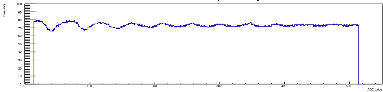
Run 12 Evt 3 Time mcm 1 chip 5 chan 2 30deg
