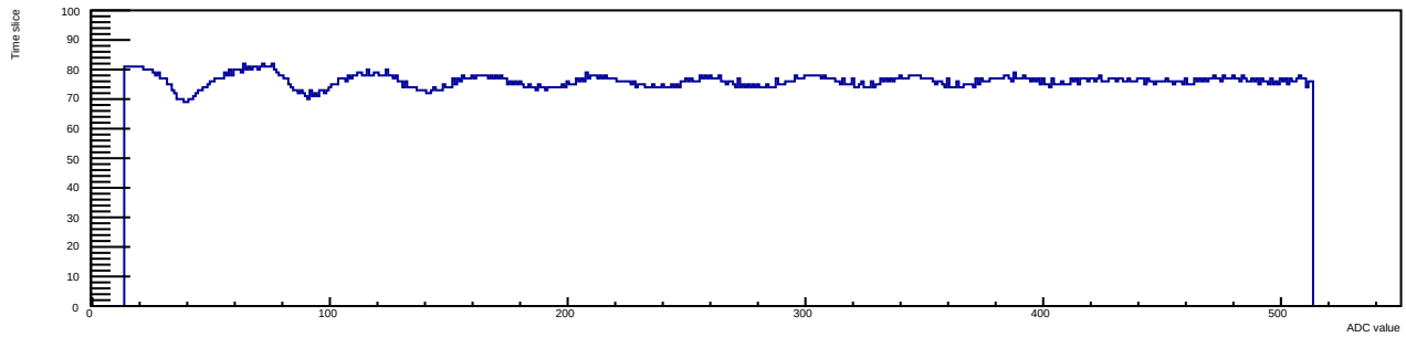
Run 12 Evt 3 Time mcm 1 chip 3 chan 3 30deg
