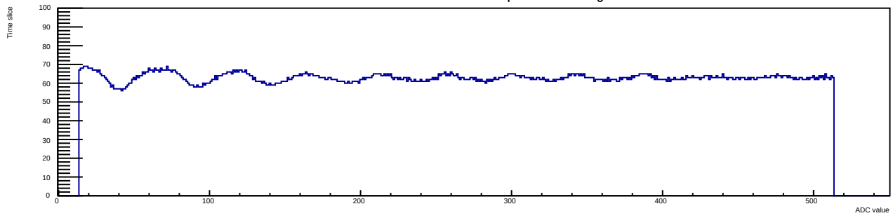
Run 12 Evt 3 Time mcm 1 chip 2 chan 8 30deg
