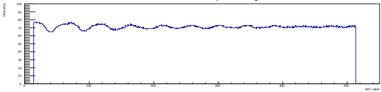
Run 12 Evt 3 Time mcm 1 chip 6 chan 6 30deg
