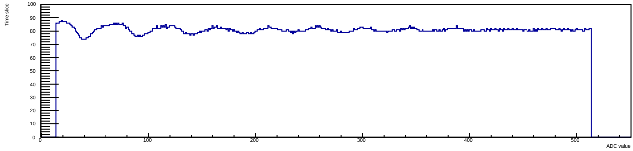
Run 12 Evt 3 Time mcm 1 chip 6 chan 13 30deg
