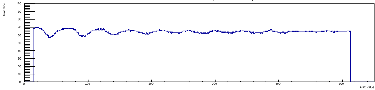
Run 12 Evt 3 Time mcm 1 chip 2 chan 5 30deg
