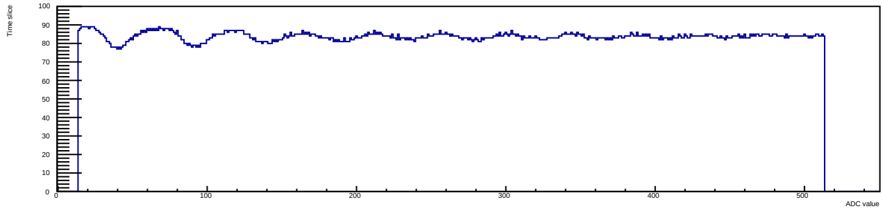
Run 12 Evt 3 Time mcm 1 chip 3 chan 9 30deg
