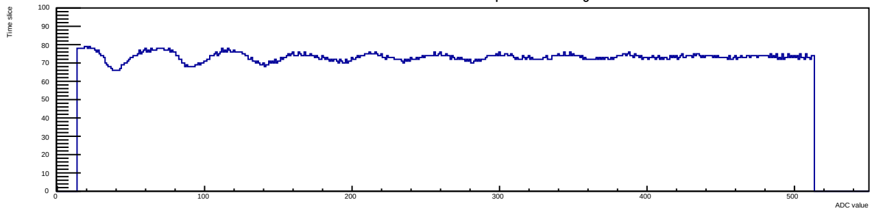
Run 12 Evt 3 Time mcm 1 chip 3 chan 8 30deg
