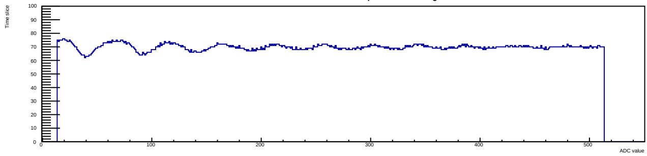
Run 12 Evt 3 Time mcm 1 chip 6 chan 5 30deg
