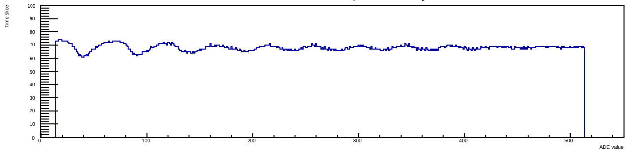
Run 12 Evt 3 Time mcm 1 chip 6 chan 11 30deg
