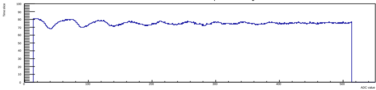
Run 12 Evt 3 Time mcm 1 chip 2 chan 6 30deg
