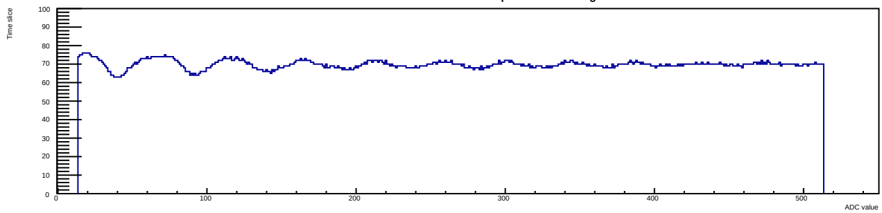
Run 12 Evt 3 Time mcm 1 chip 6 chan 7 30deg
