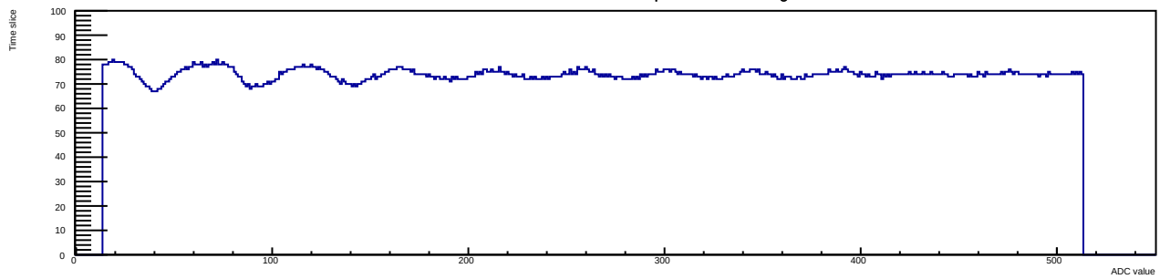
Run 12 Evt 3 Time mcm 1 chip 6 chan 14 30deg
