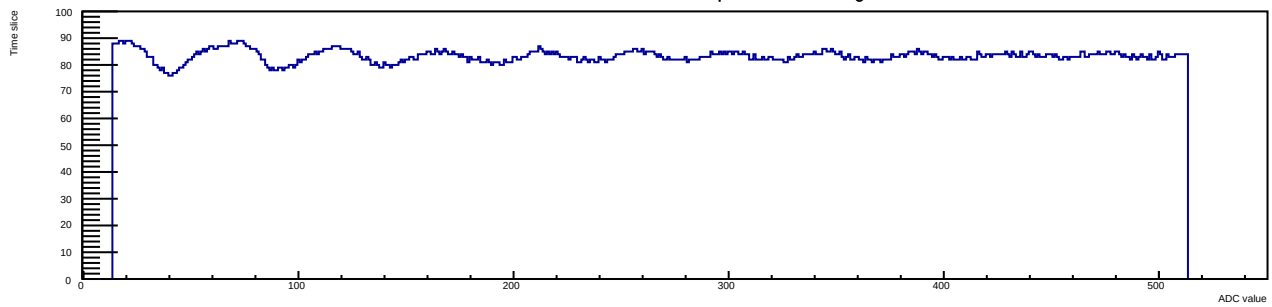
Run 12 Evt 3 Time mcm 1 chip 7 chan 15 30deg
