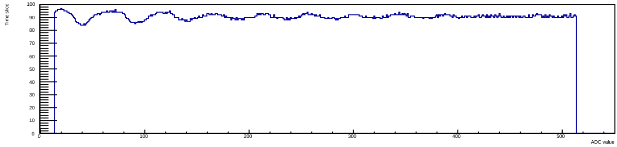
Run 12 Evt 3 Time mcm 1 chip 3 chan 1 30deg
