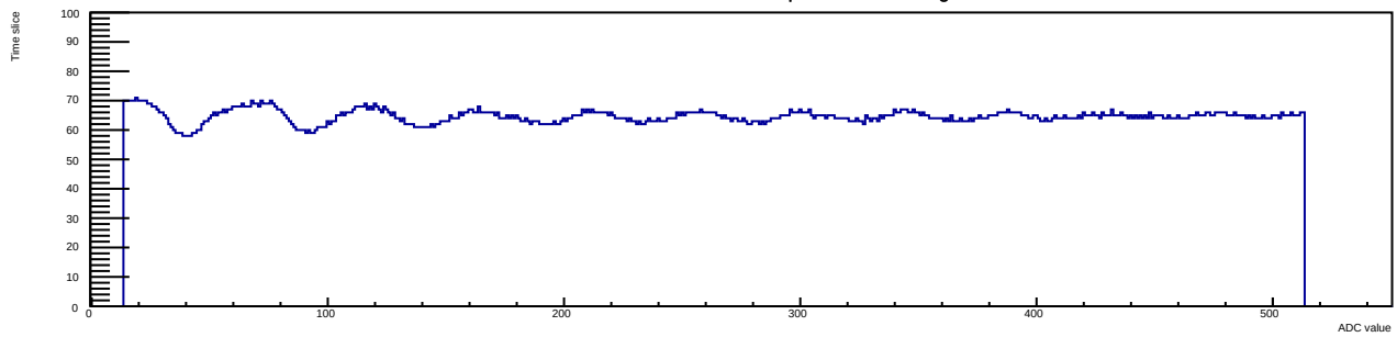
Run 12 Evt 3 Time mcm 1 chip 1 chan 11 30deg
