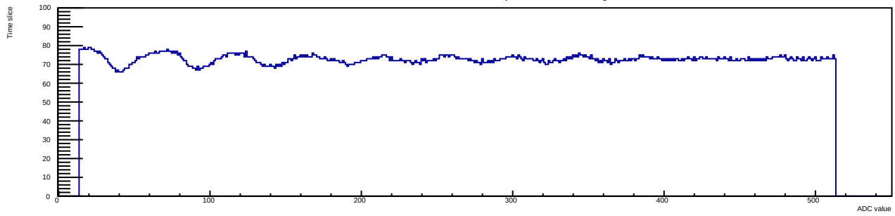
Run 12 Evt 3 Time mcm 1 chip 7 chan 13 30deg
