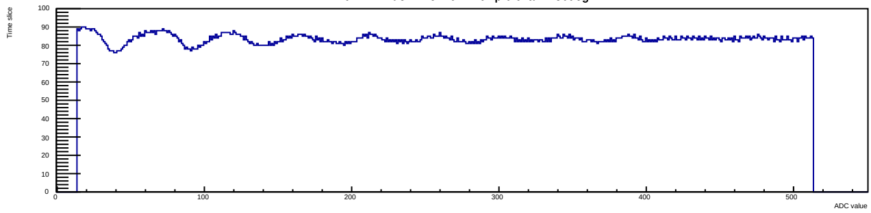
Run 12 Evt 3 Time mcm 1 chip 0 chan 4 30deg
