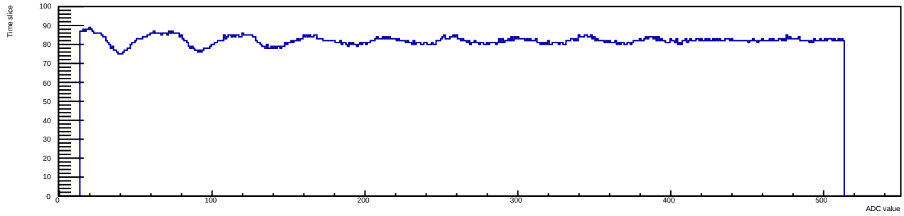
Run 12 Evt 3 Time mcm 1 chip 4 chan 5 30deg
