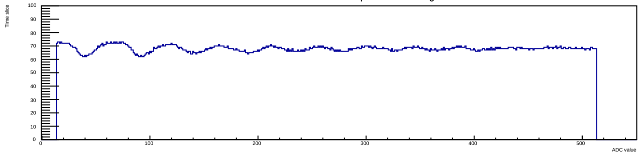
Run 12 Evt 3 Time mcm 1 chip 6 chan 12 30deg
