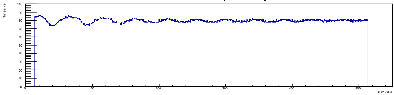
Run 12 Evt 3 Time mcm 1 chip 0 chan 6 30deg
