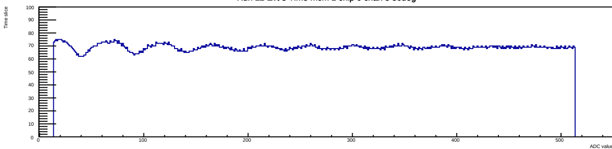
Run 12 Evt 3 Time mcm 1 chip 0 chan 3 30deg
