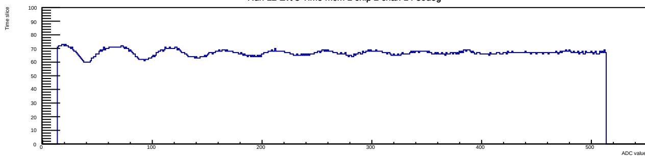
Run 12 Evt 3 Time mcm 1 chip 2 chan 14 30deg
