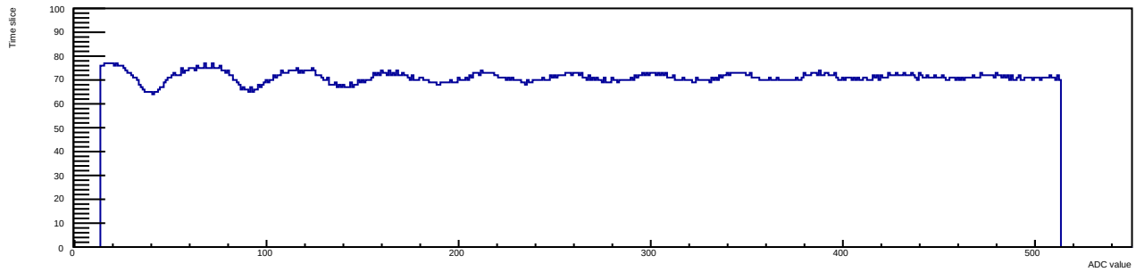
Run 12 Evt 3 Time mcm 1 chip 6 chan 3 30deg
