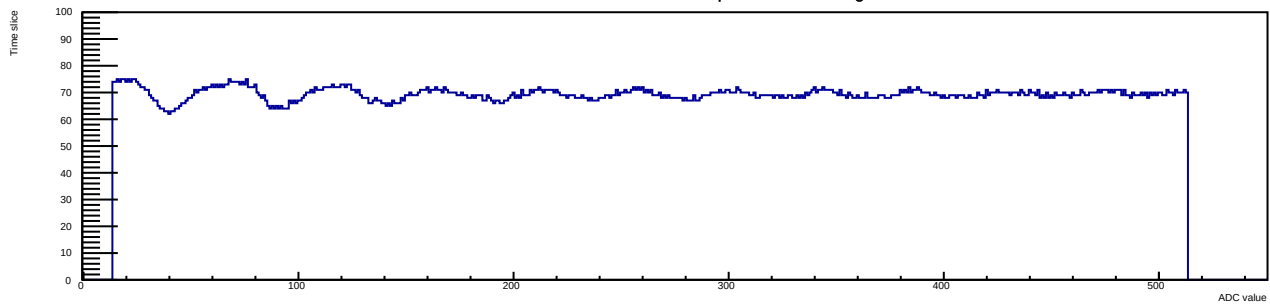
Run 12 Evt 3 Time mcm 1 chip 1 chan 13 30deg
