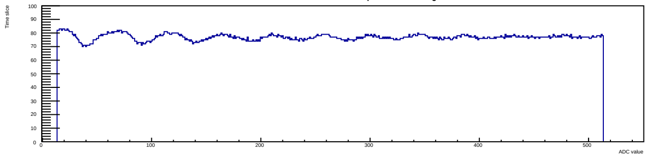
Run 12 Evt 3 Time mcm 1 chip 2 chan 3 30deg
