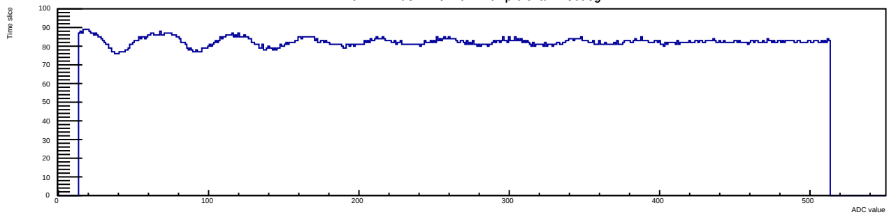
Run 12 Evt 3 Time mcm 1 chip 6 chan 4 30deg
