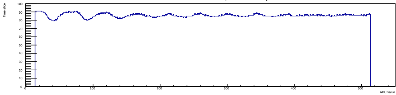
Run 12 Evt 3 Time mcm 1 chip 7 chan 6 30deg
