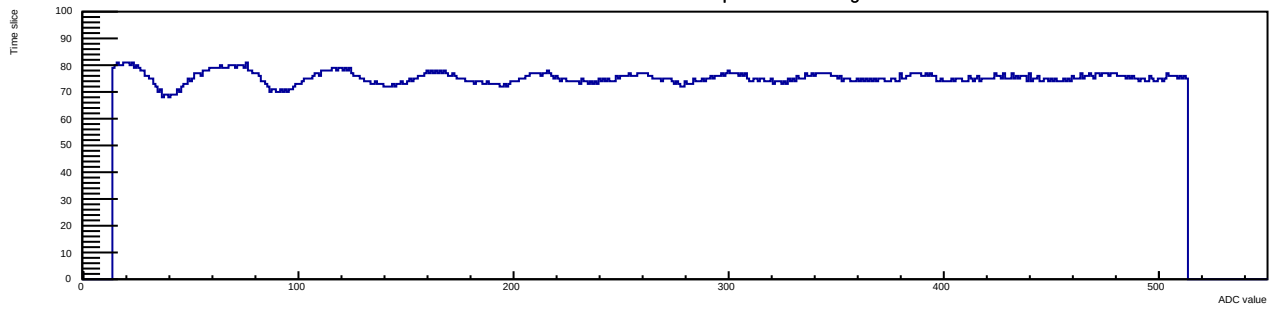
Run 12 Evt 3 Time mcm 1 chip 4 chan 4 30deg
