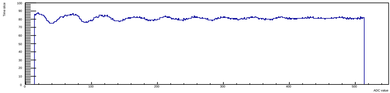
Run 12 Evt 3 Time mcm 1 chip 5 chan 11 30deg
