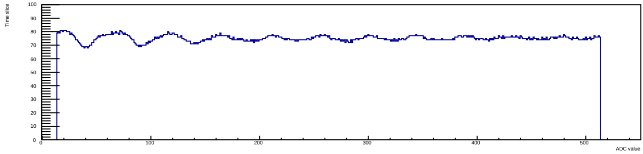
Run 12 Evt 3 Time mcm 1 chip 5 chan 9 30deg
