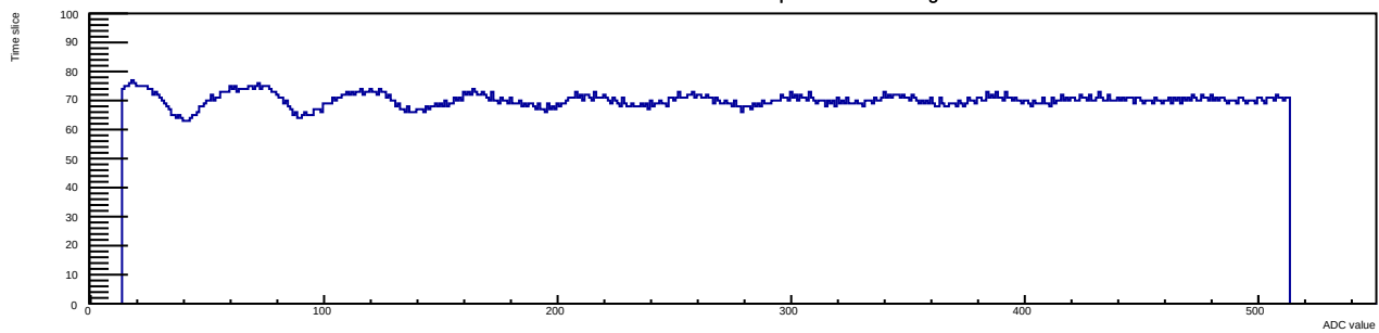
Run 12 Evt 3 Time mcm 1 chip 0 chan 11 30deg
