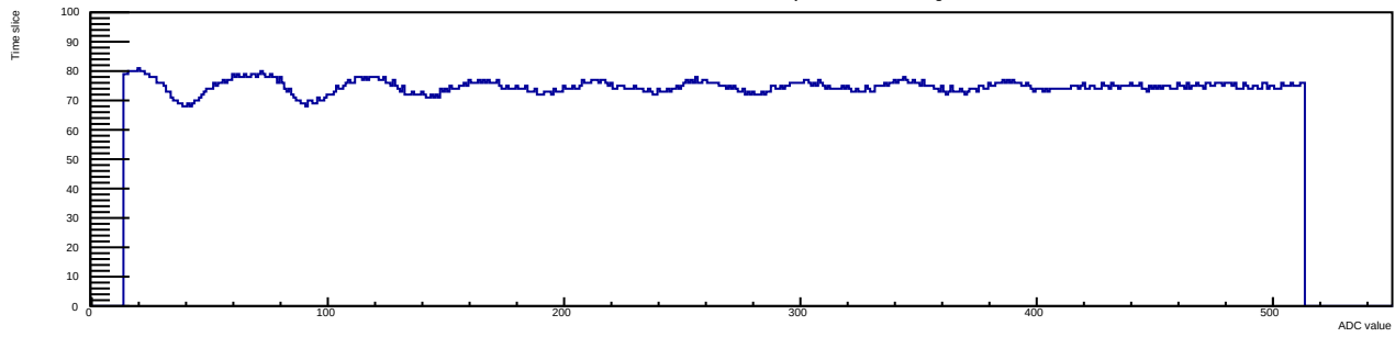
Run 12 Evt 3 Time mcm 1 chip 7 chan 5 30deg
