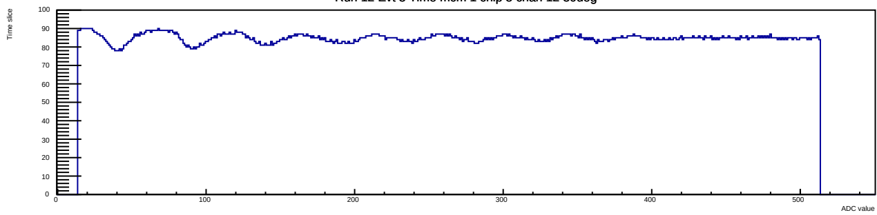
Run 12 Evt 3 Time mcm 1 chip 5 chan 12 30deg
