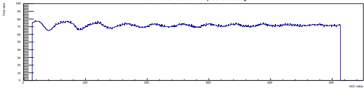
Run 12 Evt 3 Time mcm 1 chip 0 chan 8 30deg
