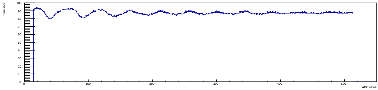
Run 12 Evt 3 Time mcm 1 chip 6 chan 2 30deg
