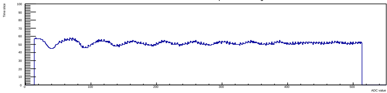
Run 12 Evt 3 Time mcm 1 chip 0 chan 10 30deg
