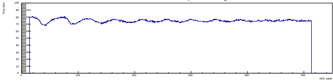
Run 12 Evt 3 Time mcm 1 chip 4 chan 12 30deg
