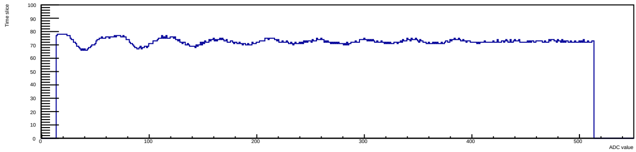
Run 12 Evt 3 Time mcm 1 chip 3 chan 10 30deg
