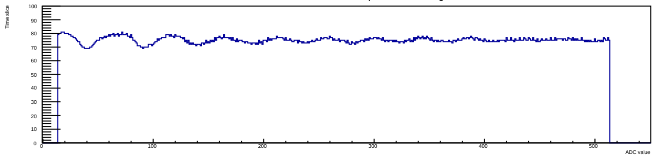
Run 12 Evt 3 Time mcm 1 chip 1 chan 10 30deg
