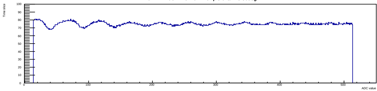
Run 12 Evt 3 Time mcm 1 chip 3 chan 13 30deg
