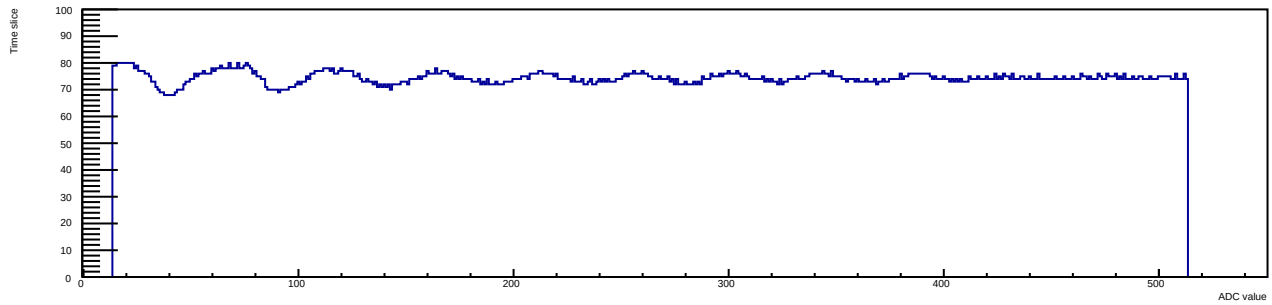
Run 12 Evt 3 Time mcm 1 chip 3 chan 11 30deg
