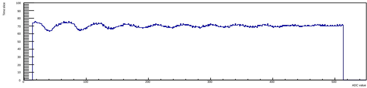
Run 12 Evt 3 Time mcm 1 chip 1 chan 2 30deg
