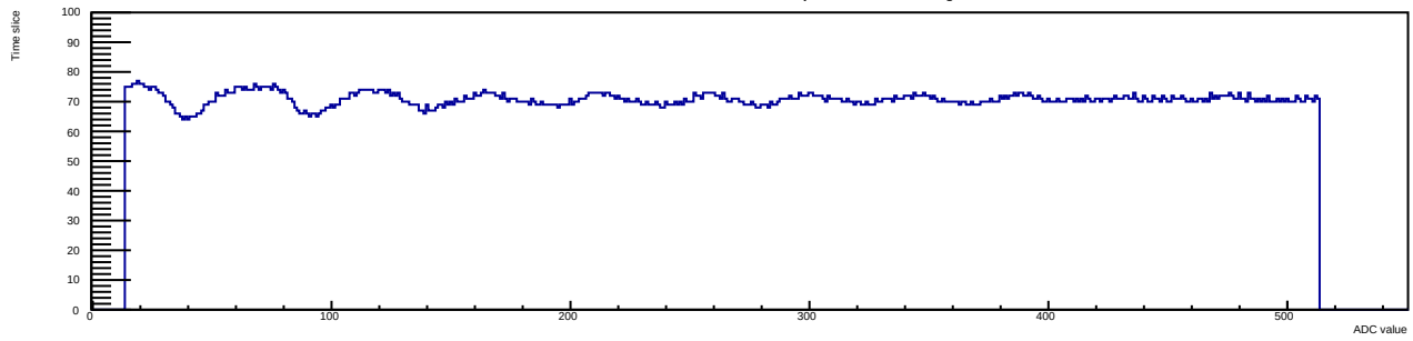
Run 12 Evt 3 Time mcm 1 chip 7 chan 9 30deg
