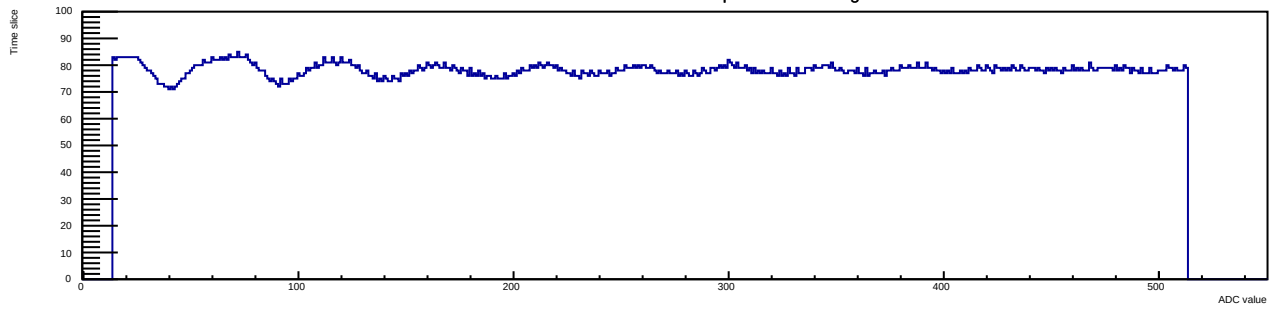
Run 12 Evt 3 Time mcm 1 chip 1 chan 0 30deg
