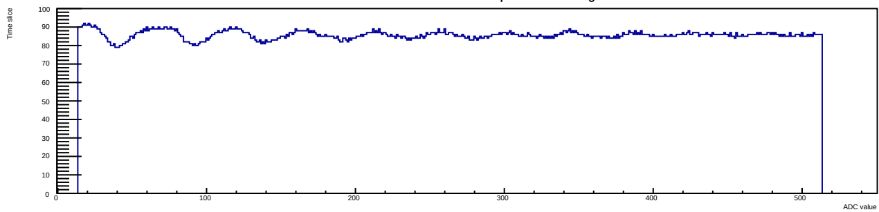
Run 12 Evt 3 Time mcm 1 chip 5 chan 3 30deg
