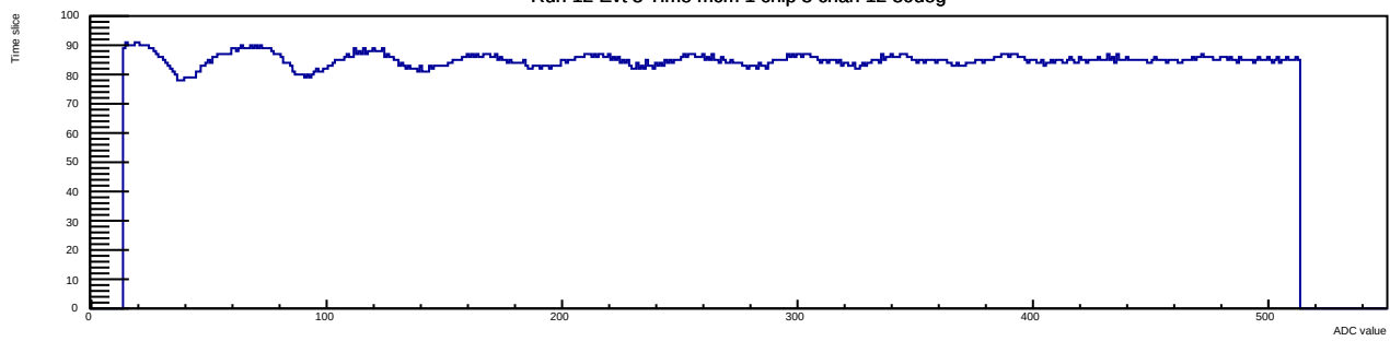
Run 12 Evt 3 Time mcm 1 chip 3 chan 12 30deg
