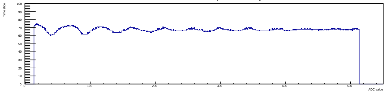
Run 12 Evt 3 Time mcm 1 chip 4 chan 14 30deg
