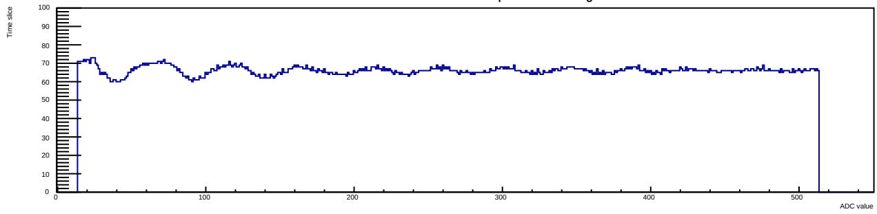
Run 12 Evt 3 Time mcm 1 chip 3 chan 0 30deg
