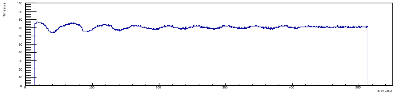
Run 12 Evt 3 Time mcm 1 chip 5 chan 6 30deg
