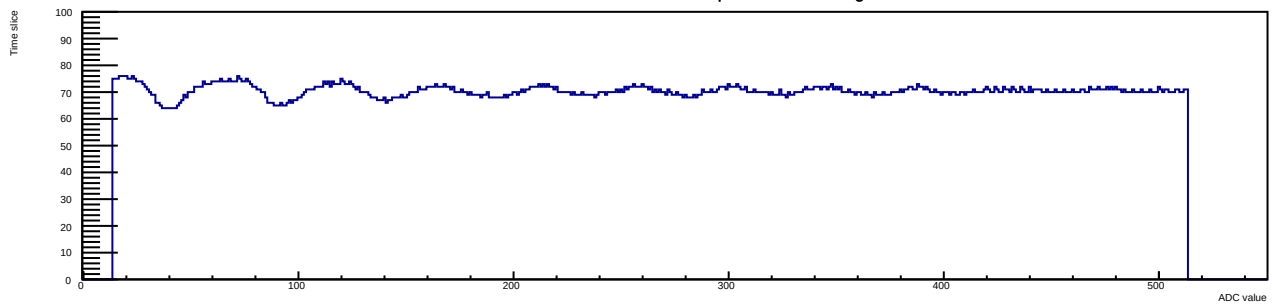
Run 12 Evt 3 Time mcm 1 chip 7 chan 10 30deg
