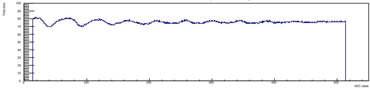
Run 12 Evt 3 Time mcm 1 chip 6 chan 9 30deg
