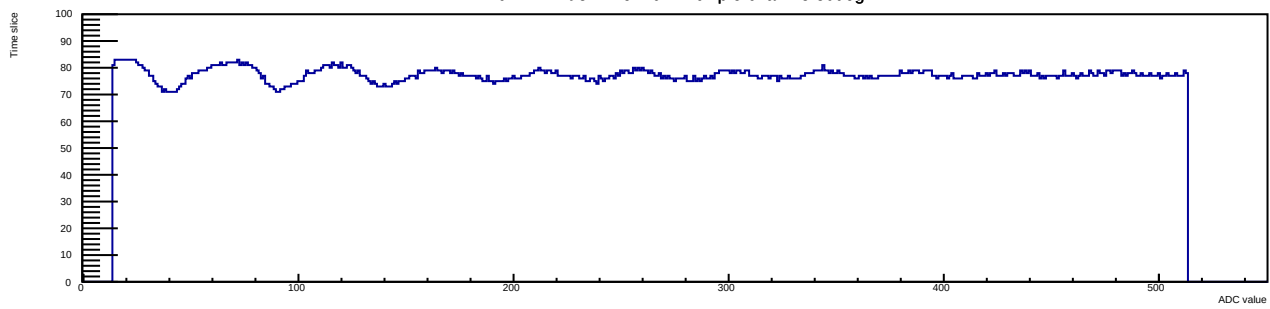
Run 12 Evt 3 Time mcm 1 chip 5 chan 13 30deg
