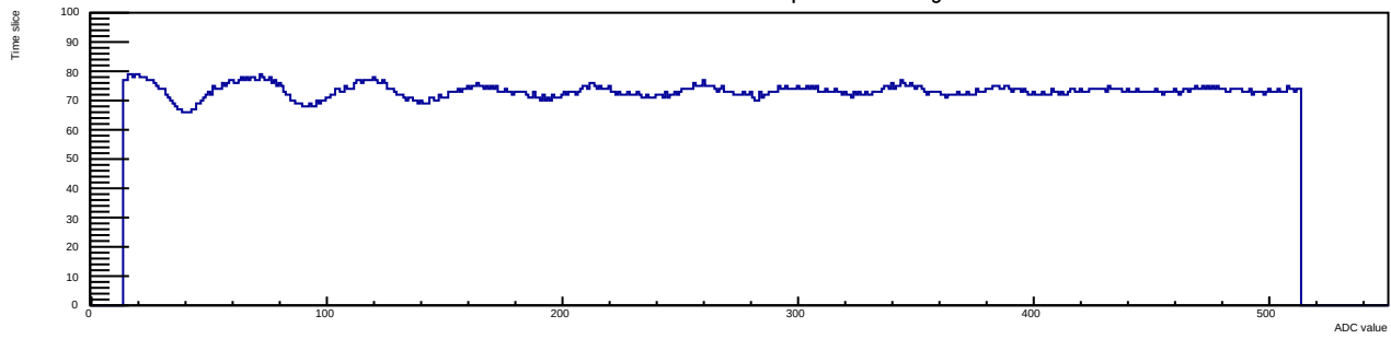
Run 12 Evt 3 Time mcm 1 chip 7 chan 4 30deg
