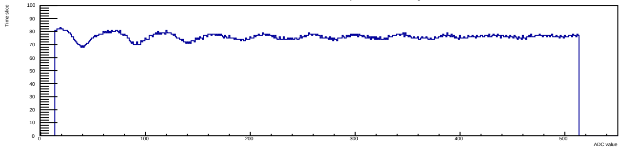
Run 12 Evt 3 Time mcm 1 chip 0 chan 13 30deg
