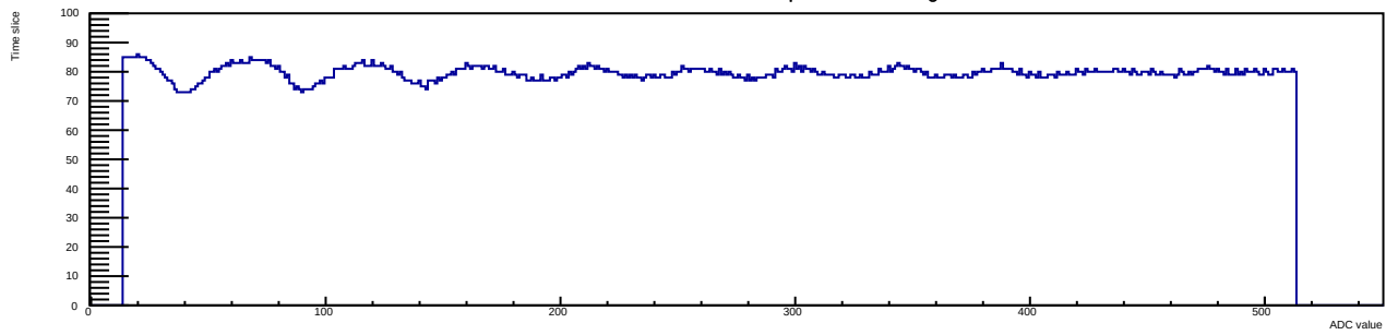
Run 12 Evt 3 Time mcm 1 chip 7 chan 1 30deg
