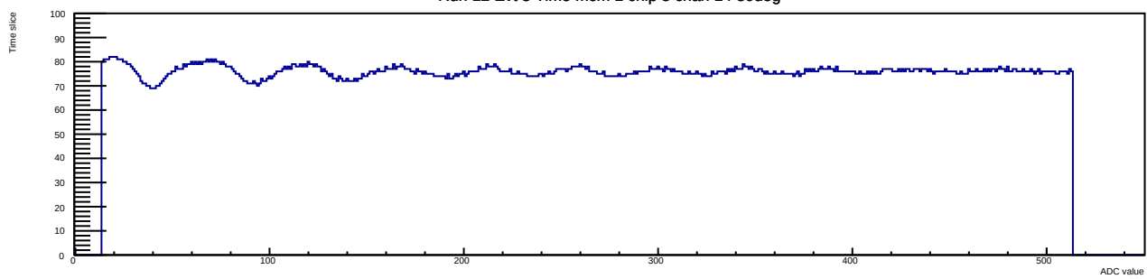
Run 12 Evt 3 Time mcm 1 chip 3 chan 14 30deg
