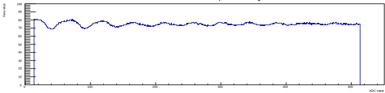
Run 12 Evt 3 Time mcm 1 chip 2 chan 7 30deg
