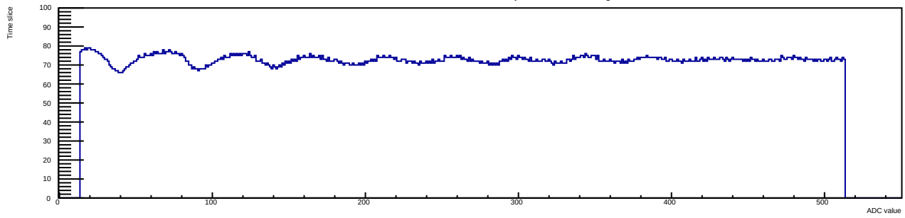
Run 12 Evt 3 Time mcm 1 chip 1 chan 9 30deg
