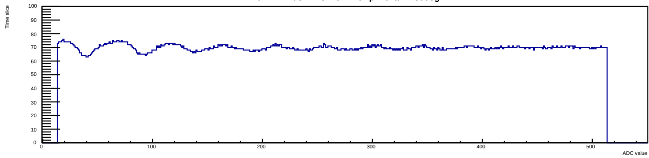
Run 12 Evt 3 Time mcm 1 chip 2 chan 4 30deg
