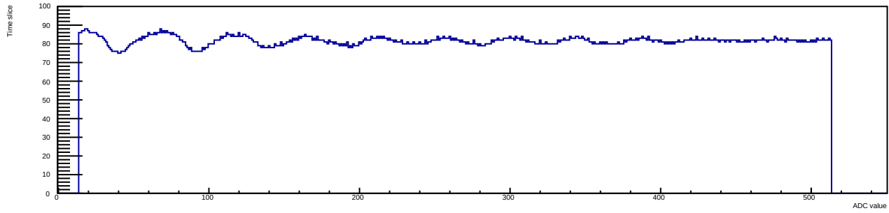
Run 12 Evt 3 Time mcm 1 chip 1 chan 1 30deg
