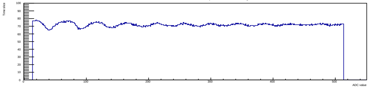
Run 12 Evt 3 Time mcm 1 chip 1 chan 5 30deg
