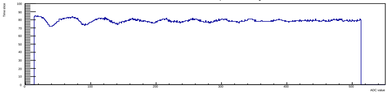
Run 12 Evt 3 Time mcm 1 chip 2 chan 2 30deg
