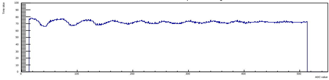
Run 12 Evt 3 Time mcm 1 chip 6 chan 8 30deg
