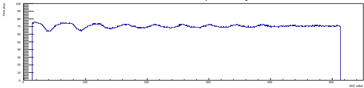
Run 12 Evt 3 Time mcm 1 chip 4 chan 11 30deg
