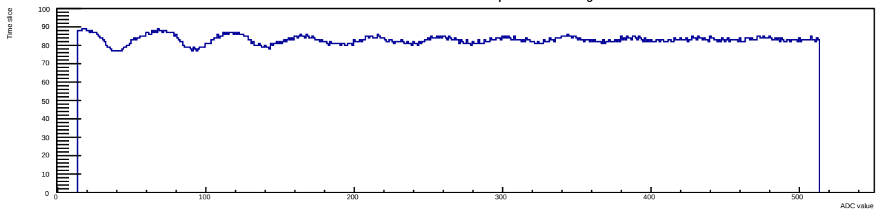
Run 12 Evt 3 Time mcm 1 chip 7 chan 3 30deg
