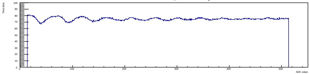
Run 12 Evt 3 Time mcm 1 chip 2 chan 11 30deg
