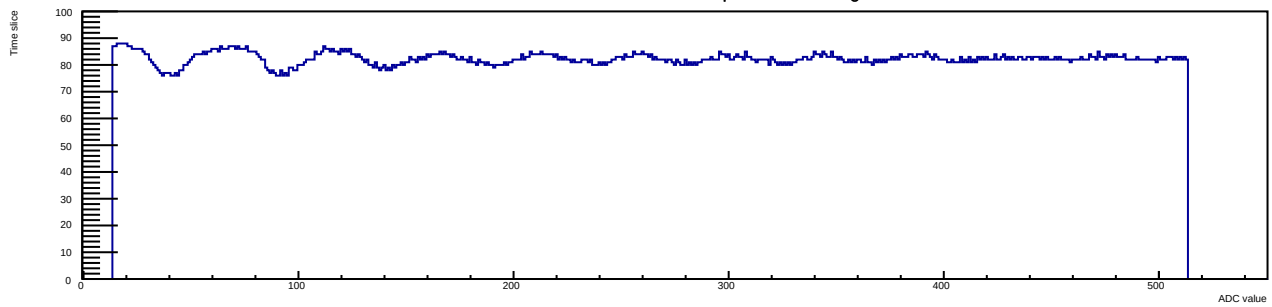
Run 12 Evt 3 Time mcm 1 chip 1 chan 7 30deg
