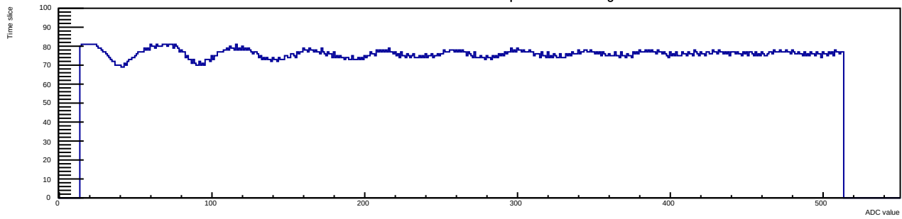
Run 12 Evt 3 Time mcm 1 chip 0 chan 12 30deg
