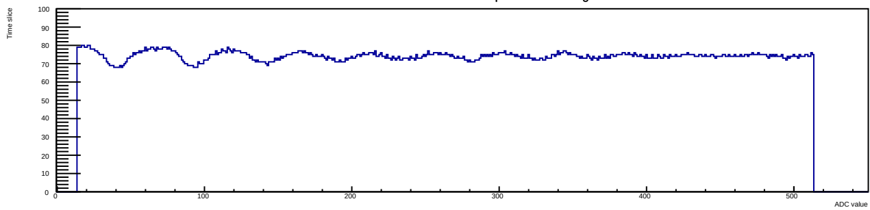
Run 12 Evt 3 Time mcm 1 chip 7 chan 2 30deg
