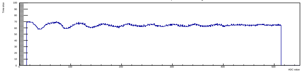
Run 12 Evt 3 Time mcm 1 chip 0 chan 5 30deg
