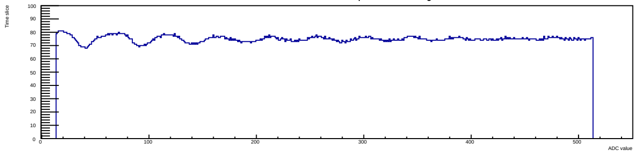
Run 12 Evt 3 Time mcm 1 chip 6 chan 15 30deg
