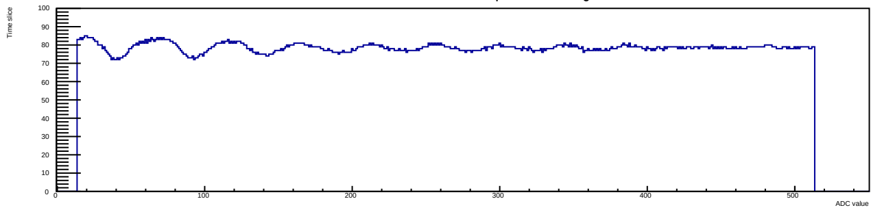
Run 12 Evt 3 Time mcm 1 chip 4 chan 9 30deg
