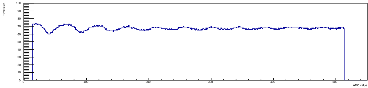
Run 12 Evt 3 Time mcm 1 chip 4 chan 13 30deg
