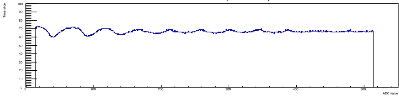
Run 12 Evt 3 Time mcm 1 chip 4 chan 3 30deg
