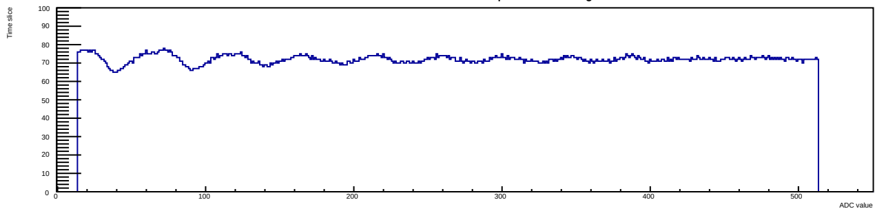
Run 12 Evt 3 Time mcm 1 chip 7 chan 7 30deg
