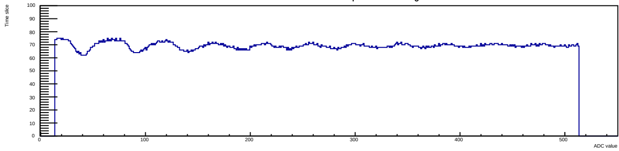
Run 12 Evt 3 Time mcm 1 chip 4 chan 0 30deg
