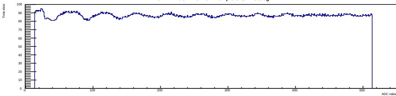
Run 12 Evt 3 Time mcm 1 chip 0 chan 1 30deg
