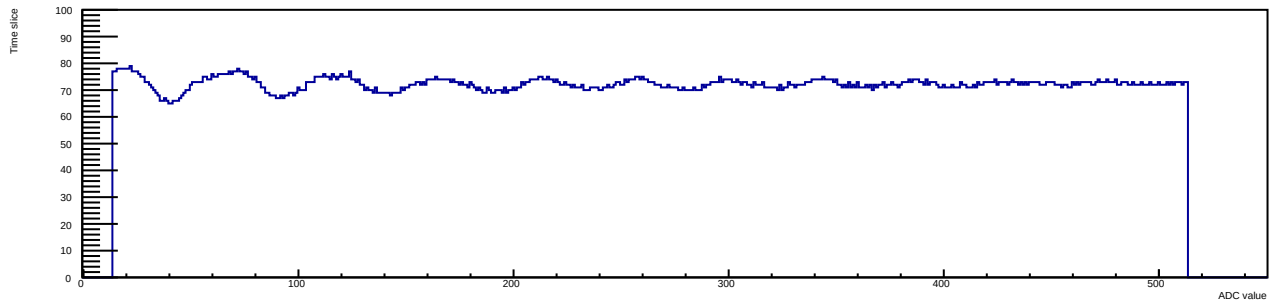
Run 12 Evt 3 Time mcm 1 chip 3 chan 6 30deg
