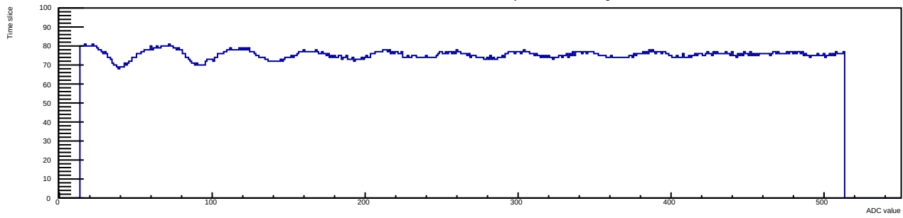
Run 12 Evt 3 Time mcm 1 chip 4 chan 1 30deg
