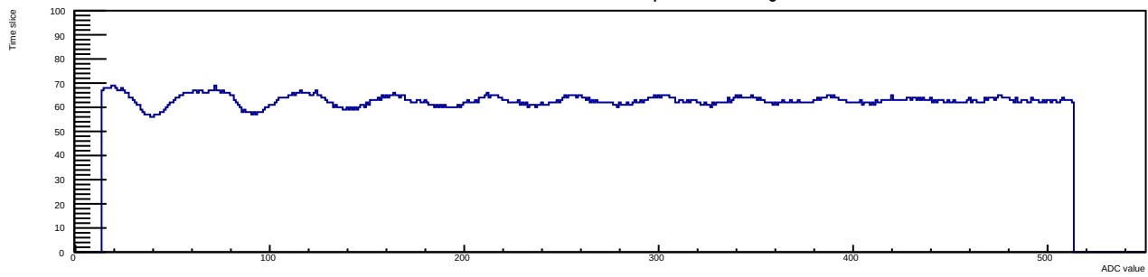
Run 12 Evt 3 Time mcm 1 chip 4 chan 2 30deg
