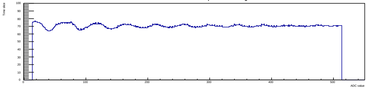
Run 12 Evt 3 Time mcm 1 chip 5 chan 4 30deg
