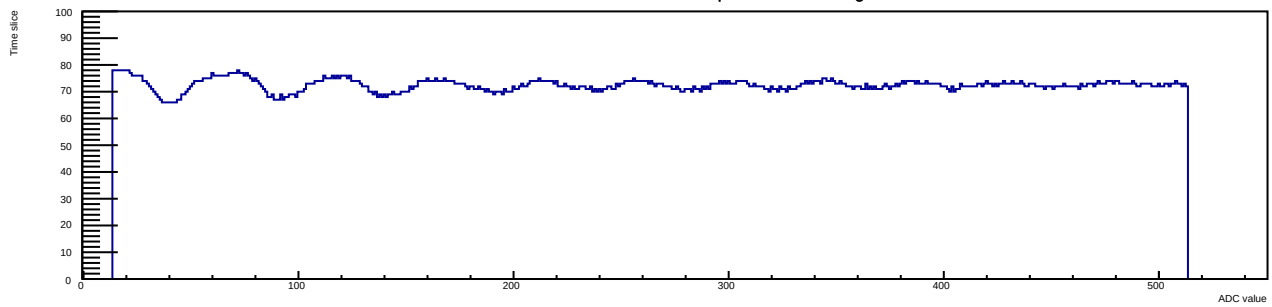
Run 12 Evt 3 Time mcm 1 chip 7 chan 11 30deg
