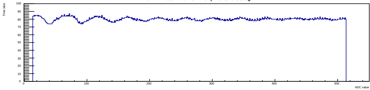
Run 12 Evt 3 Time mcm 1 chip 7 chan 0 30deg
