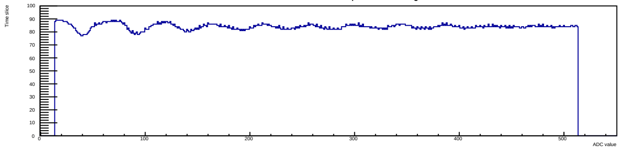
Run 12 Evt 3 Time mcm 1 chip 5 chan 1 30deg
