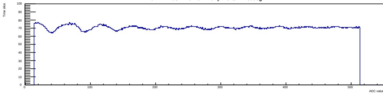
Run 12 Evt 3 Time mcm 1 chip 2 chan 12 30deg
