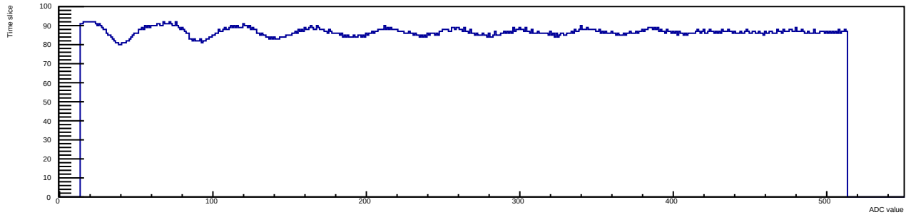
Run 12 Evt 3 Time mcm 1 chip 3 chan 5 30deg
