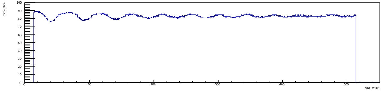
Run 12 Evt 3 Time mcm 1 chip 6 chan 1 30deg
