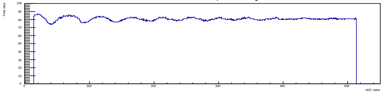
Run 12 Evt 3 Time mcm 1 chip 2 chan 0 30deg
