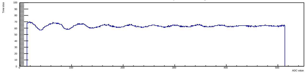
Run 12 Evt 3 Time mcm 1 chip 2 chan 9 30deg
