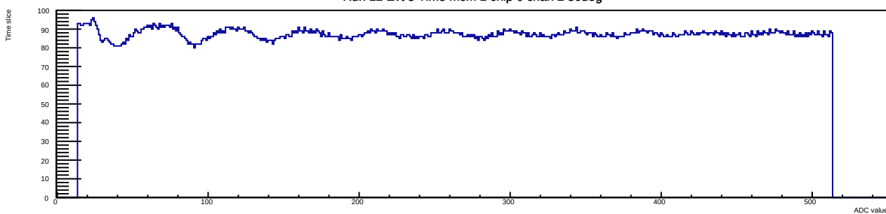
Run 12 Evt 3 Time mcm 1 chip 0 chan 2 30deg
