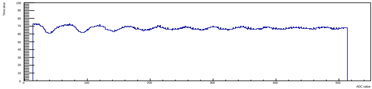
Run 12 Evt 3 Time mcm 1 chip 5 chan 7 30deg
