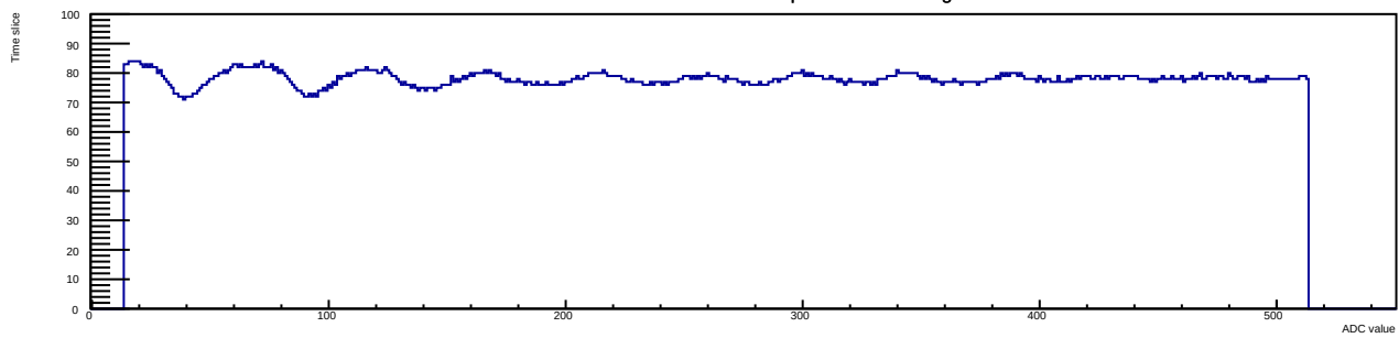
Run 12 Evt 3 Time mcm 1 chip 4 chan 10 30deg
