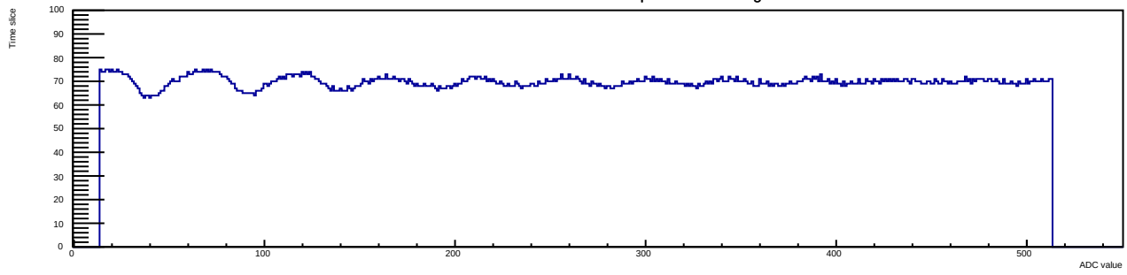
Run 12 Evt 3 Time mcm 1 chip 7 chan 8 30deg
