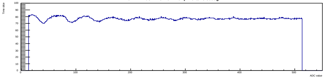
Run 12 Evt 3 Time mcm 1 chip 4 chan 8 30deg
