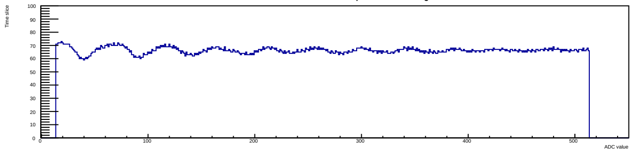
Run 12 Evt 3 Time mcm 1 chip 0 chan 14 30deg
