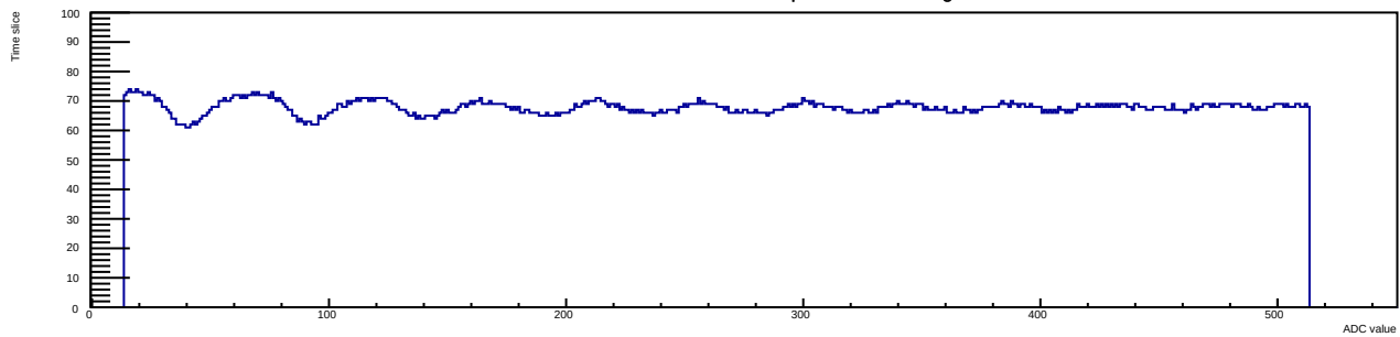
Run 12 Evt 3 Time mcm 1 chip 4 chan 15 30deg
