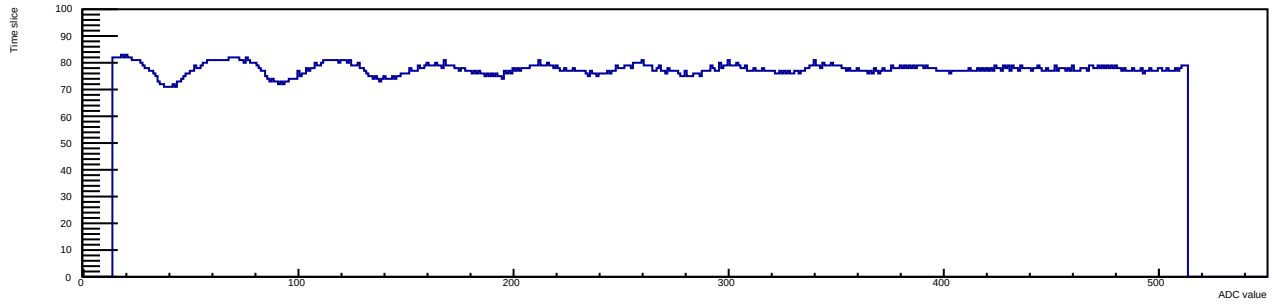
Run 12 Evt 3 Time mcm 1 chip 5 chan 5 30deg
