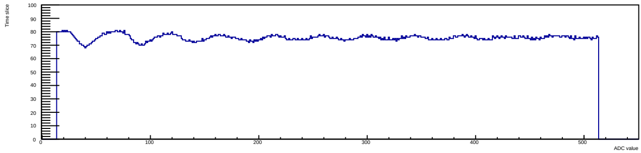
Run 12 Evt 3 Time mcm 1 chip 3 chan 2 30deg
