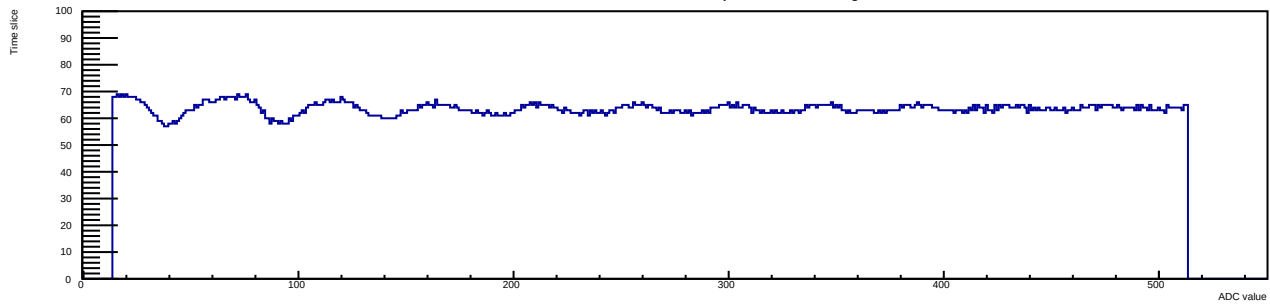
Run 12 Evt 3 Time mcm 1 chip 2 chan 1 30deg
