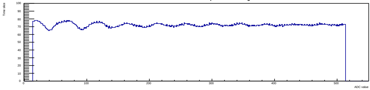
Run 12 Evt 3 Time mcm 1 chip 6 chan 0 30deg
