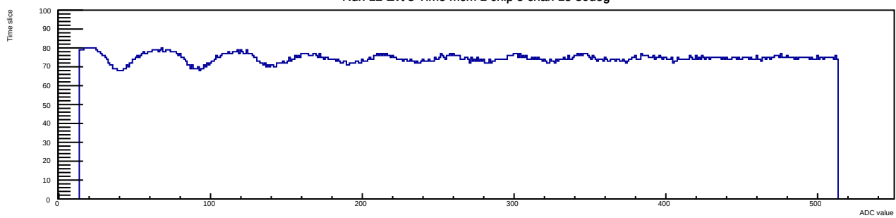
Run 12 Evt 3 Time mcm 1 chip 5 chan 15 30deg
