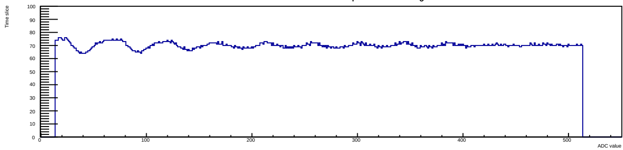
Run 12 Evt 3 Time mcm 1 chip 1 chan 14 30deg
