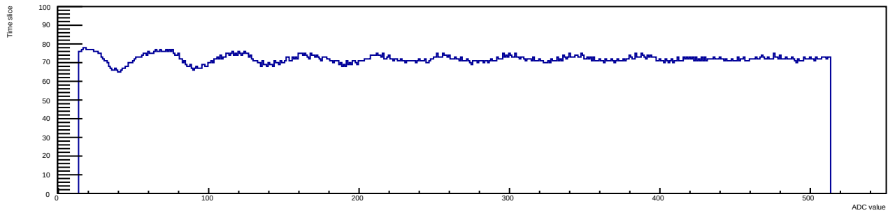
Run 12 Evt 3 Time mcm 1 chip 1 chan 3 30deg
