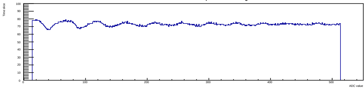
Run 12 Evt 3 Time mcm 1 chip 1 chan 15 30deg
