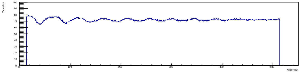
Run 12 Evt 3 Time mcm 1 chip 3 chan 7 30deg
