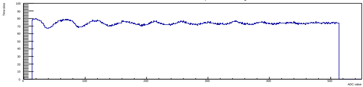
Run 12 Evt 3 Time mcm 1 chip 7 chan 14 30deg
