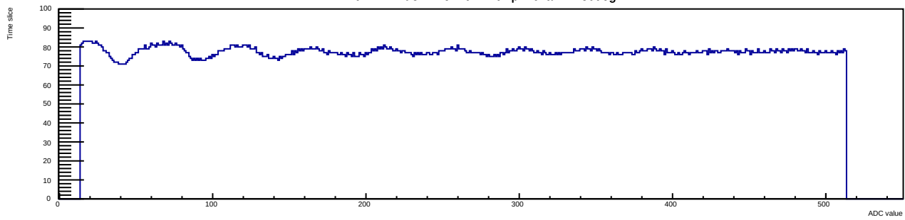
Run 12 Evt 3 Time mcm 1 chip 1 chan 12 30deg
