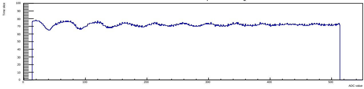
Run 12 Evt 3 Time mcm 1 chip 1 chan 8 30deg
