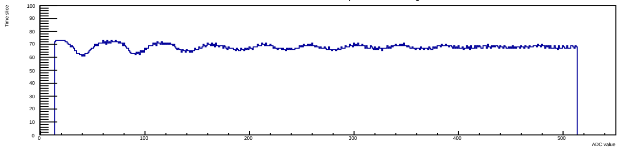
Run 12 Evt 3 Time mcm 1 chip 0 chan 15 30deg
