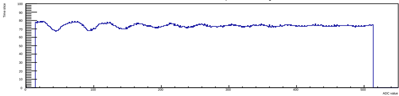
Run 12 Evt 4 Time mcm 1 chip 6 chan 14 30deg
