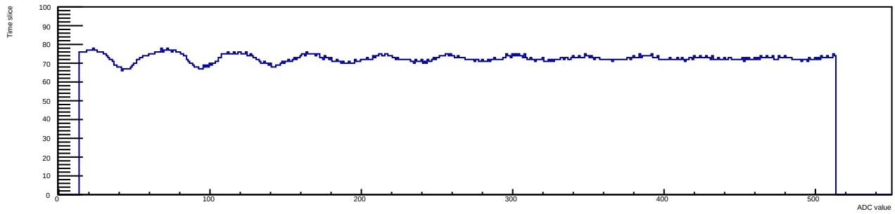
Run 12 Evt 4 Time mcm 1 chip 3 chan 10 30deg
