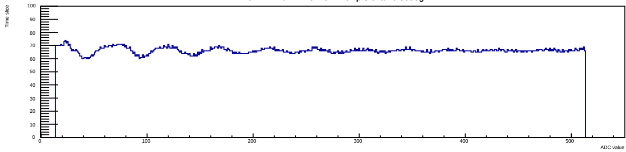
Run 12 Evt 4 Time mcm 1 chip 3 chan 0 30deg
