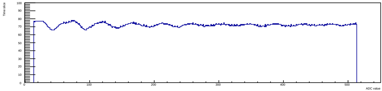
Run 12 Evt 4 Time mcm 1 chip 3 chan 7 30deg
