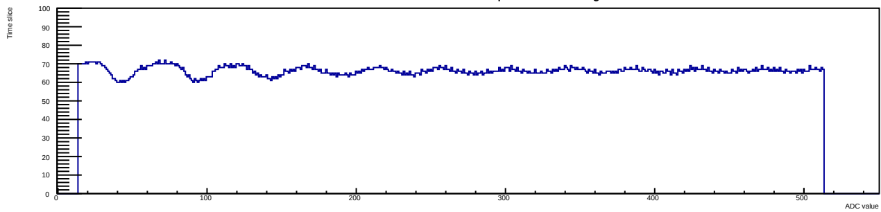
Run 12 Evt 4 Time mcm 1 chip 0 chan 14 30deg
