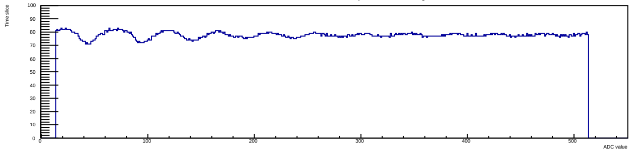
Run 12 Evt 4 Time mcm 1 chip 5 chan 5 30deg
