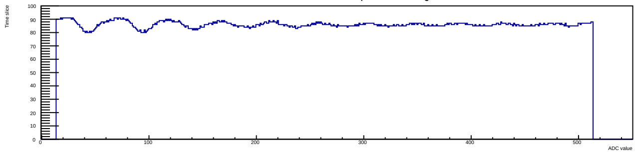
Run 12 Evt 4 Time mcm 1 chip 7 chan 6 30deg
