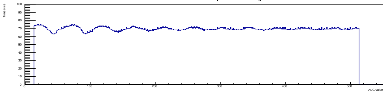
Run 12 Evt 4 Time mcm 1 chip 1 chan 13 30deg
