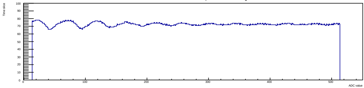
Run 12 Evt 4 Time mcm 1 chip 7 chan 11 30deg
