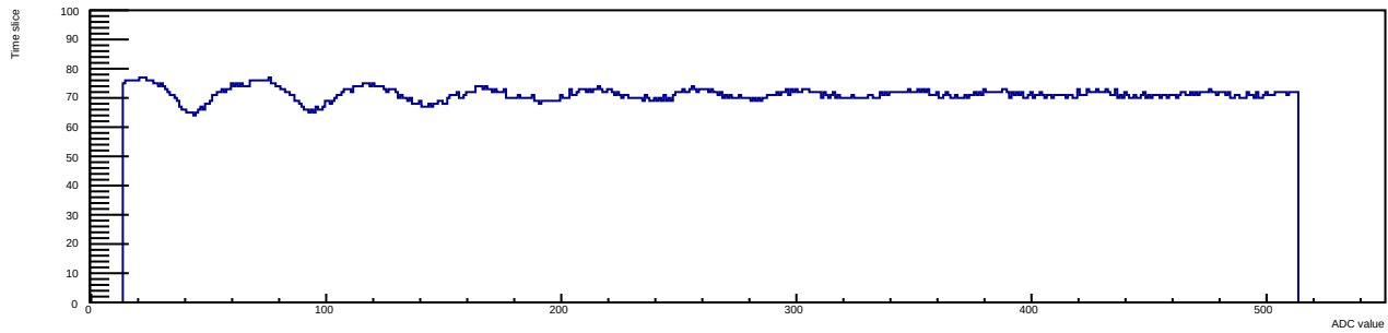
Run 12 Evt 4 Time mcm 1 chip 6 chan 3 30deg
