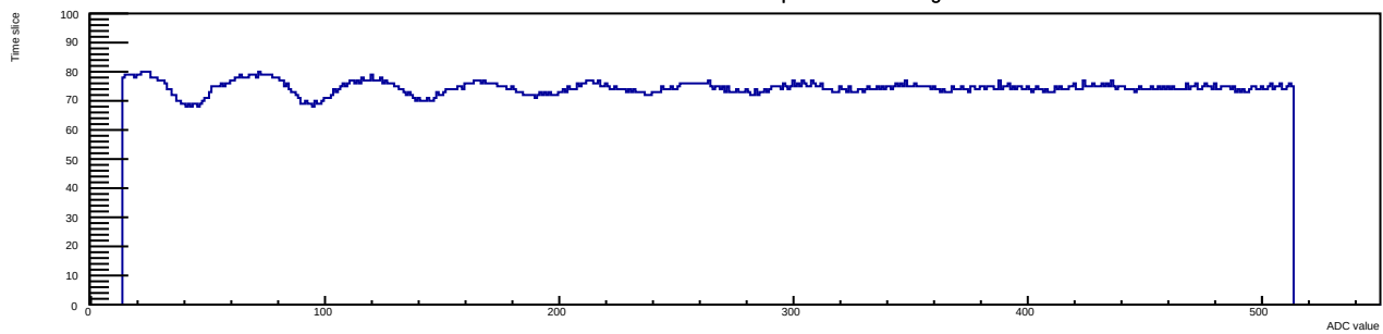
Run 12 Evt 4 Time mcm 1 chip 5 chan 15 30deg
