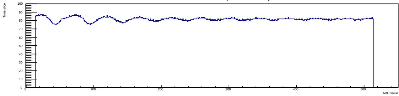
Run 12 Evt 4 Time mcm 1 chip 1 chan 1 30deg
