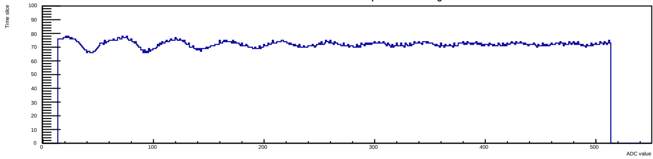
Run 12 Evt 4 Time mcm 1 chip 1 chan 8 30deg
