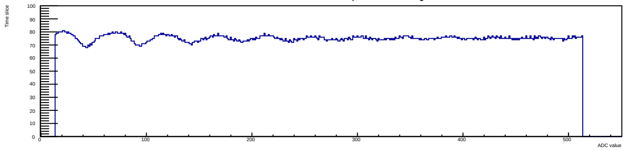
Run 12 Evt 4 Time mcm 1 chip 1 chan 10 30deg
