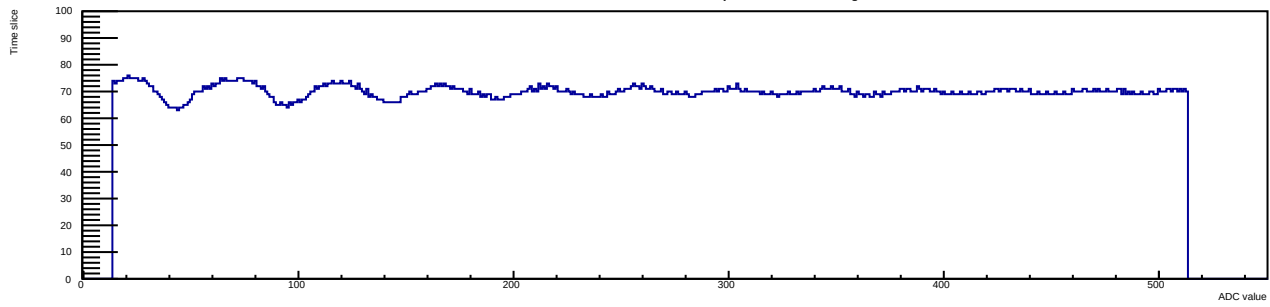
Run 12 Evt 4 Time mcm 1 chip 6 chan 5 30deg
