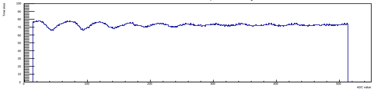
Run 12 Evt 4 Time mcm 1 chip 7 chan 13 30deg
