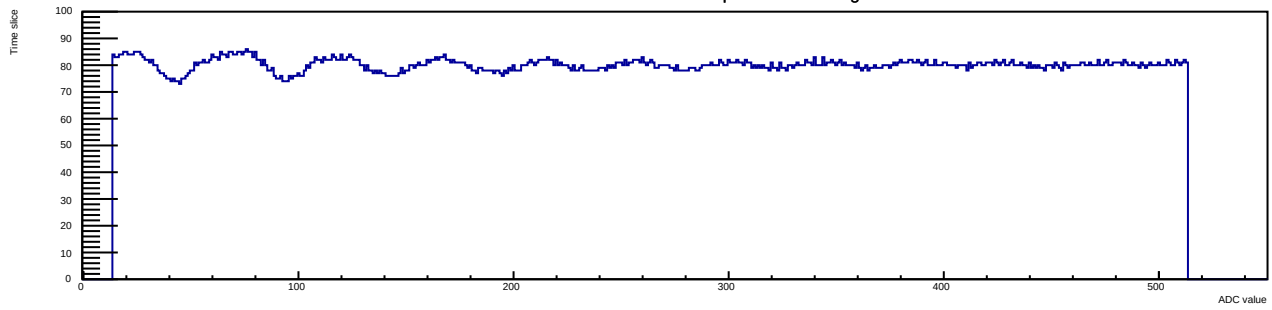
Run 12 Evt 4 Time mcm 1 chip 7 chan 0 30deg
