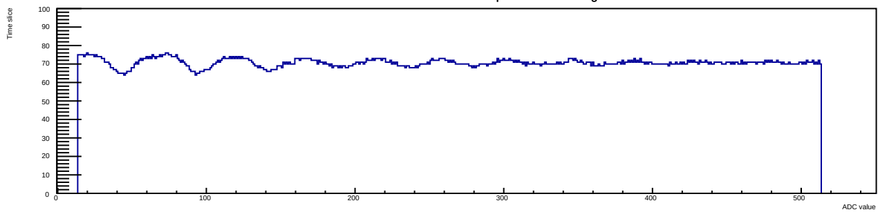
Run 12 Evt 4 Time mcm 1 chip 4 chan 11 30deg
