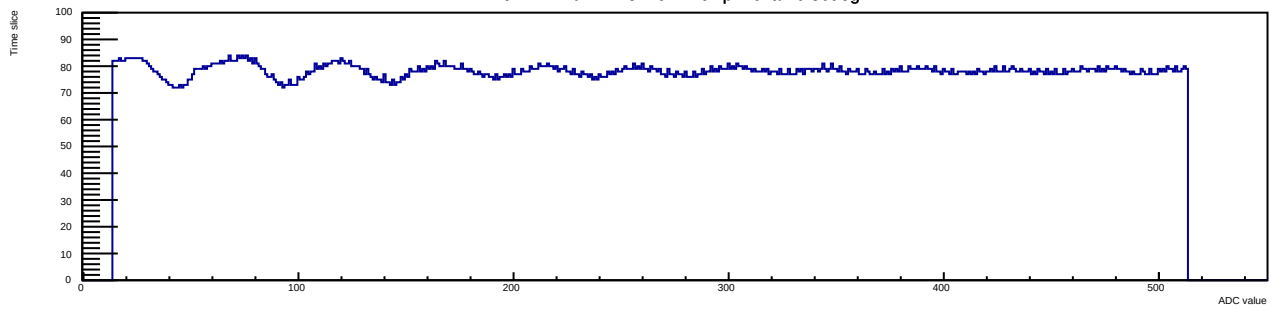
Run 12 Evt 4 Time mcm 1 chip 1 chan 0 30deg
