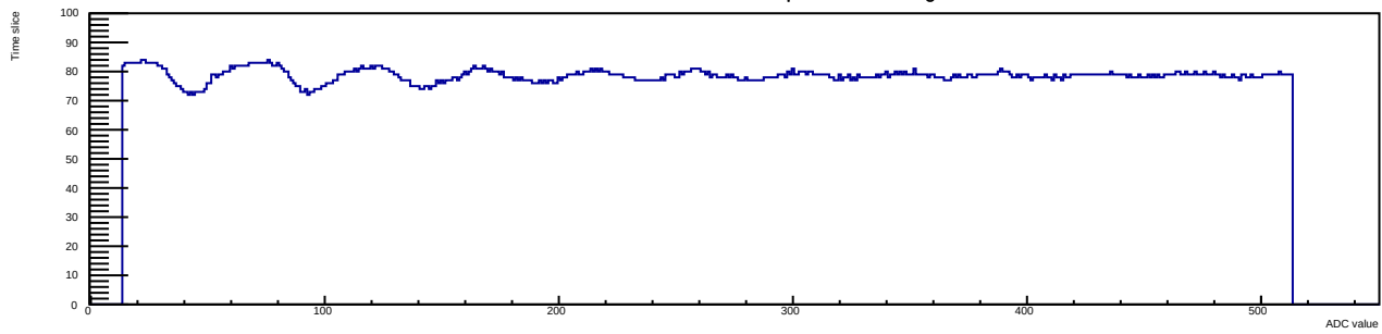
Run 12 Evt 4 Time mcm 1 chip 4 chan 9 30deg
