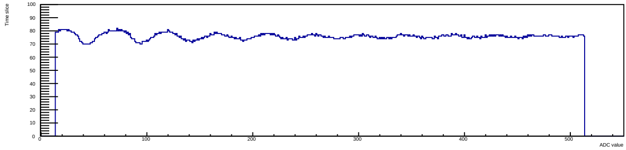
Run 12 Evt 4 Time mcm 1 chip 6 chan 9 30deg
