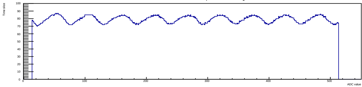
Run 13 Evt 4 Time mcm 1 chip 5 chan 9 40deg
