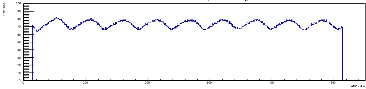
Run 13 Evt 4 Time mcm 1 chip 1 chan 4 40deg
