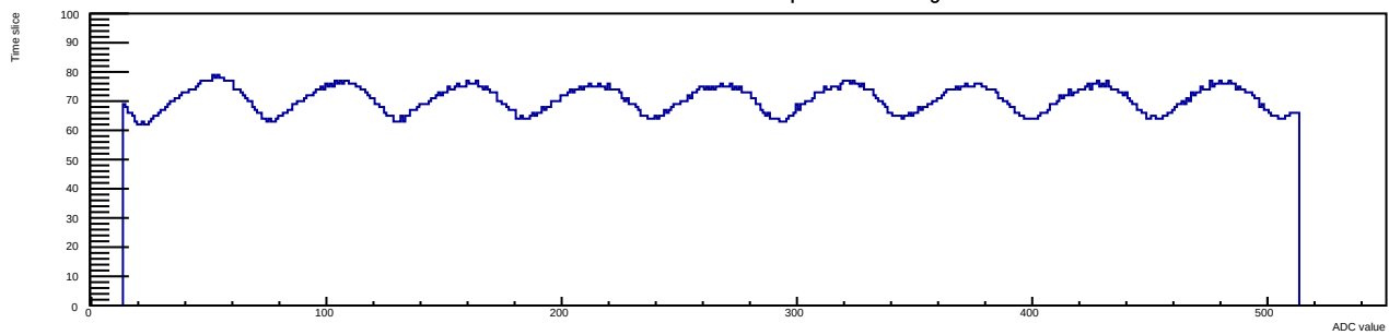
Run 13 Evt 4 Time mcm 1 chip 4 chan 3 40deg
