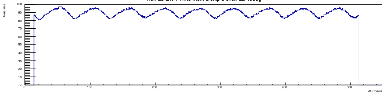
Run 13 Evt 4 Time mcm 1 chip 5 chan 12 40deg
