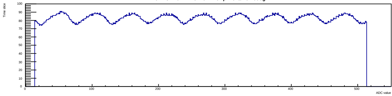
Run 13 Evt 4 Time mcm 1 chip 7 chan 0 40deg
