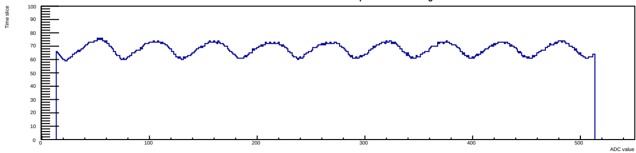
Run 13 Evt 4 Time mcm 1 chip 1 chan 11 40deg
