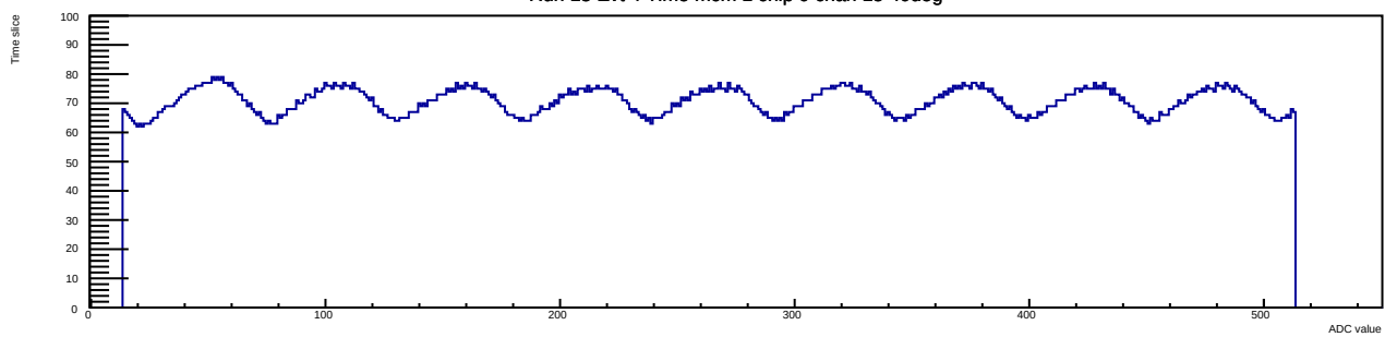
Run 13 Evt 4 Time mcm 1 chip 0 chan 15 40deg
