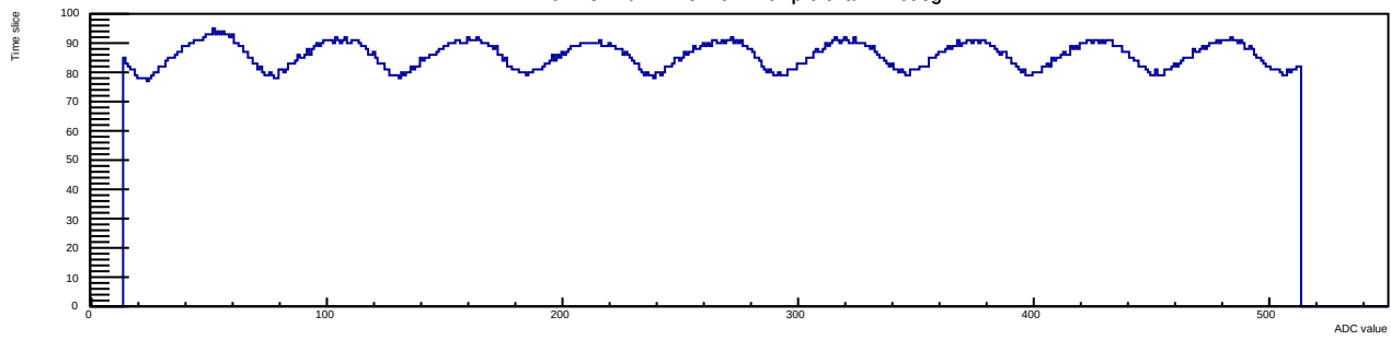
Run 13 Evt 4 Time mcm 1 chip 6 chan 4 40deg
