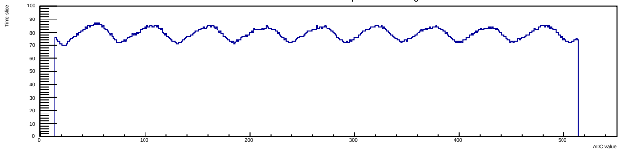
Run 13 Evt 4 Time mcm 1 chip 4 chan 8 40deg
