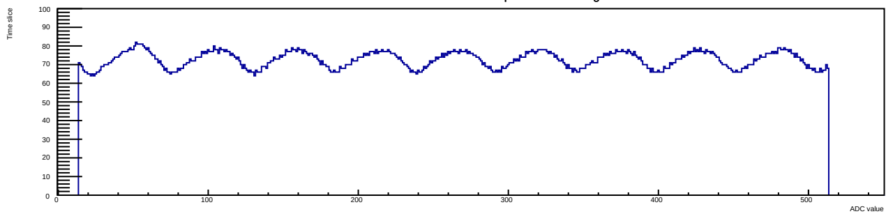
Run 13 Evt 4 Time mcm 1 chip 0 chan 3 40deg
