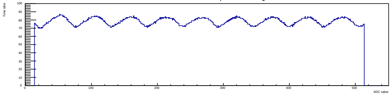
Run 13 Evt 4 Time mcm 1 chip 4 chan 12 40deg
