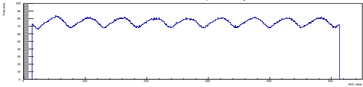
Run 13 Evt 4 Time mcm 1 chip 1 chan 5 40deg
