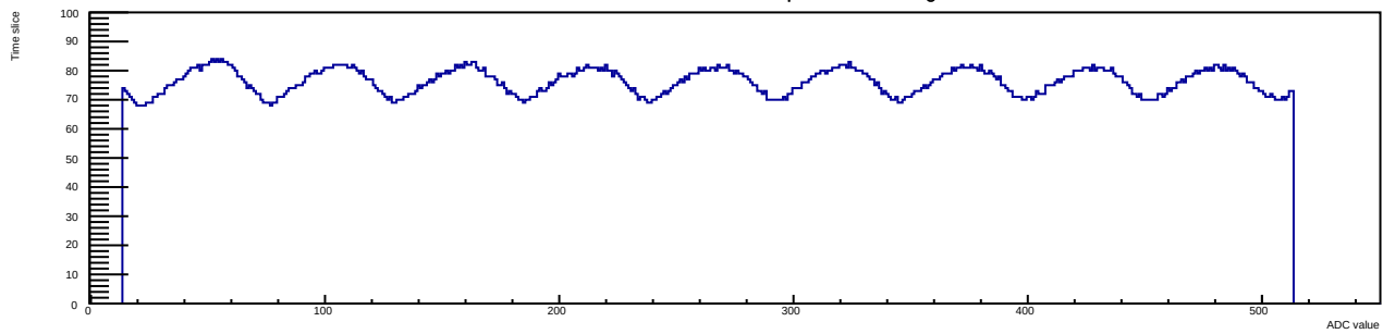
Run 13 Evt 4 Time mcm 1 chip 7 chan 7 40deg
