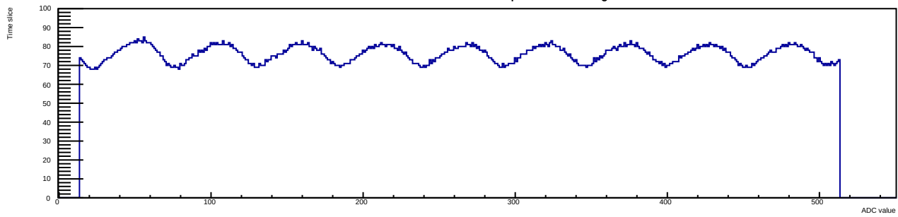
Run 13 Evt 4 Time mcm 1 chip 1 chan 9 40deg
