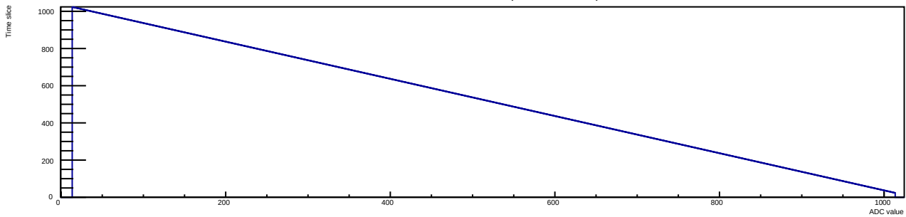
Run 18 Evt 5 Time mcm 0 chip 7 chan 4 ramps-1
