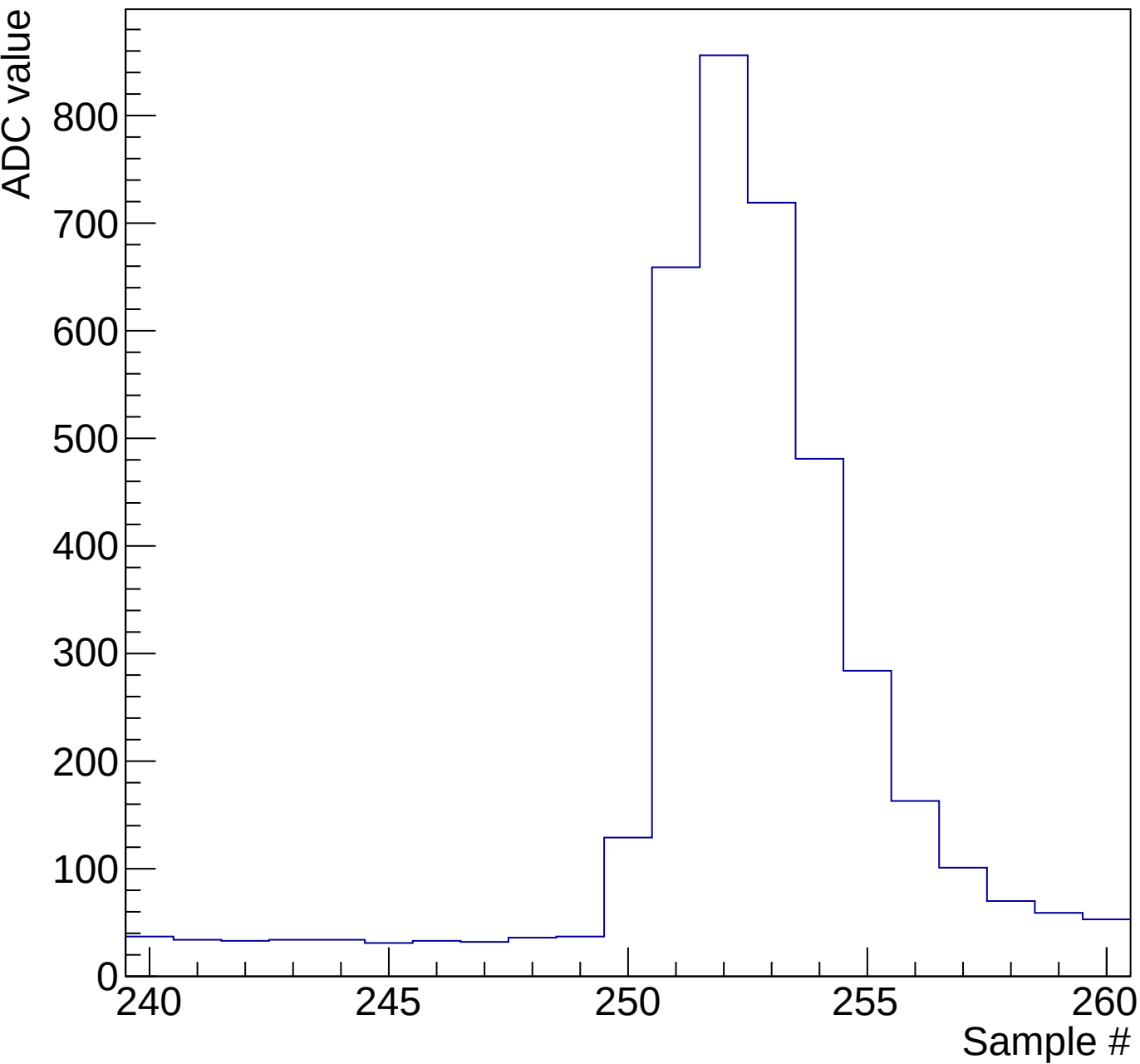
Pulstrain mcm0 evt1 run35 ch15 10ns-puls1
