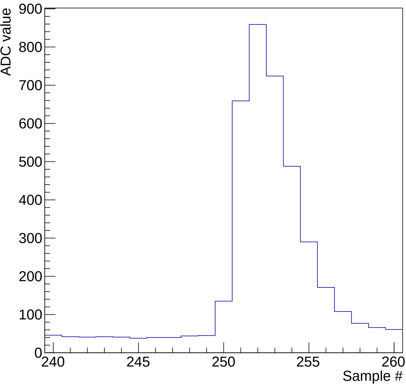
Pulstrain mcm0 evt1 run35 ch11 10ns-puls1
