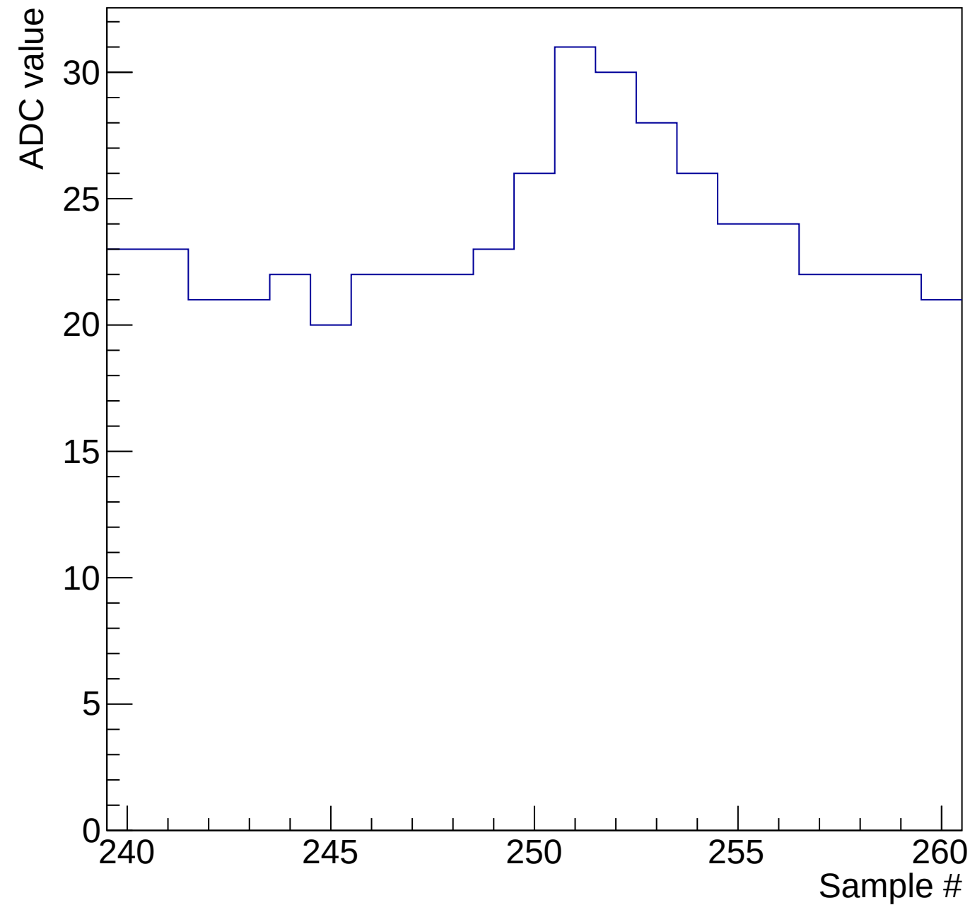
Pulstrain mcm0 evt1 run35 ch10 10ns-puls1
