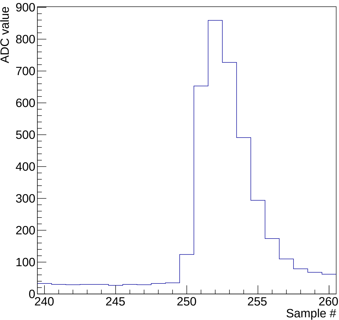
Pulstrain mcm0 evt1 run35 ch7 10ns-puls1
