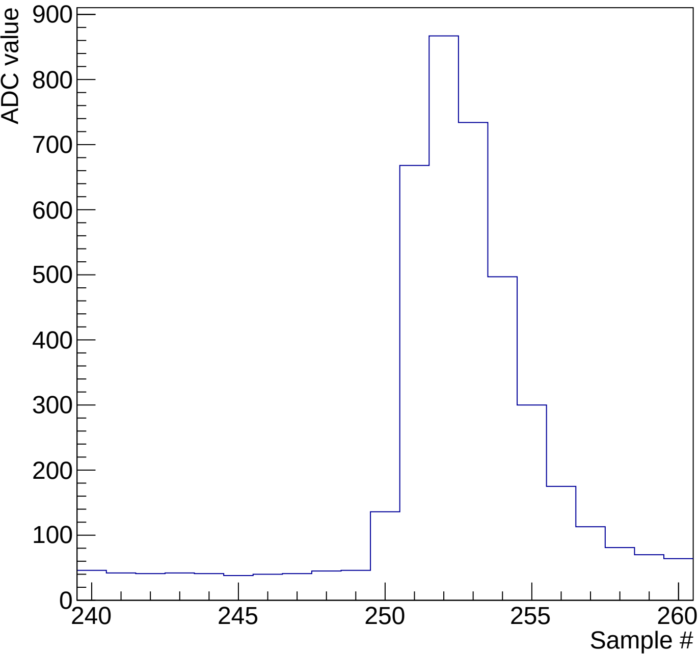
Pulstrain mcm0 evt1 run35 ch1 10ns-puls1
