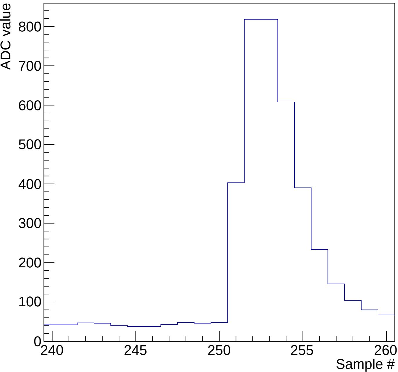
Pulstrain mcm0 evt2 run35 ch1 10ns-puls1
