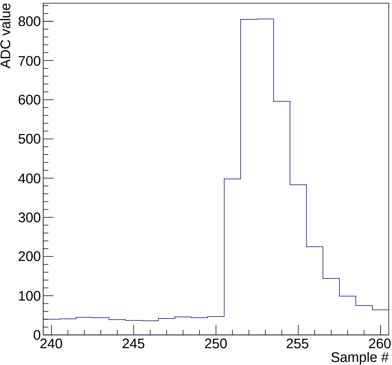
Pulstrain mcm0 evt2 run35 ch11 10ns-puls1
