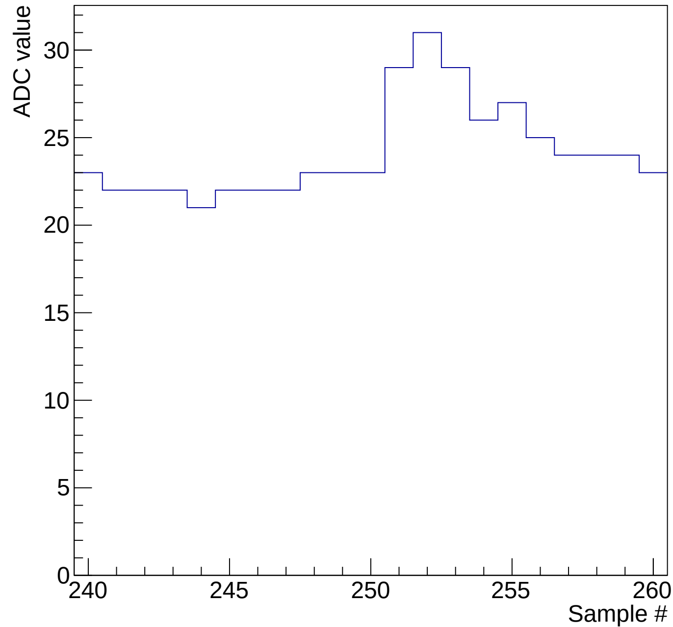
Pulstrain mcm0 evt2 run35 ch10 10ns-puls1
