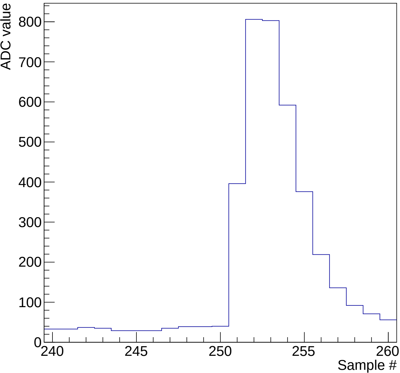
Pulstrain mcm0 evt2 run35 ch15 10ns-puls1
