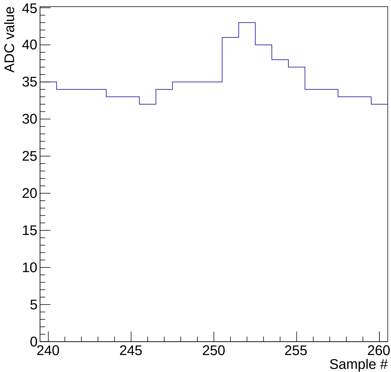
Pulstrain mcm0 evt2 run35 ch12 10ns-puls1
