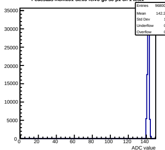
Pedestals mcm101-5E10-refV0-g0-s0-p1 ch 1 test1
