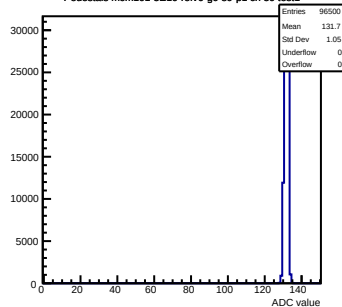
Pedestals mcm101-5E10-refV0-g0-s0-p1 ch 59 test1
