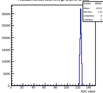
Pedestals mcm101-5E10-refV0-g0-s0-p1 ch 48 test1
