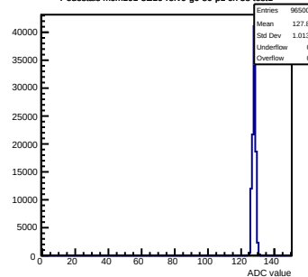
Pedestals mcm101-5E10-refV0-g0-s0-p1 ch 58 test1
