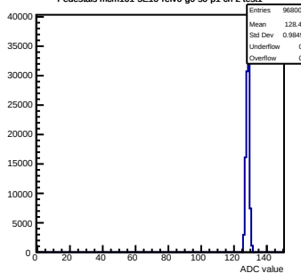
Pedestals mcm101-5E10-refV0-g0-s0-p1 ch 2 test1
