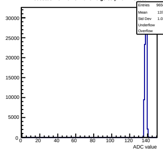
Pedestals mcm101-5E10-refV0-g0-s0-p1 ch 123 test1
