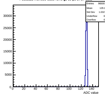
Pedestals mcm101-5E10-refV0-g0-s0-p1 ch 57 test1
