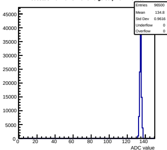
Pedestals mcm101-5E10-refV0-g0-s0-p1 ch 120 test1
