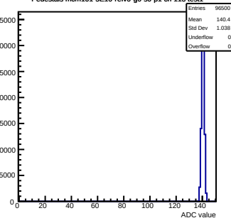
Pedestals mcm101-5E10-refV0-g0-s0-p1 ch 113 test1
