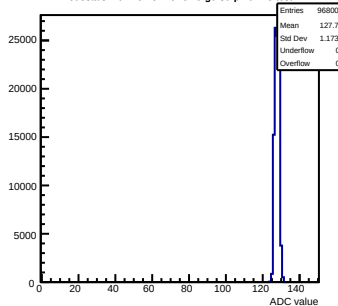
Pedestals mcm101-5E10-refV0-g0-s0-p1 ch 15 test1
