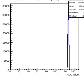
Pedestals mcm101-5E10-refV0-g0-s0-p1 ch 55 test1
