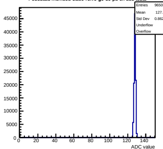
Pedestals mcm101-5E10-refV0-g0-s0-p1 ch 118 test1
