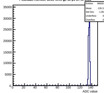
Pedestals mcm101-5E10-refV0-g0-s0-p1 ch 49 test1
