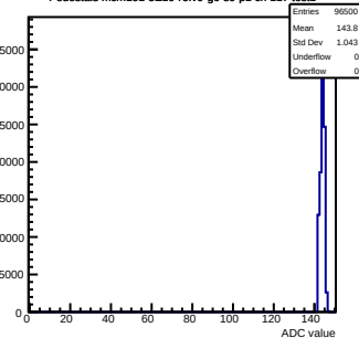
Pedestals mcm101-5E10-refV0-g0-s0-p1 ch 117 test1
