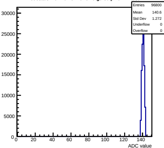
Pedestals mcm101-5E10-refV0-g0-s0-p1 ch 12 test1
