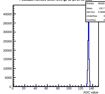
Pedestals mcm101-5E10-refV0-g0-s0-p1 ch 51 test1
