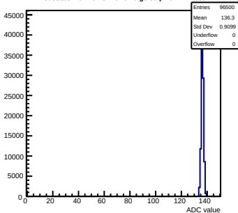
Pedestals mcm101-5E10-refV0-g0-s0-p1 ch 124 test1
