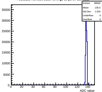
Pedestals mcm101-5E10-refV0-g0-s0-p1 ch 116 test1
