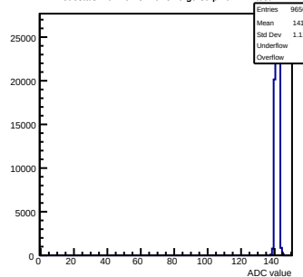
Pedestals mcm101-5E10-refV0-g0-s0-p1 ch 127 test1
