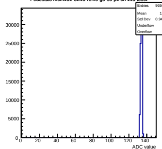
Pedestals mcm101-5E10-refV0-g0-s0-p1 ch 115 test1
