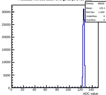
Pedestals mcm101-5E10-refV0-g0-s0-p1 ch 56 test1
