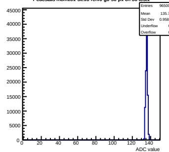
Pedestals mcm101-5E10-refV0-g0-s0-p1 ch 50 test1
