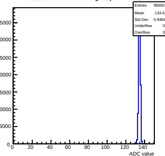
Pedestals mcm101-5E10-refV0-g0-s0-p1 ch 125 test1
