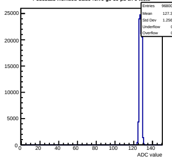
Pedestals mcm101-5E10-refV0-g0-s0-p1 ch 9 test1
