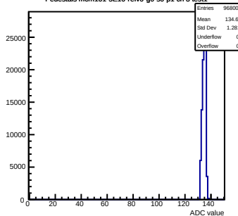
Pedestals mcm101-5E10-refV0-g0-s0-p1 ch 3 test1
