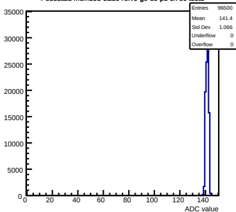
Pedestals mcm101-5E10-refV0-g0-s0-p1 ch 60 test1
