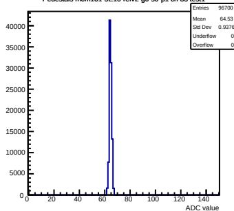
Pedestals mcm101-5E10-ref2-g0-s0-p1 ch 83 test1
