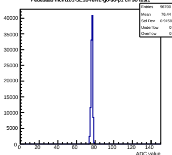
Pedestals mcm101-5E10-ref2-g0-s0-p1 ch 90 test1
