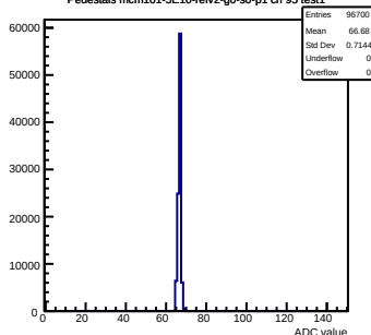
Pedestals mcm101-5E10-ref2-g0-s0-p1 ch 95 test1
