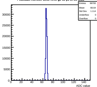
Pedestals mcm101-5E10-ref2-g0-s0-p1 ch 81 test1
