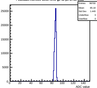
Pedestals mcm101-5E10-ref2-g0-s0-p1 ch 80 test1
