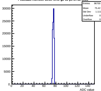
Pedestals mcm101-5E10-ref2-g0-s0-p1 ch 82 test1
