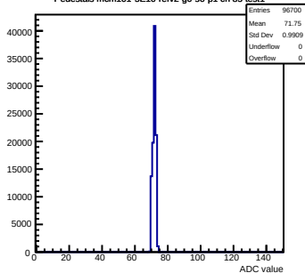
Pedestals mcm101-5E10-ref2-g0-s0-p1 ch 85 test1
