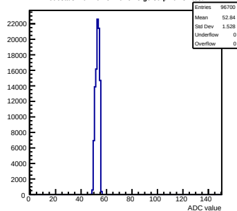
Pedestals mcm101-5E10-refV3-g0-s0-p1 ch 31 test1
