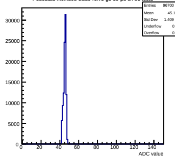
Pedestals mcm101-5E10-refV3-g0-s0-p1 ch 23 test1
