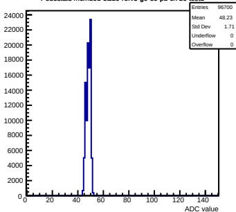
Pedestals mcm101-5E10-refV3-g0-s0-p1 ch 20 test1
