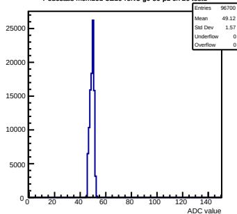
Pedestals mcm101-5E10-refV3-g0-s0-p1 ch 26 test1
