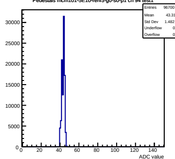
Pedestals mcm101-5E10-refV3-g0-s0-p1 ch 94 test1
