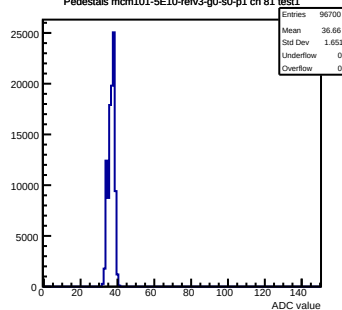
Pedestals mcm101-5E10-refV3-g0-s0-p1 ch 81 test1
