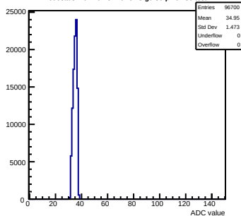
Pedestals mcm101-5E10-refV3-g0-s0-p1 ch 30 test1
