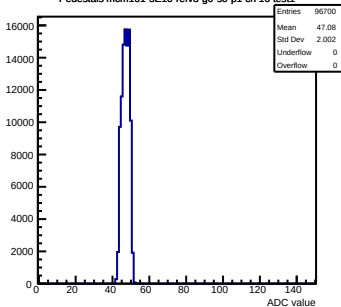
Pedestals mcm101-5E10-refV3-g0-s0-p1 ch 16 test1
