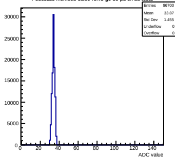
Pedestals mcm101-5E10-refV3-g0-s0-p1 ch 22 test1
