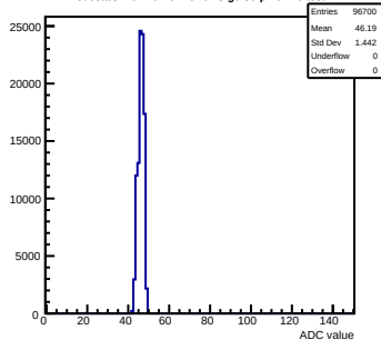
Pedestals mcm101-5E10-refV3-g0-s0-p1 ch 29 test1
