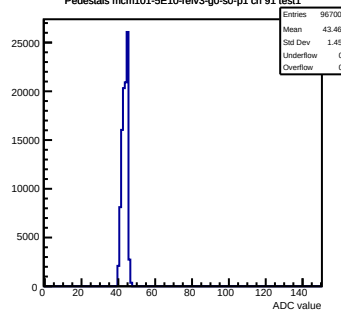
Pedestals mcm101-5E10-refV3-g0-s0-p1 ch 91 test1
