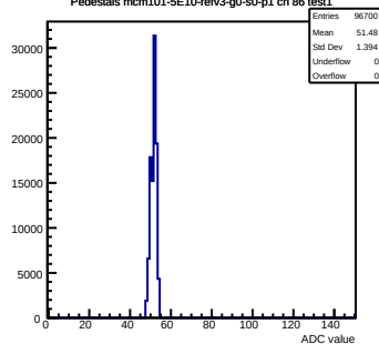
Pedestals mcm101-5E10-refV3-g0-s0-p1 ch 86 test1
