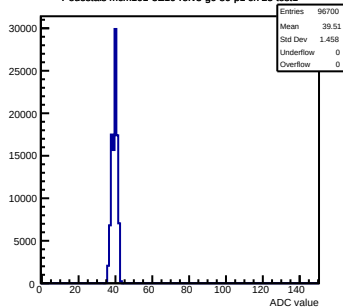
Pedestals mcm101-5E10-refV3-g0-s0-p1 ch 25 test1
