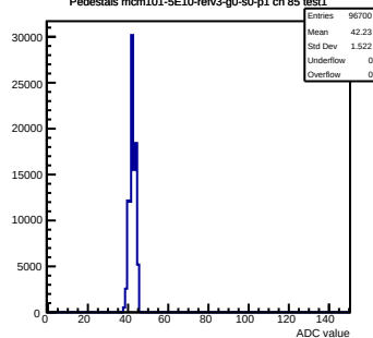
Pedestals mcm101-5E10-refV3-g0-s0-p1 ch 85 test1
