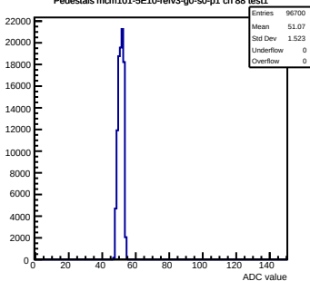
Pedestals mcm101-5E10-refV3-g0-s0-p1 ch 88 test1
