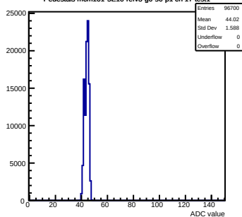
Pedestals mcm101-5E10-refV3-g0-s0-p1 ch 17 test1
