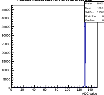
Pedestals mcm101-5E10-refV6-g0-s0-p1 ch 118 test1
