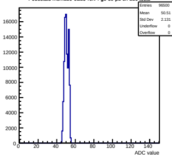
Pedestals mcm120-6E15-refV4-g0-s0-p1 ch 116 test1
