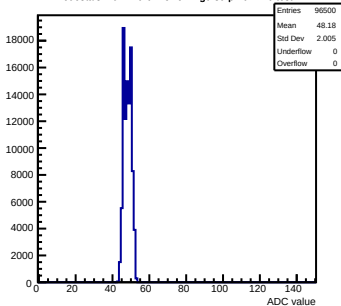
Pedestals mcm120-6E15-refV4-g0-s0-p1 ch 120 test1
