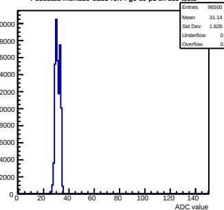
Pedestals mcm120-6E15-refV4-g0-s0-p1 ch 119 test1
