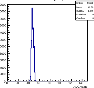
Pedestals mcm120-6E15-refV4-g0-s0-p1 ch 127 test1
