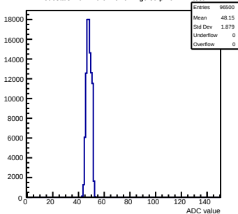
Pedestals mcm120-6E15-refV4-g0-s0-p1 ch 124 test1
