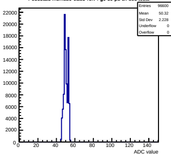
Pedestals mcm120-6E15-refv4-g0-s0-p1 ch 108 test1
