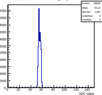
Pedestals mcm120-6E15-refV4-g0-s0-p1 ch 121 test1
