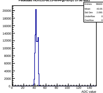
Pedestals mcm120-6E15-refv4-g0-s0-p1 ch 98 test1
