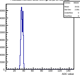
Pedestals mcm120-6E15-refV4-g0-s0-p1 ch 113 test1
