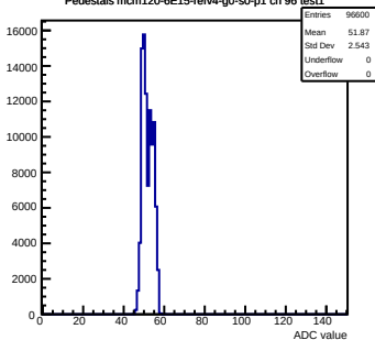
Pedestals mcm120-6E15-refv4-g0-s0-p1 ch 96 test1
