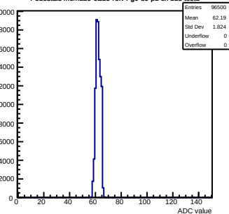
Pedestals mcm120-6E15-refV4-g0-s0-p1 ch 118 test1
