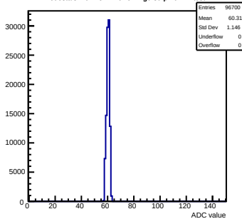
Pedestals mcm151-E16-refv4-g0-s0-p1 ch 27 test1
