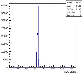
Pedestals mcm151-E16-refv4-g0-s0-p1 ch 88 test1
