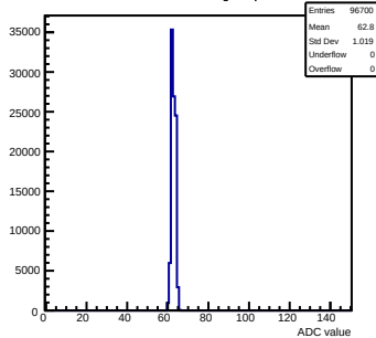
Pedestals mcm151-E16-refv4-g0-s0-p1 ch 95 test1
