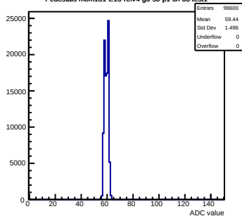
Pedestals mcm151-E16-refv4-g0-s0-p1 ch 33 test1
