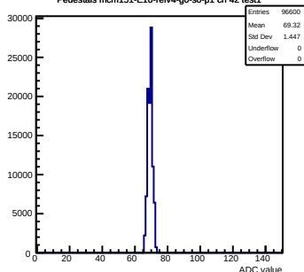
Pedestals mcm151-E16-refv4-g0-s0-p1 ch 42 test1
