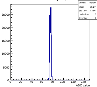
Pedestals mcm151-E16-refv4-g0-s0-p1 ch 84 test1
