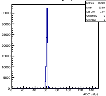
Pedestals mcm151-E16-refv4-g0-s0-p1 ch 86 test1
