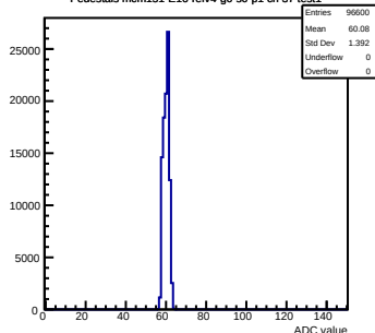
Pedestals mcm151-E16-refv4-g0-s0-p1 ch 37 test1
