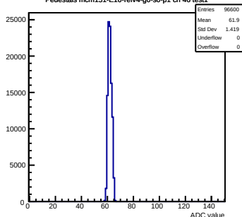
Pedestals mcm151-E16-refv4-g0-s0-p1 ch 46 test1
