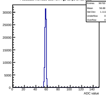
Pedestals mcm151-E16-refv4-g0-s0-p1 ch 83 test1
