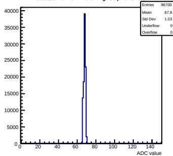
Pedestals mcm151-E16-refv4-g0-s0-p1 ch 87 test1
