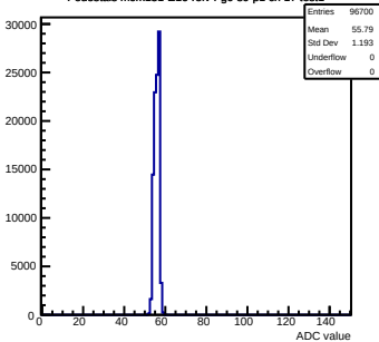
Pedestals mcm151-E16-refv4-g0-s0-p1 ch 17 test1
