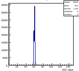
Pedestals mcm151-E16-refv4-g0-s0-p1 ch 94 test1
