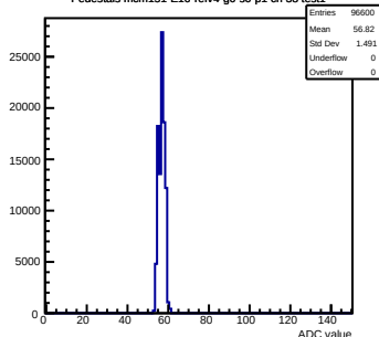
Pedestals mcm151-E16-refv4-g0-s0-p1 ch 38 test1
