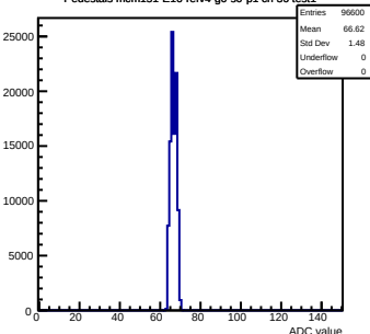
Pedestals mcm151-E16-refv4-g0-s0-p1 ch 36 test1
