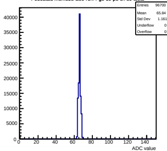
Pedestals mcm151-E16-refv4-g0-s0-p1 ch 19 test1
