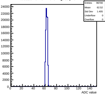
Pedestals mcm151-E16-refv4-g0-s0-p1 ch 20 test1
