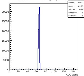
Pedestals mcm151-E16-refv4-g0-s0-p1 ch 89 test1
