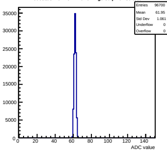
Pedestals mcm151-E16-refv4-g0-s0-p1 ch 30 test1
