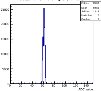
Pedestals mcm151-E16-refv4-g0-s0-p1 ch 16 test1
