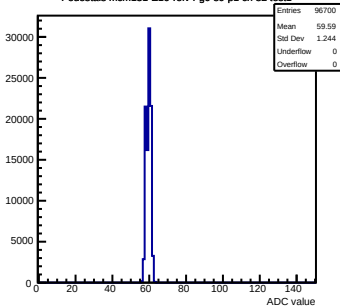
Pedestals mcm151-E16-refv4-g0-s0-p1 ch 82 test1
