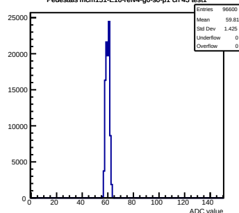
Pedestals mcm151-E16-refv4-g0-s0-p1 ch 43 test1
