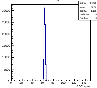
Pedestals mcm151-E16-refv4-g0-s0-p1 ch 31 test1
