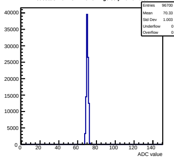
Pedestals mcm151-E16-refv4-g0-s0-p1 ch 91 test1
