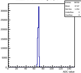
Pedestals mcm151-E16-refv4-g0-s0-p1 ch 24 test1
