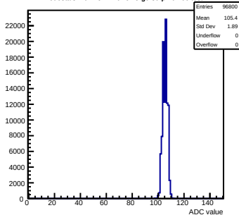
Pedestals mcm151-E16- \text{refV5-g0-s0-p1} ch 66 test1
