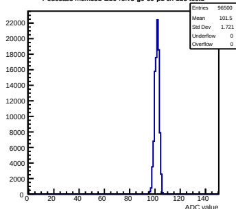
Pedestals mcm151-E16-refV5-g0-s0-p1 ch 123 test1
