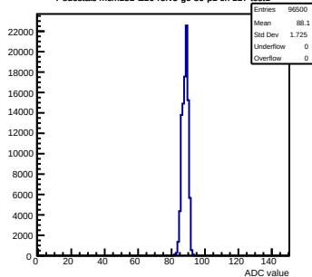
Pedestals mcm151-E16-refV5-g0-s0-p1 ch 117 test1
