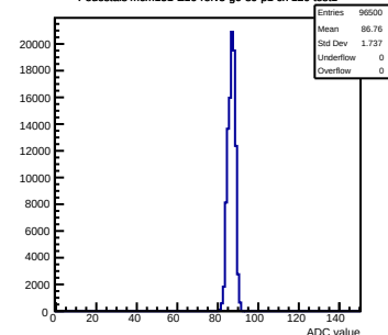
Pedestals mcm151-E16-refV5-g0-s0-p1 ch 120 test1
