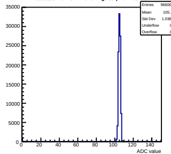
Pedestals mcm151-E16-refv1-g0-s0-p1 ch 99 test1
