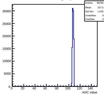
Pedestals mcm151-E16-refv1-q0-s0-p1 ch 25 test1
