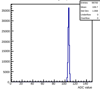
Pedestals mcm151-E16-refv1-q0-s0-p1 ch 24 test1
