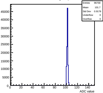
Pedestals mcm151-E16-refv1-g0-s0-p1 ch 95 test1
