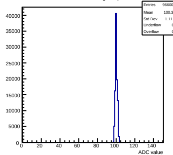
Pedestals mcm151-E16-refv1-g0-s0-p1 ch 111 test1
