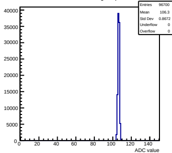
Pedestals mcm151-E16-refv1-g0-s0-p1 ch 93 test1
