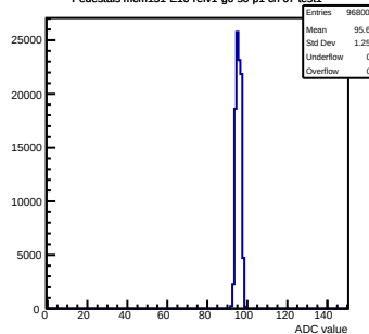
Pedestals mcm151-E16-refv1-q0-s0-p1 ch 67 test1
