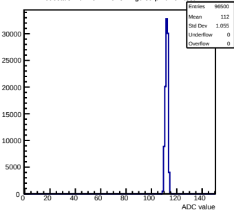
Pedestals mcm151-E16-refv1-g0-s0-p1 ch 52 test1
