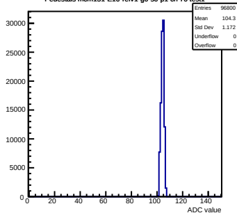
Pedestals mcm151-E16-refv1-q0-s0-p1 ch 70 test1
