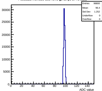
Pedestals mcm151-E16-refv1-q0-s0-p1 ch 72 test1
