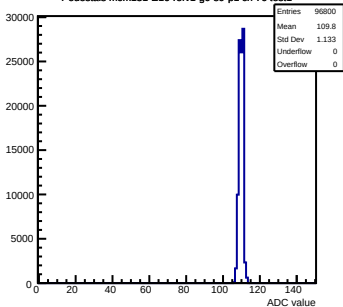
Pedestals mcm151-E16-refv1-q0-s0-p1 ch 76 test1
