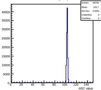
Pedestals mcm151-E16-refv1-q0-s0-p1 ch 88 test1
