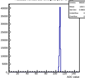
Pedestals mcm151-E16-refv1-g0-s0-p1 ch 49 test1
