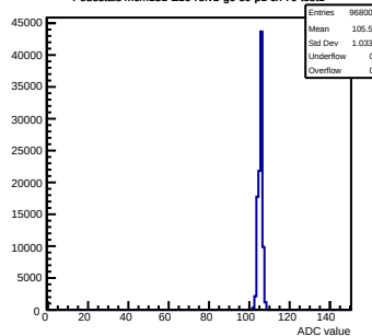
Pedestals mcm151-E16-refv1-q0-s0-p1 ch 79 test1
