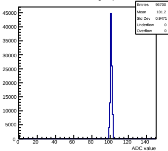
Pedestals mcm151-E16-refv1-q0-s0-p1 ch 26 test1
