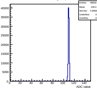
Pedestals mcm151-E16-refv1-g0-s0-p1 ch 57 test1
