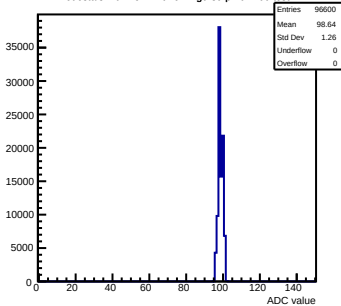
Pedestals mcm151-E16-refv1-g0-s0-p1 ch 96 test1
