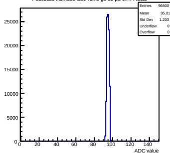
Pedestals mcm151-E16-refv1-q0-s0-p1 ch 74 test1
