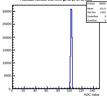
Pedestals mcm151-E16-refv1-q0-s0-p1 ch 65 test1
