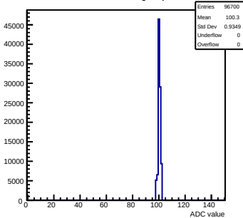
Pedestals mcm151-E16-refv1-q0-s0-p1 ch 94 test1
