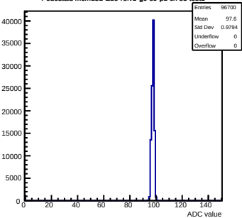
Pedestals mcm151-E16-refv1-g0-s0-p1 ch 83 test1
