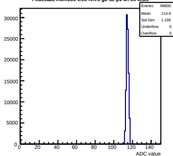
Pedestals mcm151-E16-refv1-q0-s0-p1 ch 69 test1
