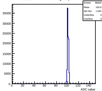
Pedestals mcm151-E16-refv1-g0-s0-p1 ch 98 test1
