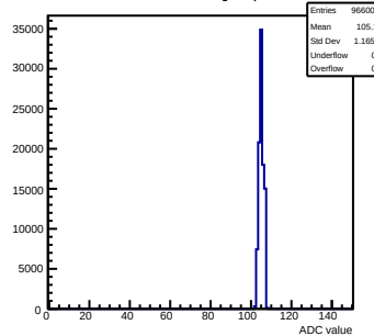
Pedestals mcm151-E16-refv1-g0-s0-p1 ch 107 test1
