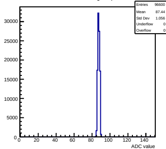
Pedestals mcm151-E16-refv1-g0-s0-p1 ch 110 test1
