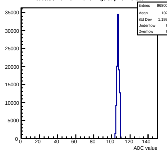
Pedestals mcm151-E16-refv1-q0-s0-p1 ch 75 test1
