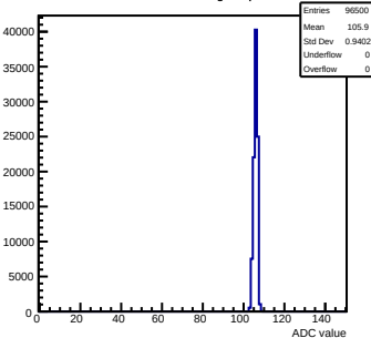
Pedestals mcm151-E16-refv1-g0-s0-p1 ch 61 test1
