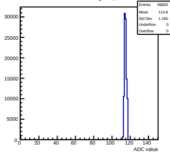
Pedestals mcm151-E16-refv1-g0-s0-p1 ch 109 test1
