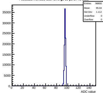
Pedestals mcm151-E16-refv1-q0-s0-p1 ch 73 test1
