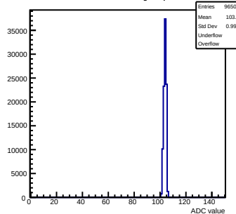
Pedestals mcm151-E16-refv1-g0-s0-p1 ch 59 test1
