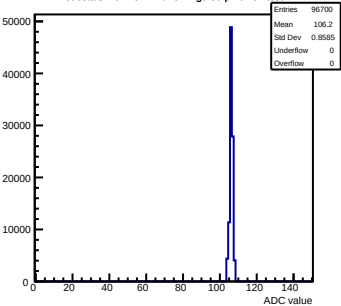
Pedestals mcm151-E16-refv1-g0-s0-p1 ch 87 test1
