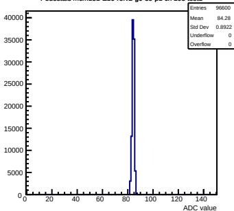
Pedestals mcm151-E16-refv2-g0-s0-p1 ch 108 test1
