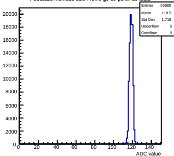
Pedestals mcm153-5E14-refV0-g0-s0-p1 ch 39 test1
