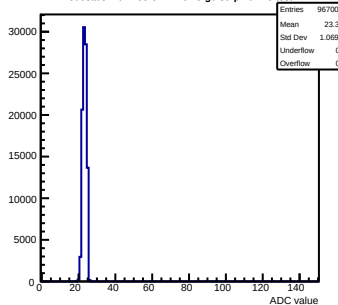
Pedestals mcm153-5E14-refv3-g0-s0-p1 ch 23 test1
