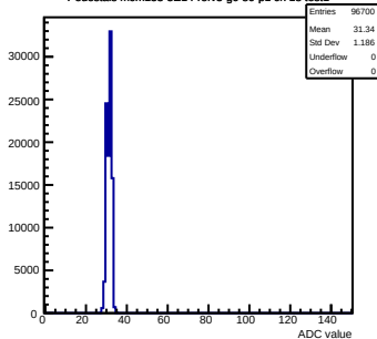
Pedestals mcm153-5E14-refv3-g0-s0-p1 ch 18 test1
