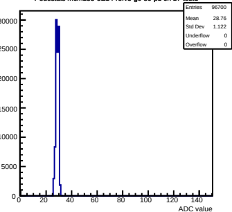
Pedestals mcm153-5E14-refv3-g0-s0-p1 ch 17 test1
