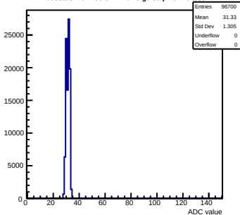
Pedestals mcm153-5E14-refv3-g0-s0-p1 ch 20 test1
