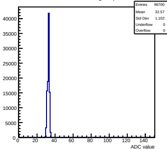
Pedestals mcm153-5E14-refv3-g0-s0-p1 ch 24 test1
