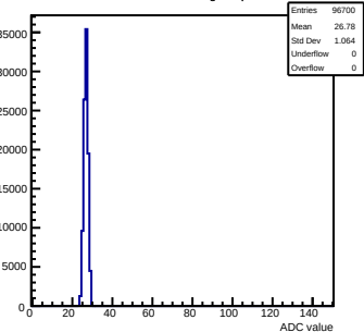
Pedestals mcm153-5E14-refv3-g0-s0-p1 ch 29 test1
