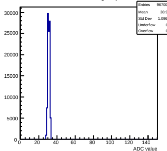
Pedestals mcm153-5E14-refv3-g0-s0-p1 ch 27 test1
