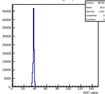
Pedestals mcm153-5E14-refv3-g0-s0-p1 ch 22 test1
