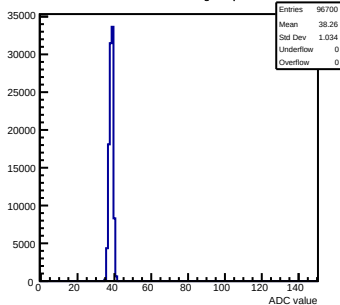
Pedestals mcm153-5E14-refv3-g0-s0-p1 ch 30 test1
