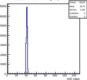
Pedestals mcm153-5E14-refv3-g0-s0-p1 ch 21 test1
