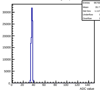
Pedestals mcm153-5E14-refv3-g0-s0-p1 ch 31 test1
