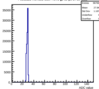
Pedestals mcm153-5E14-refv3-g0-s0-p1 ch 19 test1
