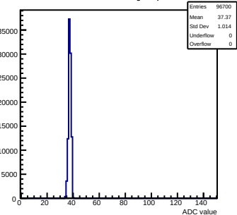
Pedestals mcm153-5E14-refv3-g0-s0-p1 ch 25 test1
