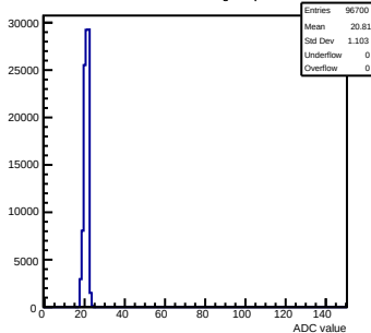
Pedestals mcm153-5E14-refv3-g0-s0-p1 ch 26 test1
