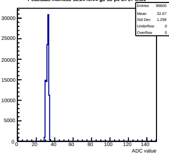
Pedestals mcm153-5E14-refv4-g0-s0-p1 ch 97 test1
