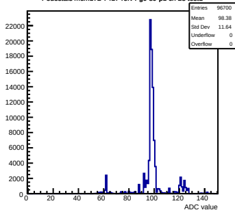
Pedestals mcm172-7417-recv4-g0-s0-p1 ch 28 test1
