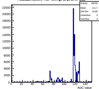
Pedestals mcm172-7417-recv4-g0-s0-p1 ch 17 test1
