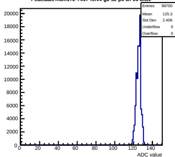
Pedestals mcm172-7417-recv4-g0-s0-p1 ch 16 test1
