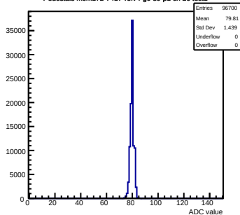
Pedestals mcm172-7417-recv4-g0-s0-p1 ch 26 test1
