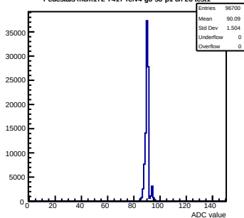
Pedestals mcm172-7417-recv4-g0-s0-p1 ch 20 test1
