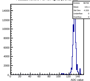
Pedestals mcm172-7417-recv4-g0-s0-p1 ch 30 test1
