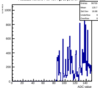
Pedestals mcm172-7417-recv4-g0-s0-p1 ch 27 test1
