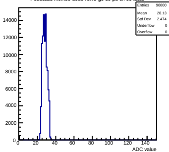
Pedestals mcm80-1016-refv3-g0-s0-p1 ch 96 test1
