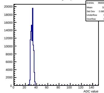
Pedestals mcm80-1016-refv3-g0-s0-p1 ch 111 test1
