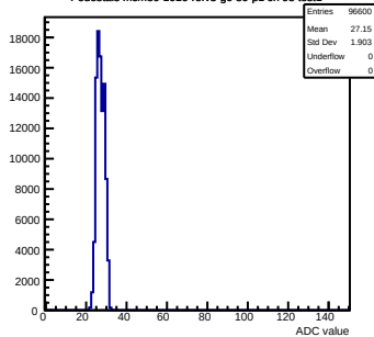
Pedestals mcm80-1016-refv3-g0-s0-p1 ch 98 test1
