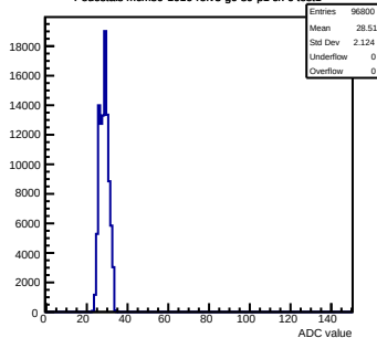
Pedestals mcm80-1016-refv3-g0-s0-p1 ch 6 test1
