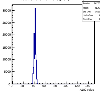
Pedestals mcm80-1016-refv3-g0-s0-p1 ch 94 test1
