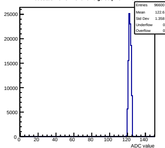
Pedestals mcm81-1816-refV0-g0-s0-p1 ch 42 test1
