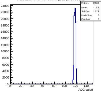
Pedestals mcm81-1816-refV0-g0-s0-p1 ch 36 test1
