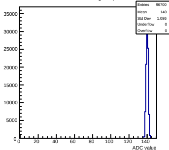
Pedestals mcm81-1816-refV0-g0-s0-p1 ch 94 test1
