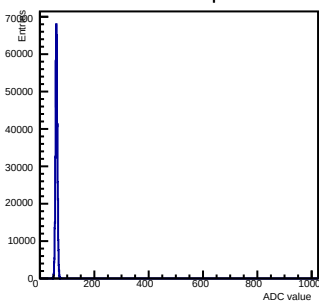
Pedestals ch 0 chip 38 nom
