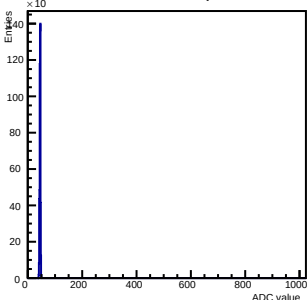
Pedestals ch 15 chip 38 nom
