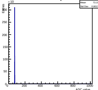
Pedestals ch 6 chip 60 nom
