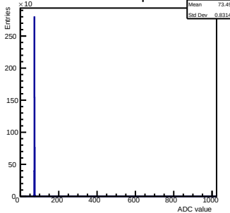
Pedestals ch 2 chip 60 nom
