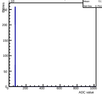
Pedestals ch 10 chip 60 nom
