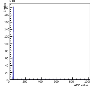
3 Pedestals ch 14 chip 60 nom
