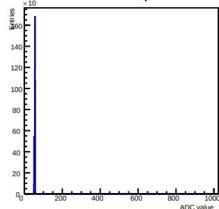
Pedestals ch 4 chip 60 nom
