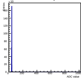
3 Pedestals ch 1 chip 60 nom
