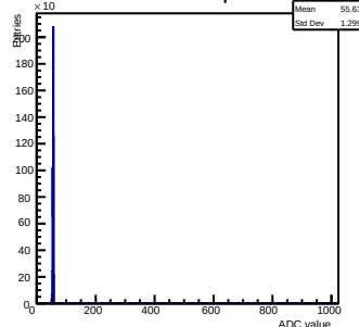
Pedestals ch 6 chip 57 nom
