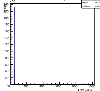
Pedestals ch 14 chip 57 nom
