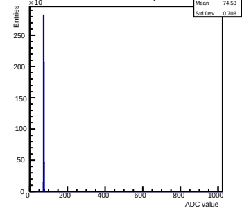
Pedestals ch 11 chip 63 nom
