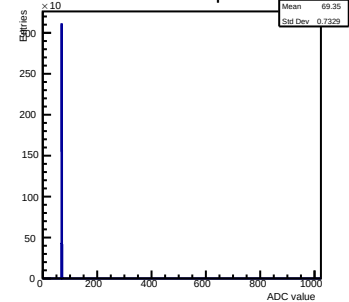
Pedestals ch 3 chip 63 nom
