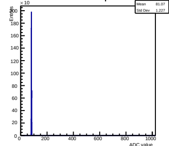
Pedestals ch 7 chip 63 nom
